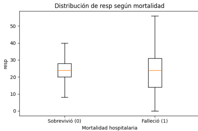
Fig. 4. Distribución de resp según mortalidad hospitalaria.
