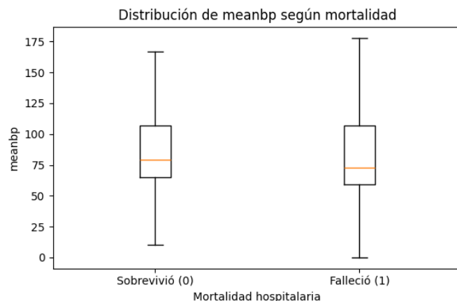
Fig. 2. Distribución de meanbp según mortalidad hospitalaria.
