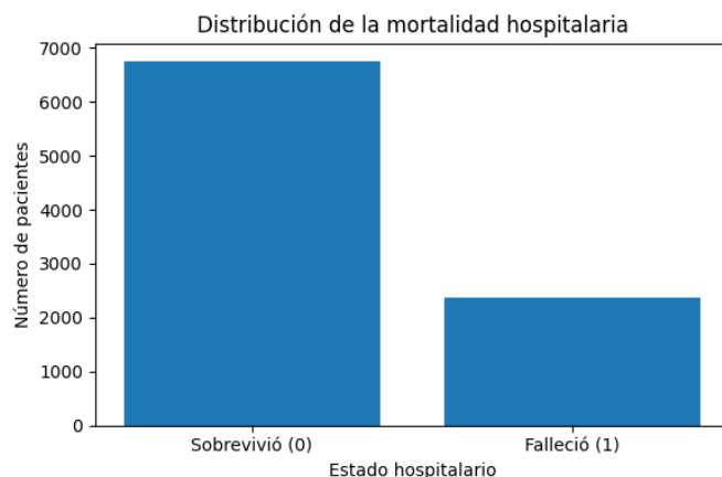
Fig. 1. Distribución de la mortalidad hospitalaria.
