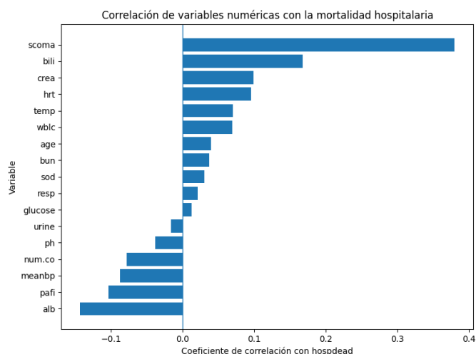
Fig. 8. Correlación de variables numéricas con la mortalidad hospitalaria.
