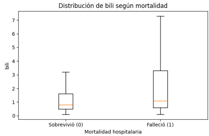
Fig. 6. Distribución de bili según mortalidad hospitalaria.
