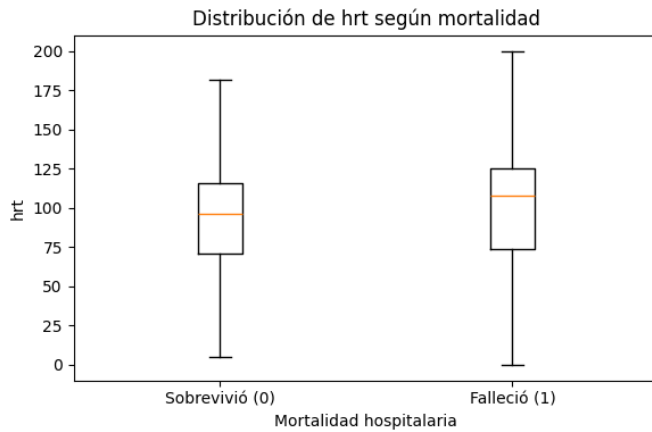
Fig. 3. Distribución de hrt según mortalidad hospitalaria.
