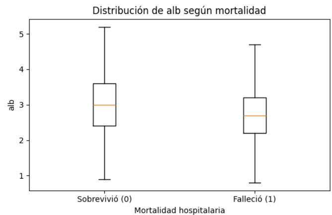
Fig. 7. Distribución de alb según mortalidad hospitalaria.
