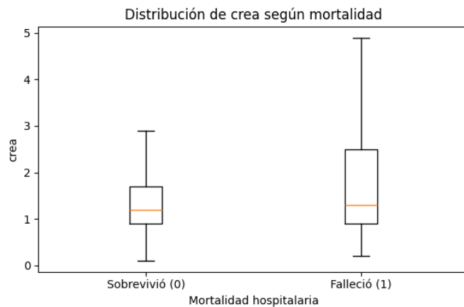
Fig. 5. Distribución de crea según mortalidad hospitalaria.
