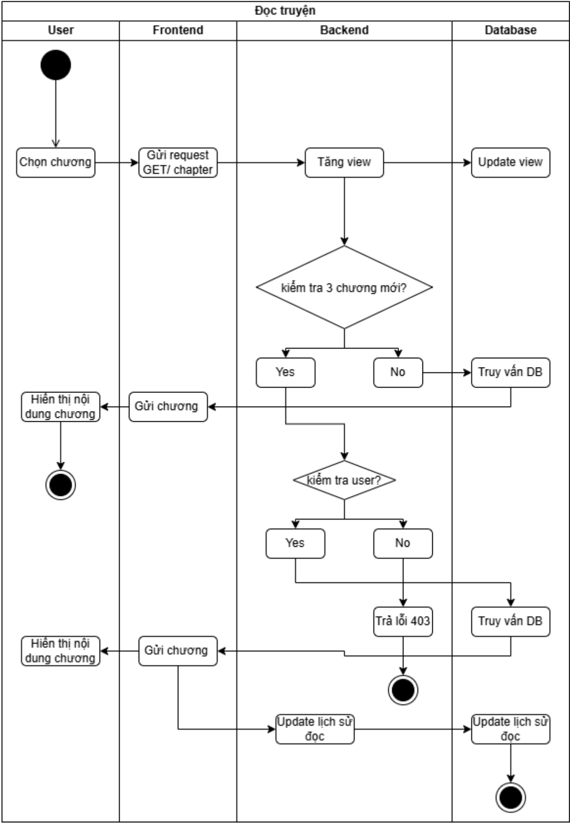
Hình 3-9 Sơ đồ hoạt động đọc truyện
