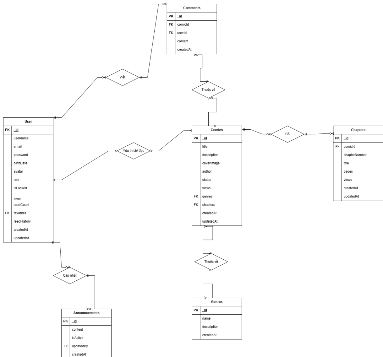
Hình 3-2 Sơ đồ dữ liệu mức luận lý
