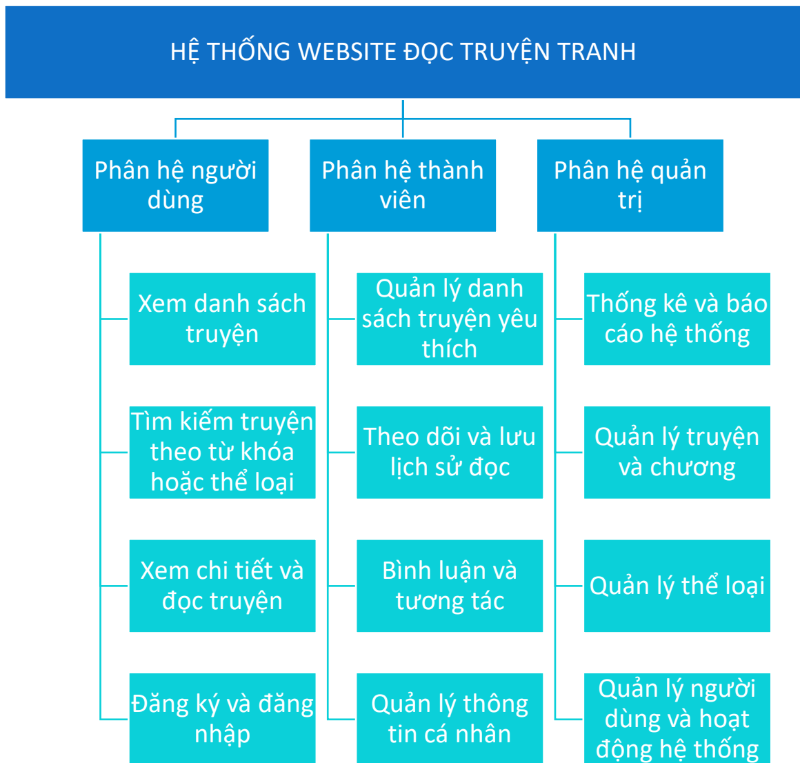
Hình 2-26 Sơ đồ chức năng
