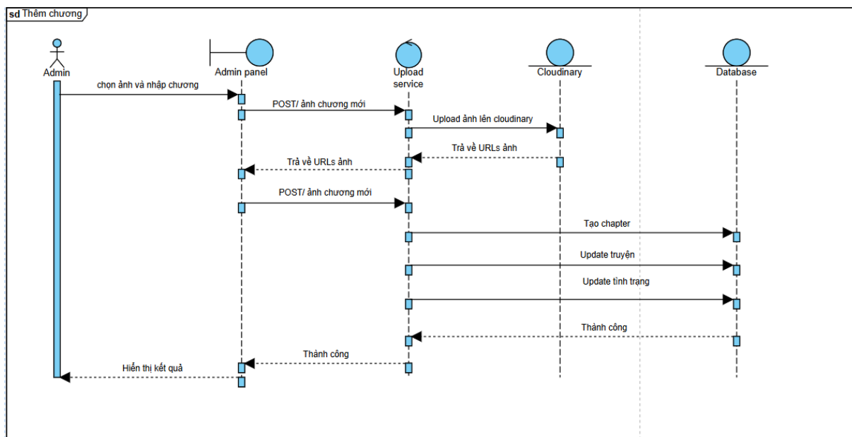
Hình 3-7 Sơ đồ tuần tự thêm chương
