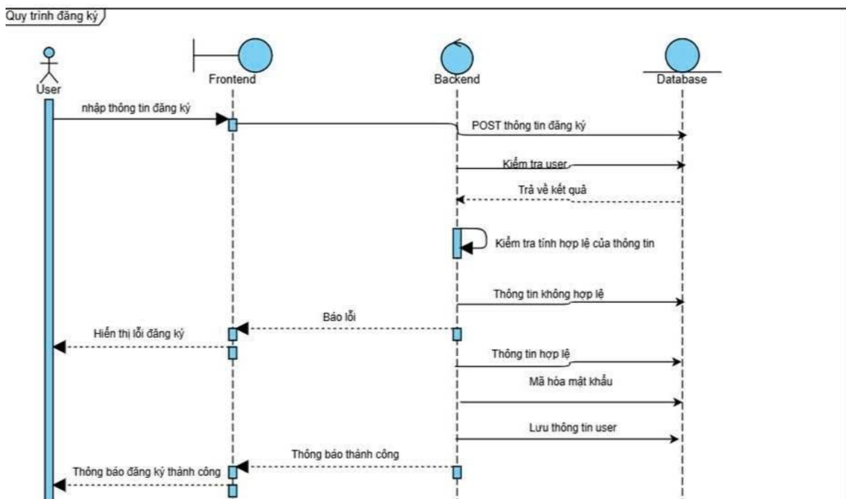
Hình 2-16 Quy trình đăng ký 1
