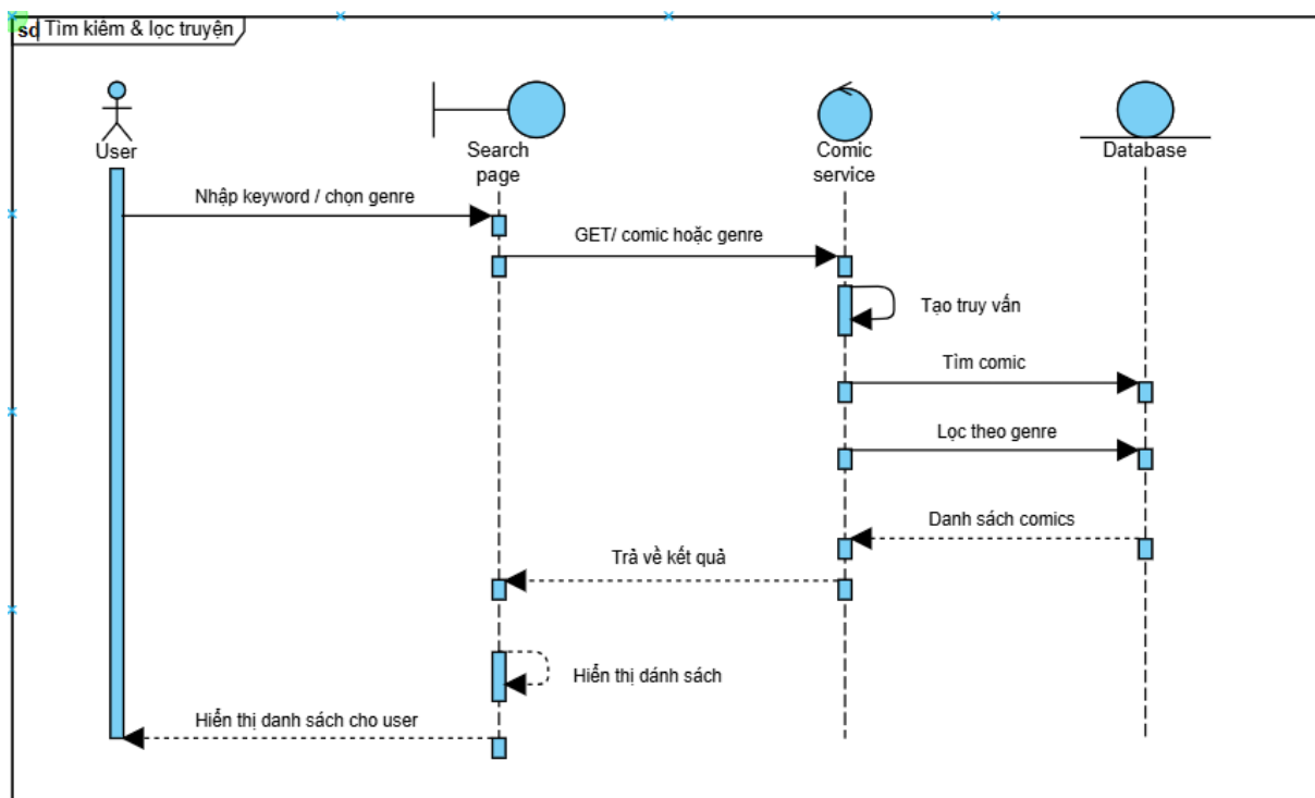
Hình 3-8 Sơ đồ tuần tự tìm kiếm và lọc
