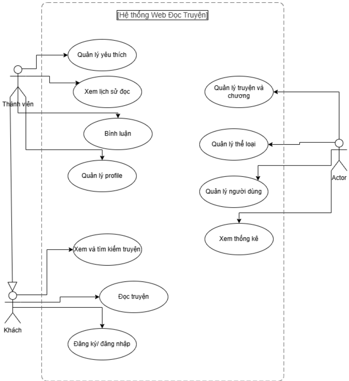
Hình 2-27 Sơ đồ use case tổng quát
