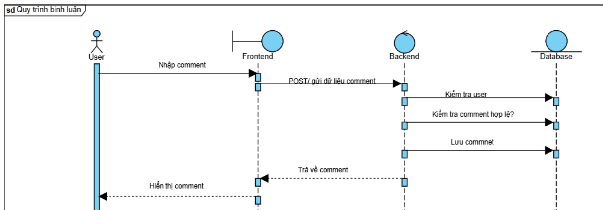
Hình 2-19 Quy trình bình luận 1
