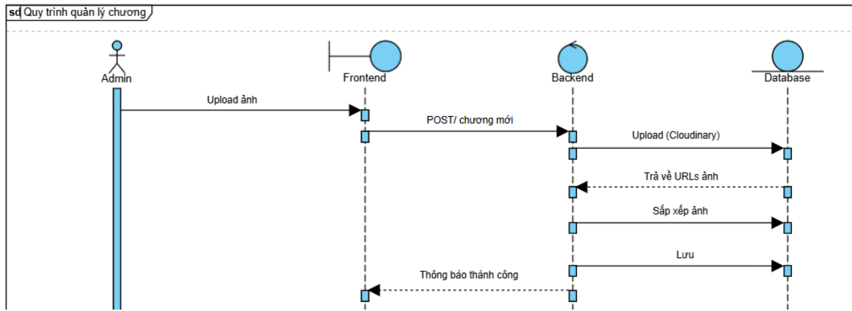
Hình 2-22 Quy trình quản lý chương 1
