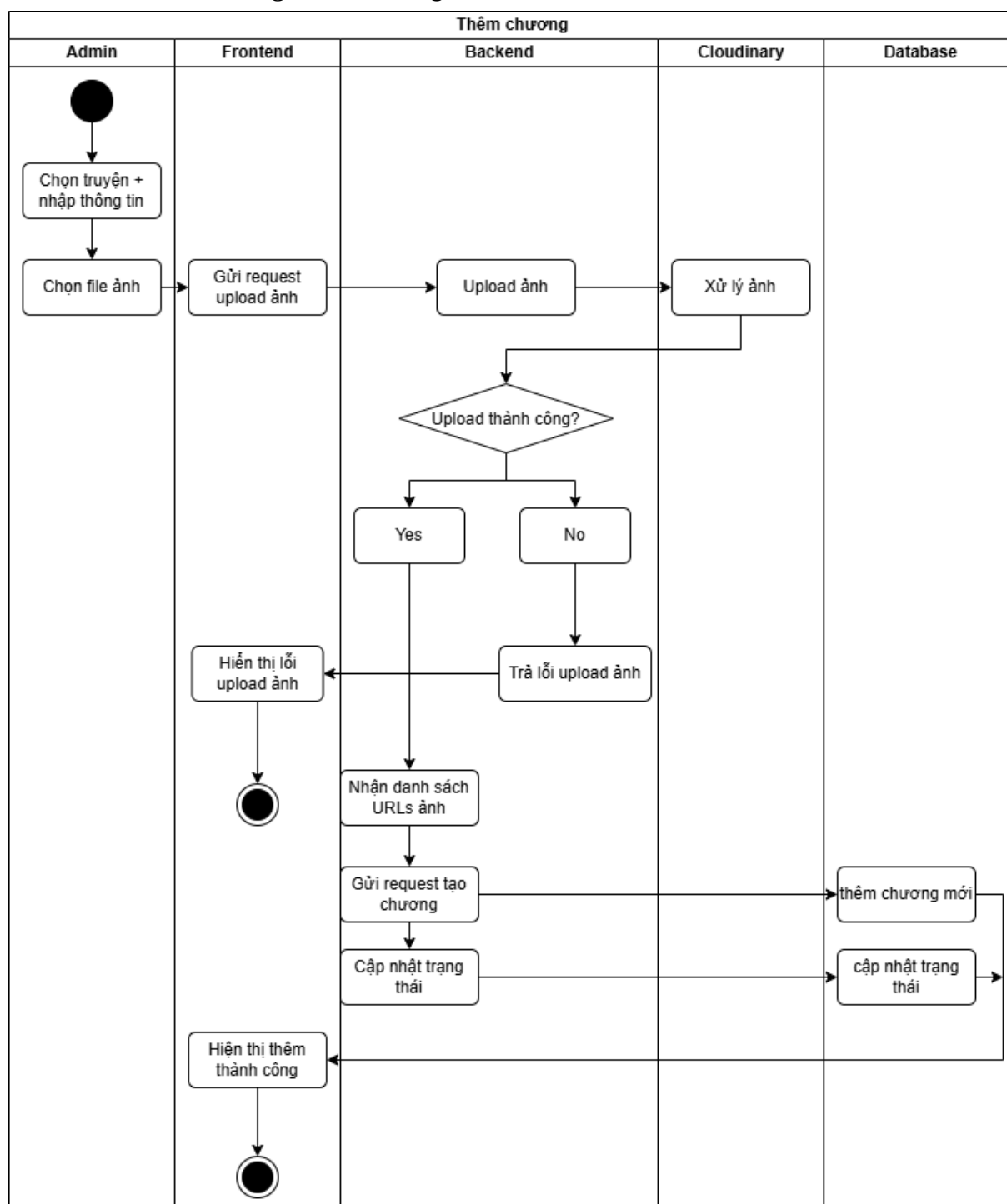
Hình 3-11 Sơ đồ hoạt động thêm chương
