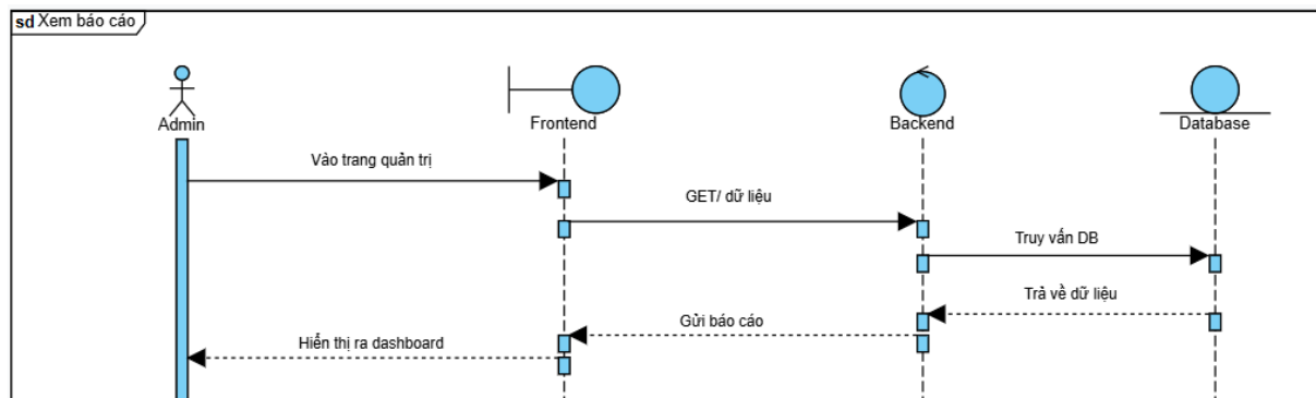
Hình 2-25 Xem báo cáo 1
