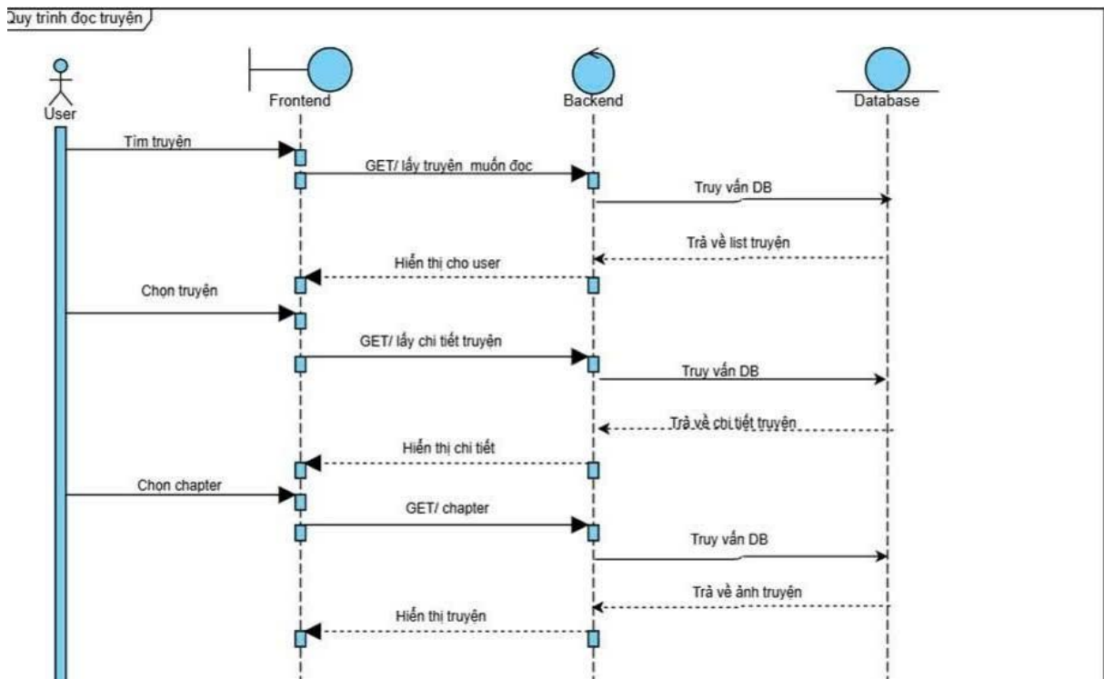
Hình 2-17 Quy trình đọc truyện 1
