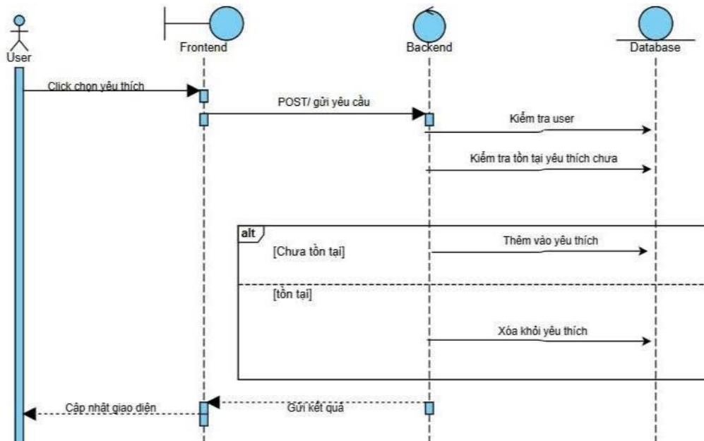
Hình 2-18 Quy trình yêu thích truyện 1
