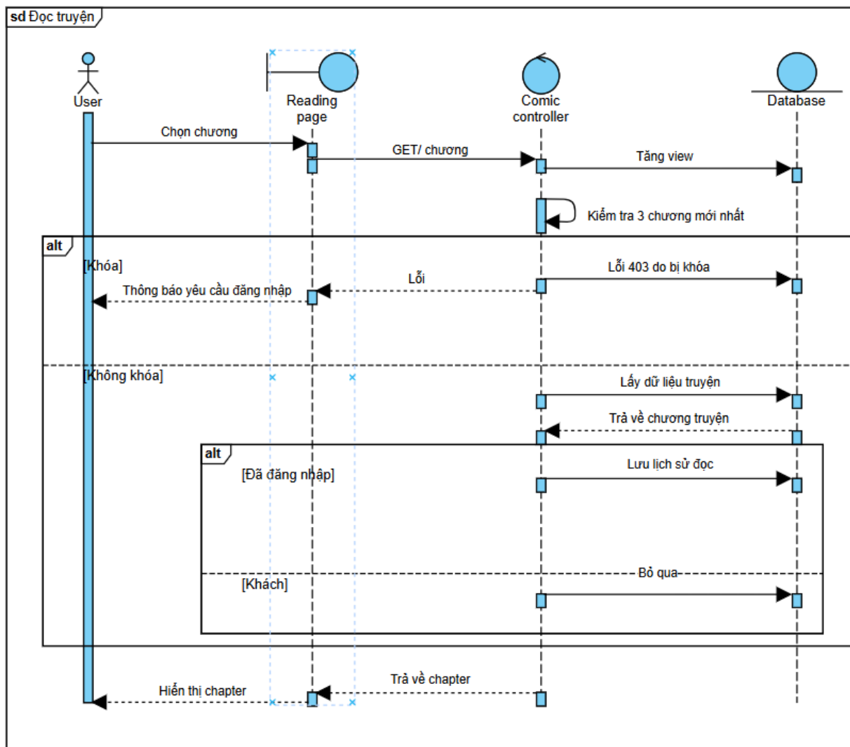
Hình 3-6 Sơ đồ tuần tự đọc truyện
