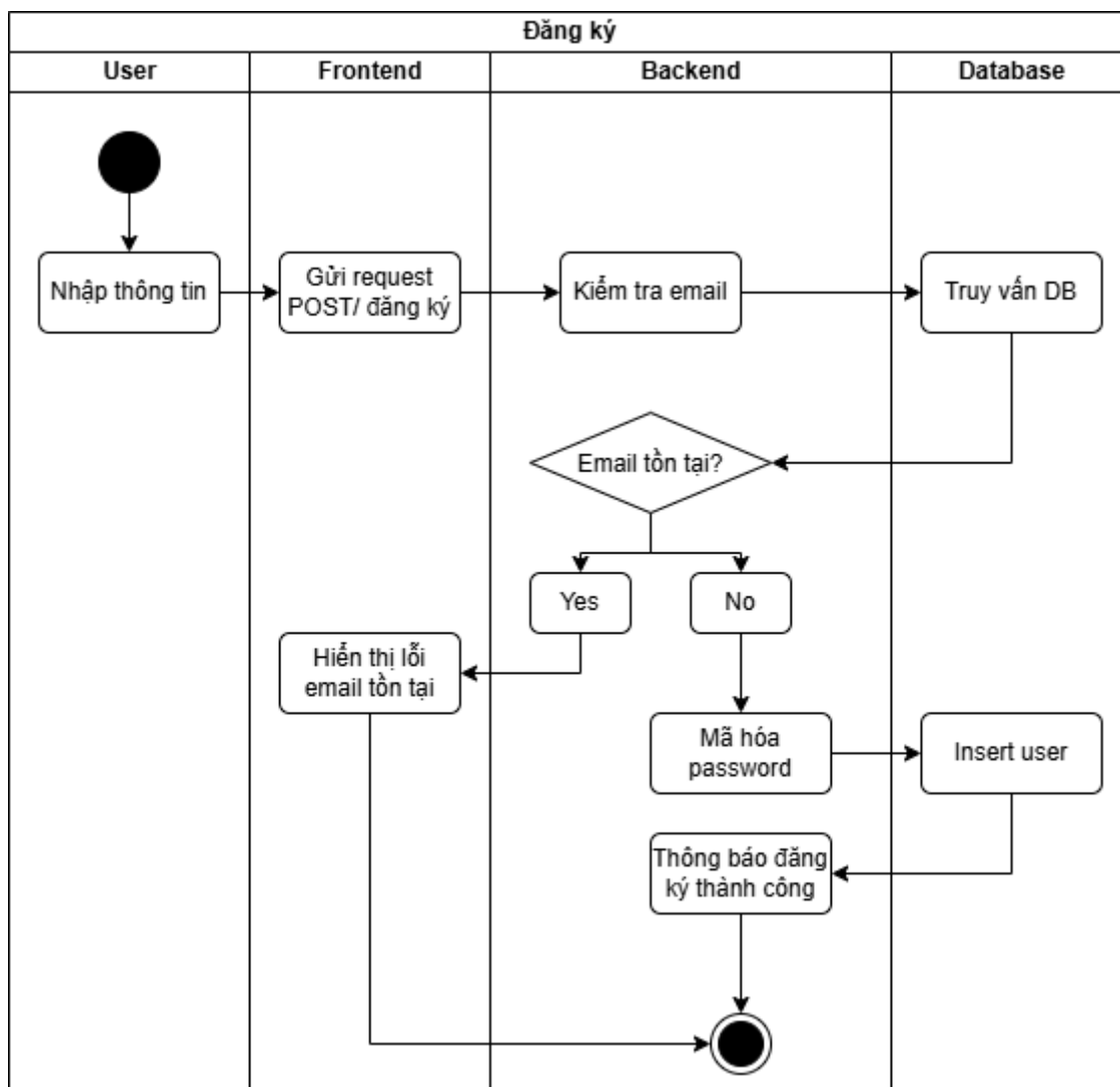
Hình 3-10 Sơ đồ hoạt động đăng ký
