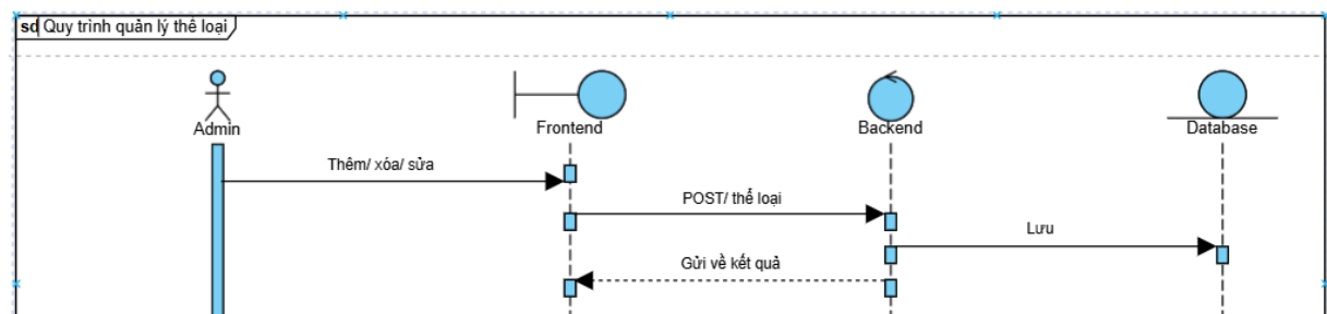
Hình 2-20 Quy trình quản lý thể loại 1
