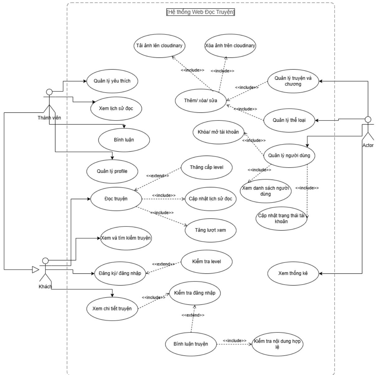
Hình 3-4 Sơ đồ use case chi tiết
