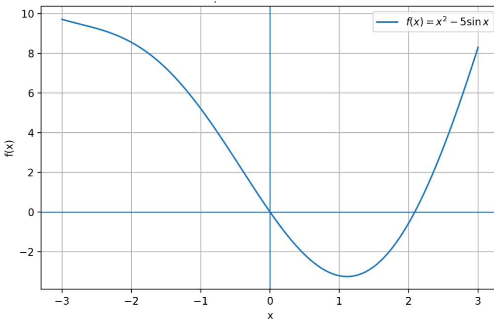
Рис. 1 – График f(x)
