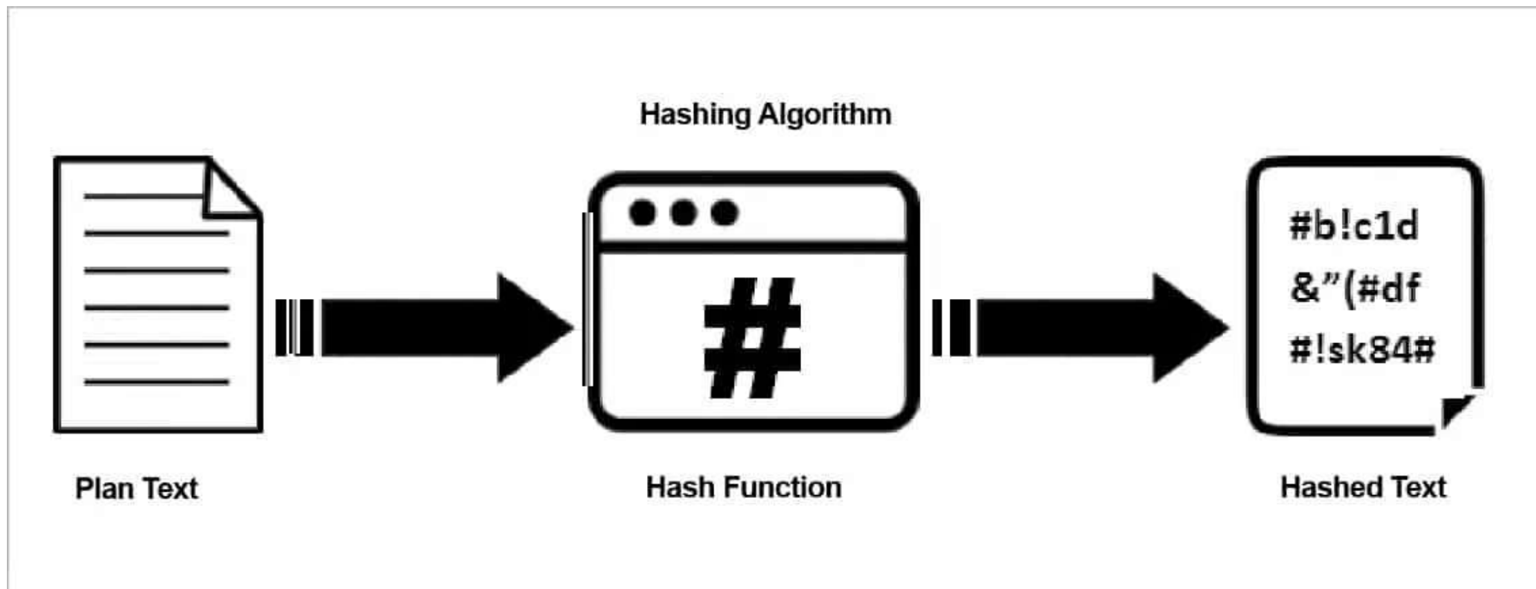
Рис 6. “Хеширование”
