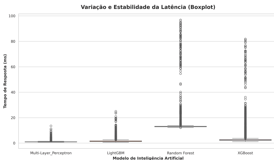
Figura 5.4: Variação e Estabilidade da Latência (Boxplot).
