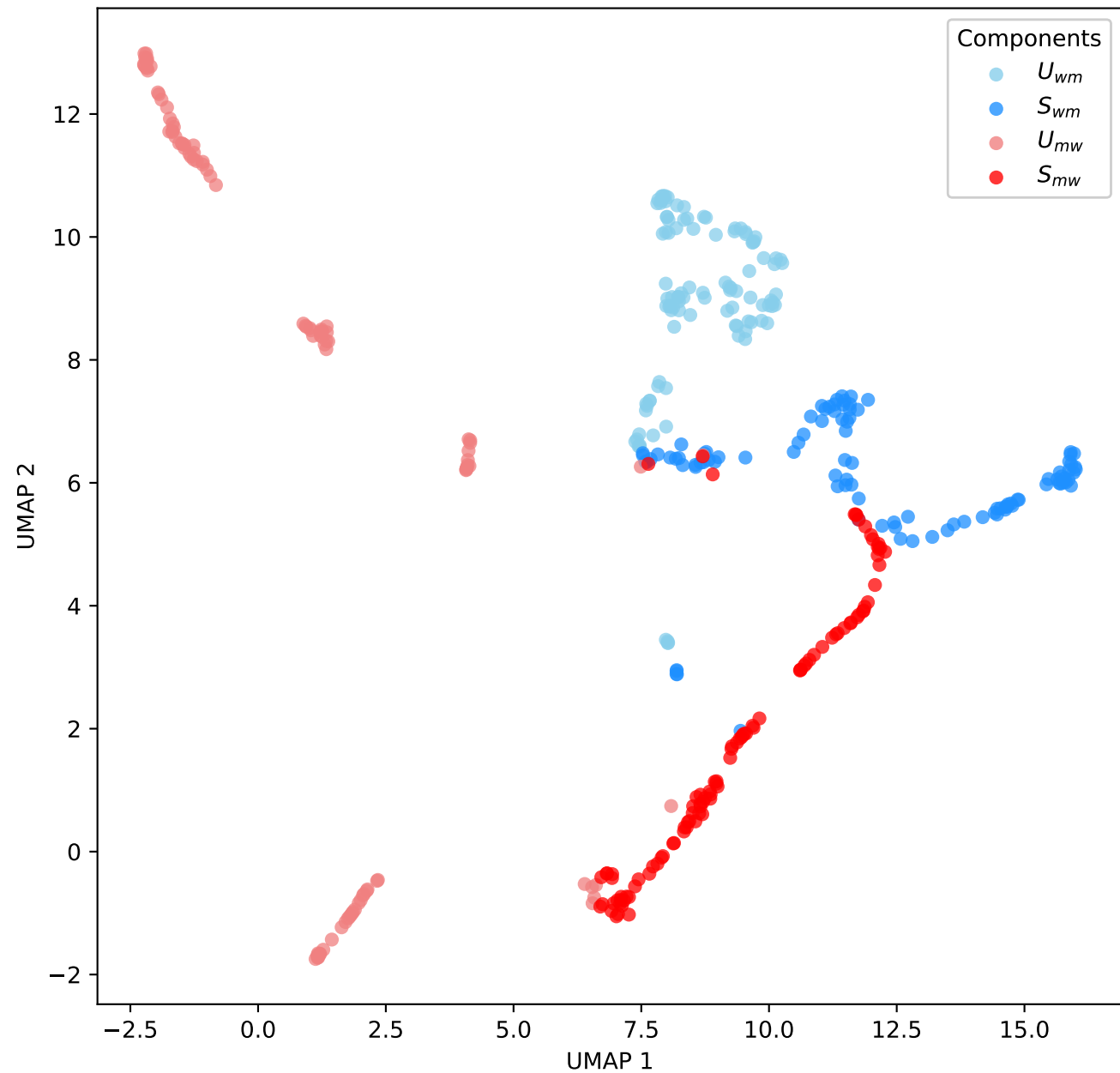
TCGA-LGG: wsi vs mol
