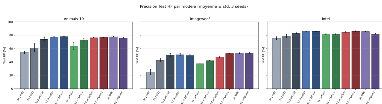
FIGURE 8.1 – Précision Test HF (moyenne \pm écart-type) de tous les modèles, sur les trois datasets.
