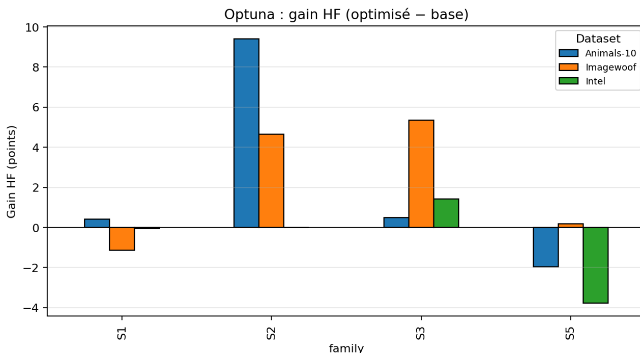
FIGURE 6.1 – Gains de précision Test HF apportés par l’optimisation Optuna (version optimisée – version de base), par stratégie et par dataset.
