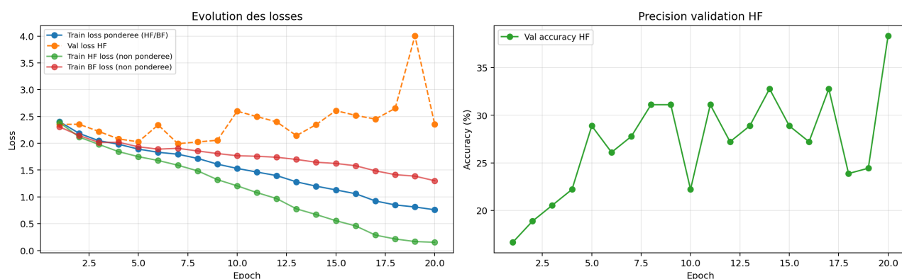
FIGURE 5.4 – Évolution des pertes et de la précision validation HF pour la Stratégie 2 sur Imagewoof .
