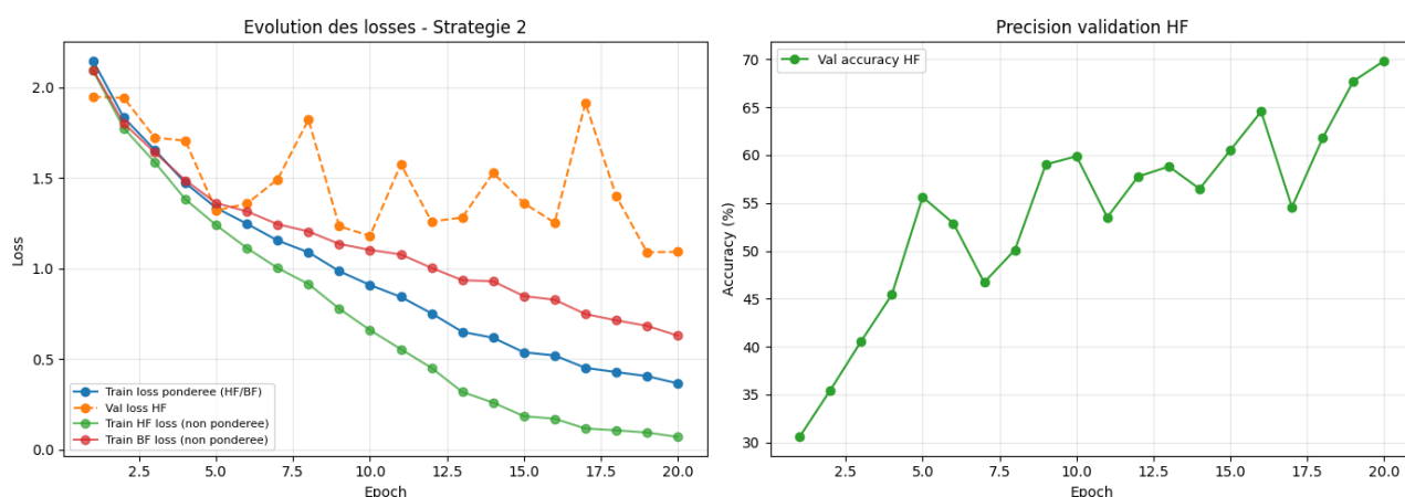
FIGURE 5.3 – Évolution des pertes et de la précision validation HF pour la Stratégie 2 (co-training pondéré HF/BF) sur Animals-10 .
