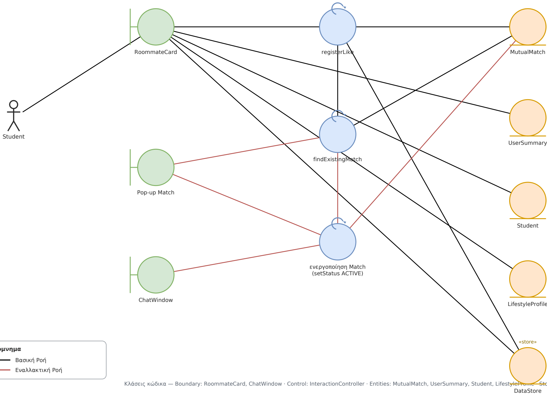
Εικόνα 4: Robustness Diagram — UC04 — Δημιουργία Αμοιβαίου Match
