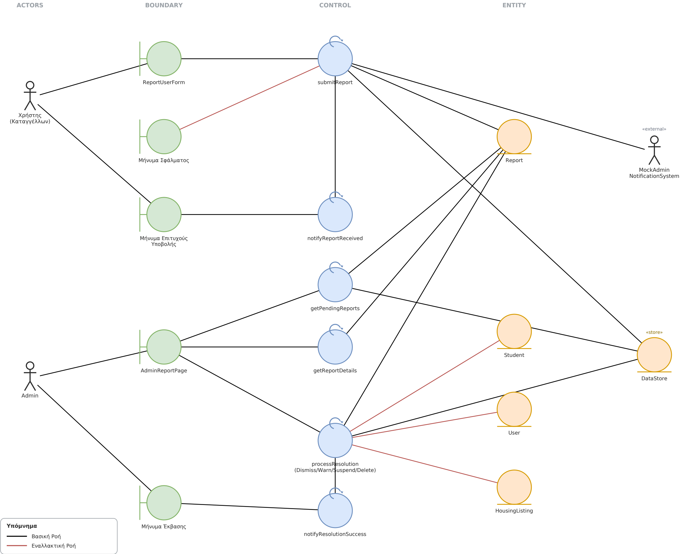
Εικόνα 9: Robustness Diagram — UC09 — Καταγγελία Χρήστη & Διαχείριση από Admin
