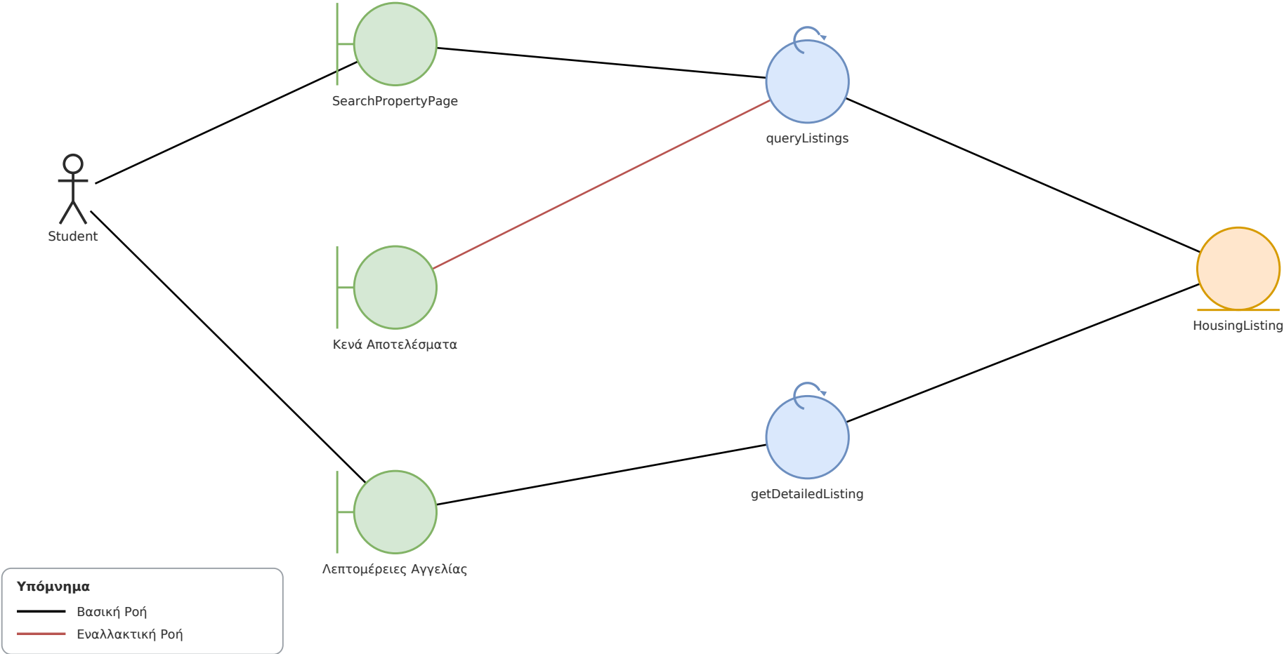
Εικόνα 7: Robustness Diagram — UC07 — Εύρεση & Προβολή Ακινήτου
