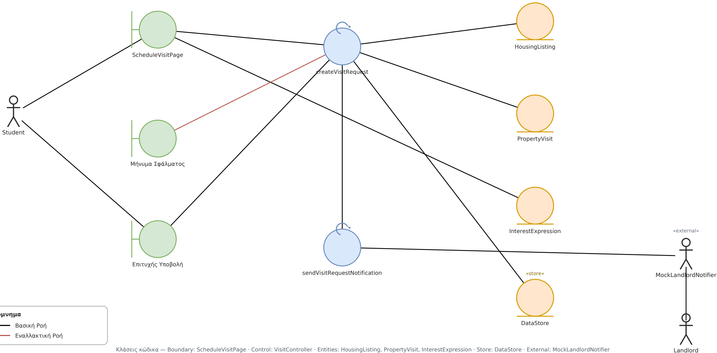
Εικόνα 10: Robustness Diagram — UC10 — Προγραμματισμός Επίσκεψης Ακινήτου
