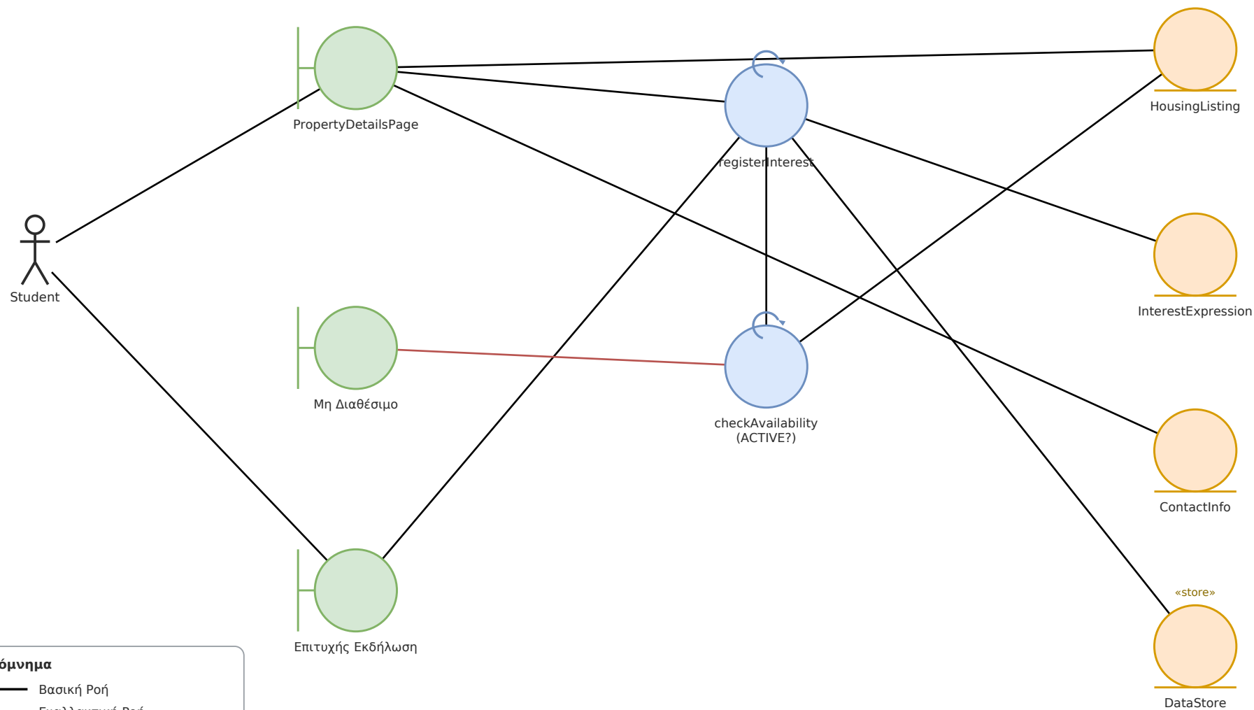
Εικόνα 8: Robustness Diagram — UC08 — Εκδήλωση Ενδιαφέροντος για Ακίνητο
