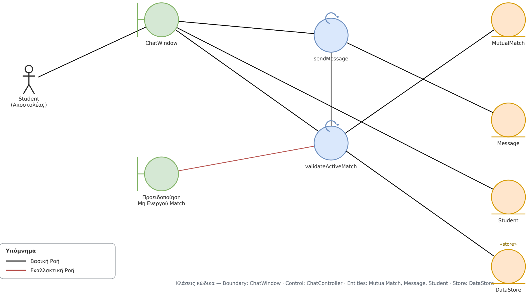
Εικόνα 5: Robustness Diagram — UC05 — Αποστολή & Λήψη Μηνυμάτων
