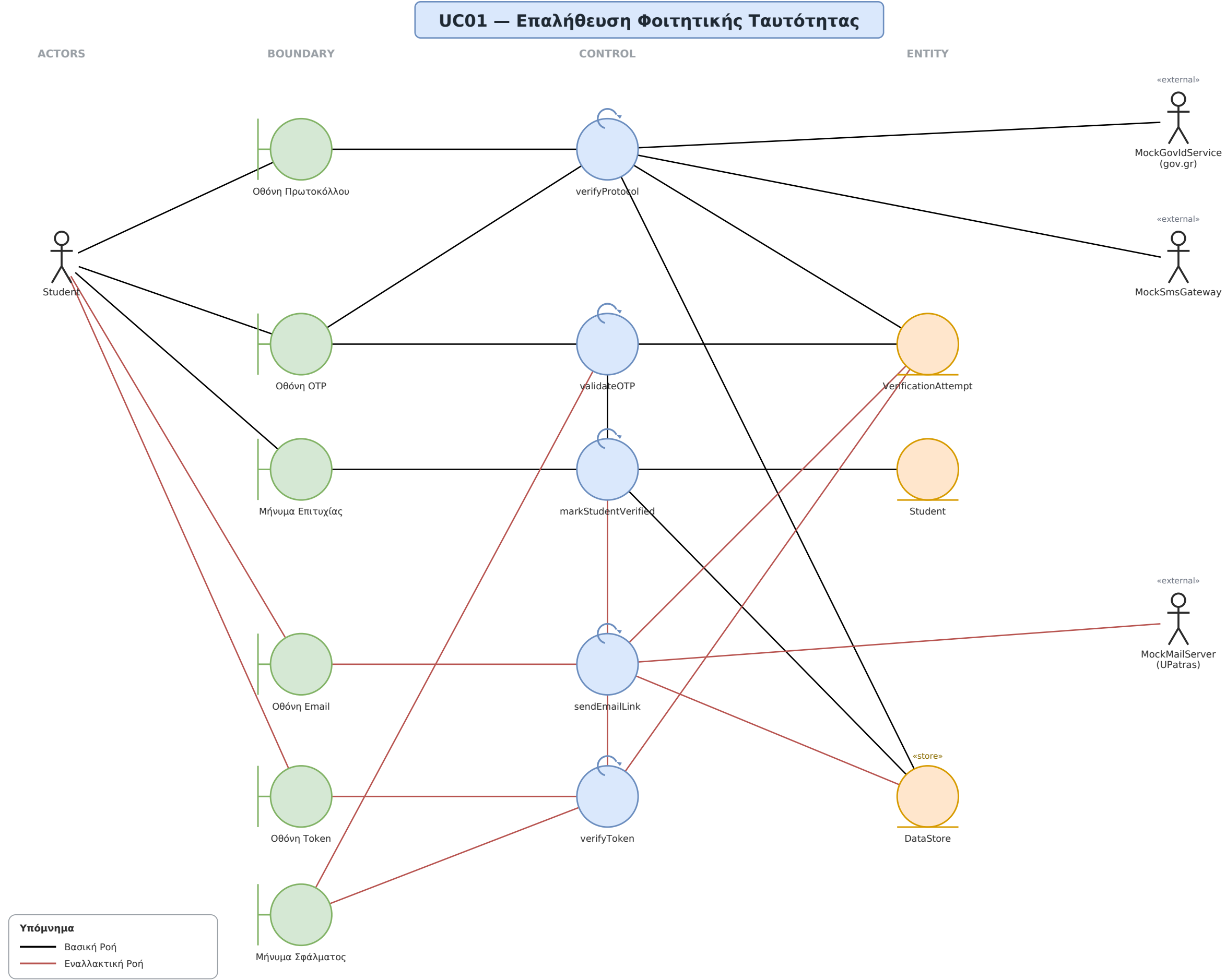
Εικόνα 1: Robustness Diagram — UC01 — Επαλήθευση Φοιτητικής Ταυτότητας
