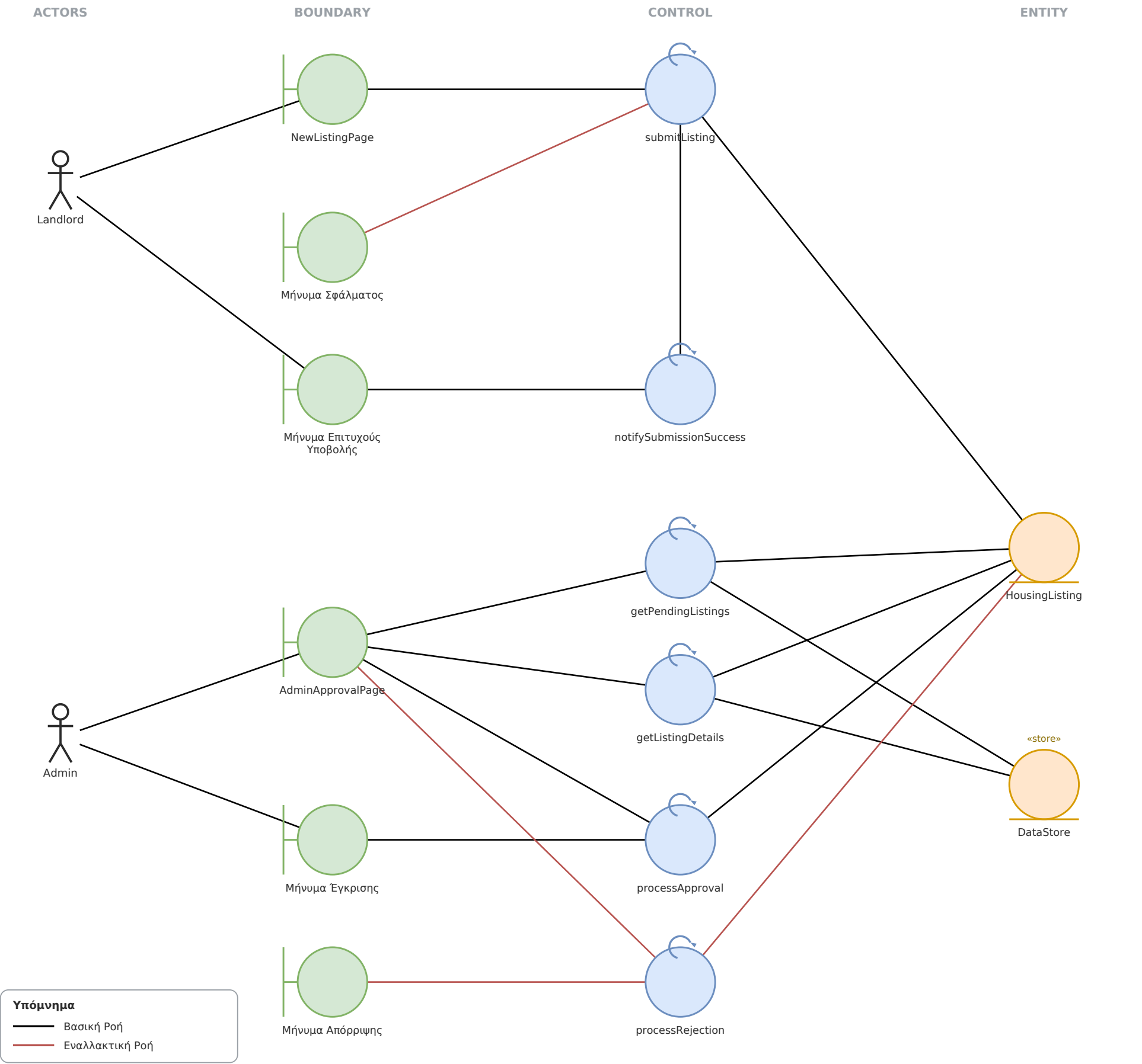
Εικόνα 6: Robustness Diagram — UC06 — Καταχώρηση Αγγελίας & Έγκριση από Admin
