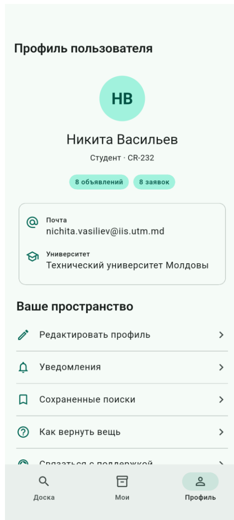
Рисунок 4. Профиль пользователя
