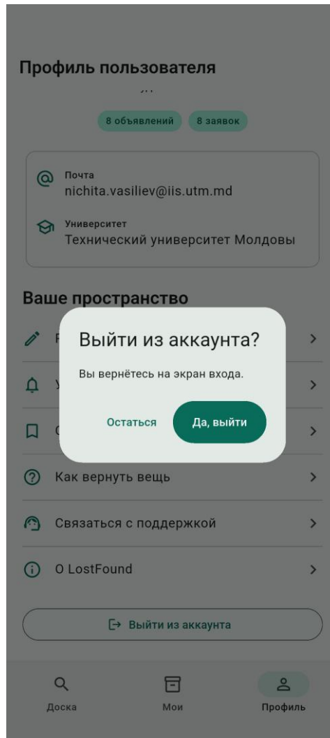
Рисунок 13. Подтверждение выхода
