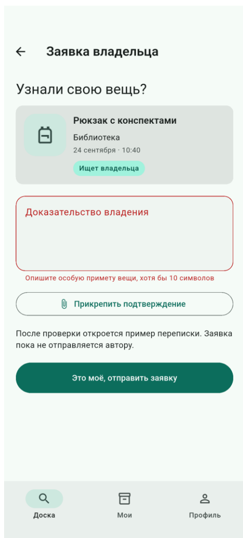
Рисунок 7. Недостаточное доказательство
