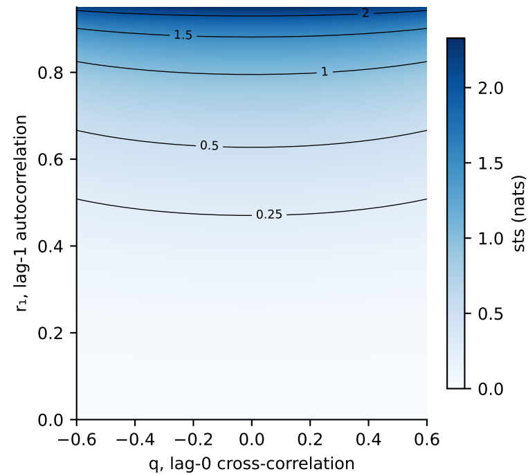
a \text{sts} = -\ln(1 - r_1^2) + \frac{1}{2} \ln(1 - r_1^2 q^2)
