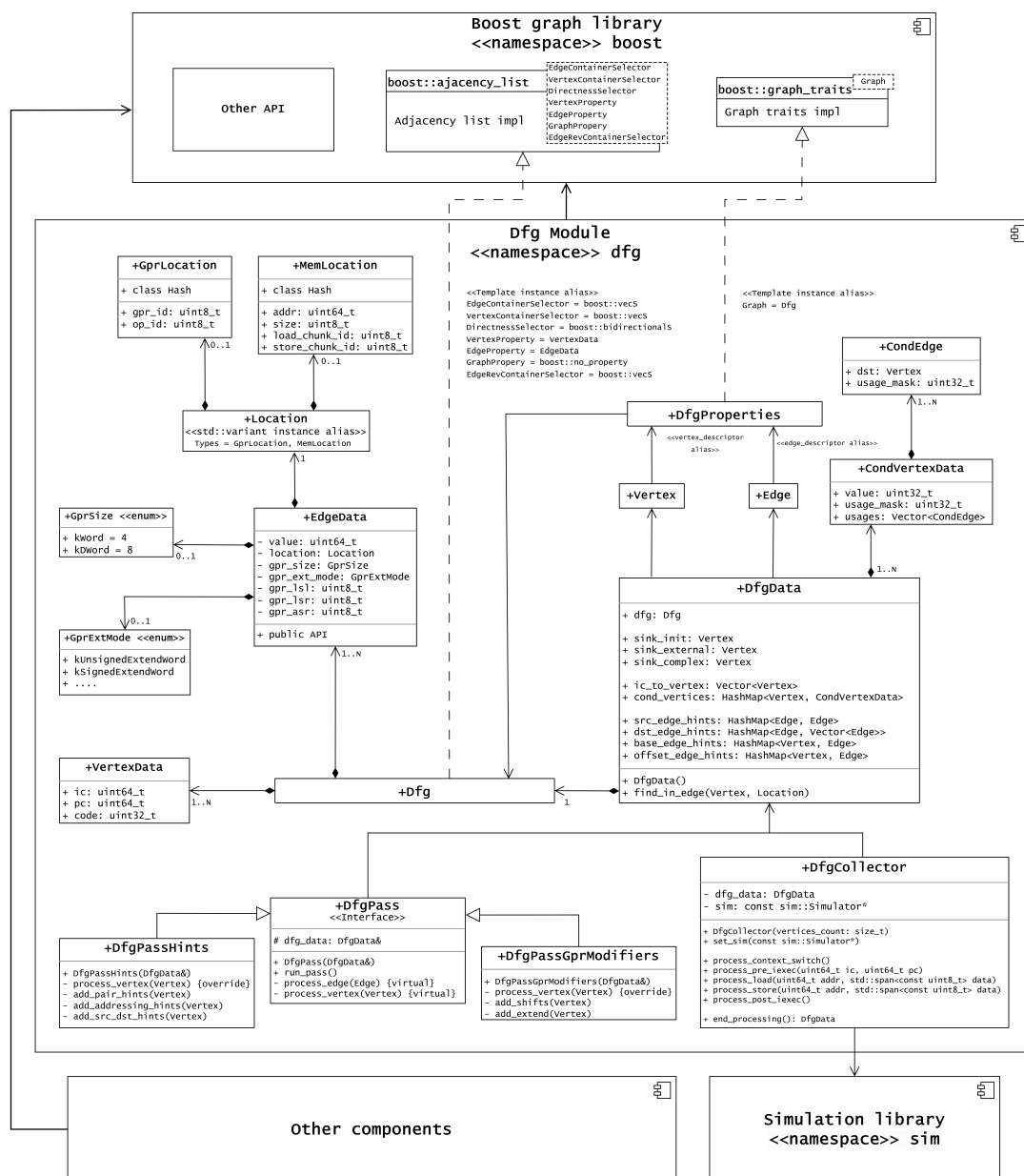
Рис. 11: UML диаграмма модуля ГПД.
