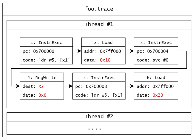
Рис. 2: Пример модифицированной трассы исполнения.
