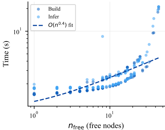
(a) T1 (LU transformer) timing
