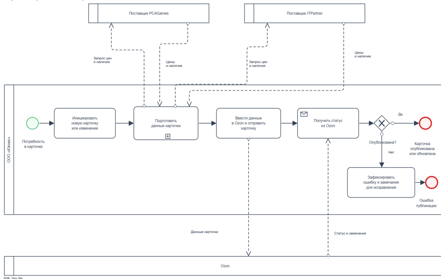
Рисунок 03 — Публикация и внешние участники
