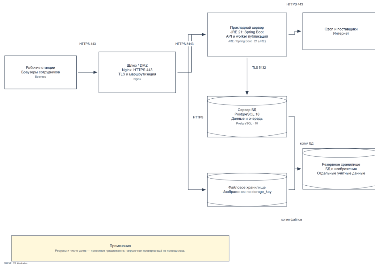
Рисунок 29 – Инфраструктурная схема
