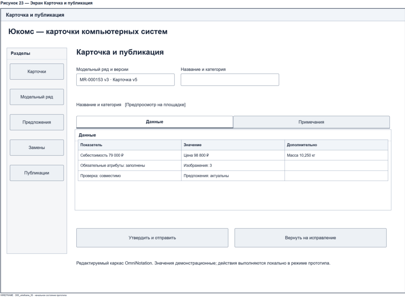
Рисунок 23 – Экран Карточка и публикация
