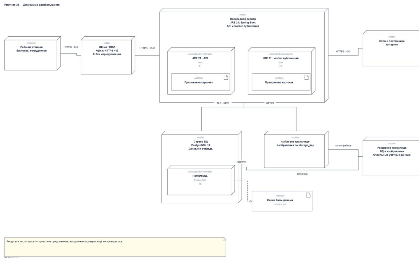
Рисунок 35 – Диаграмма развёртывания
