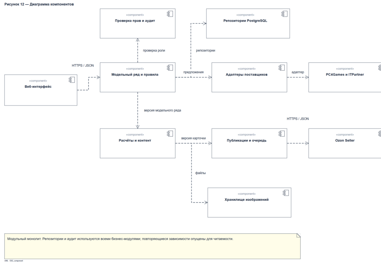
Рисунок 12 – Диаграмма компонентов
