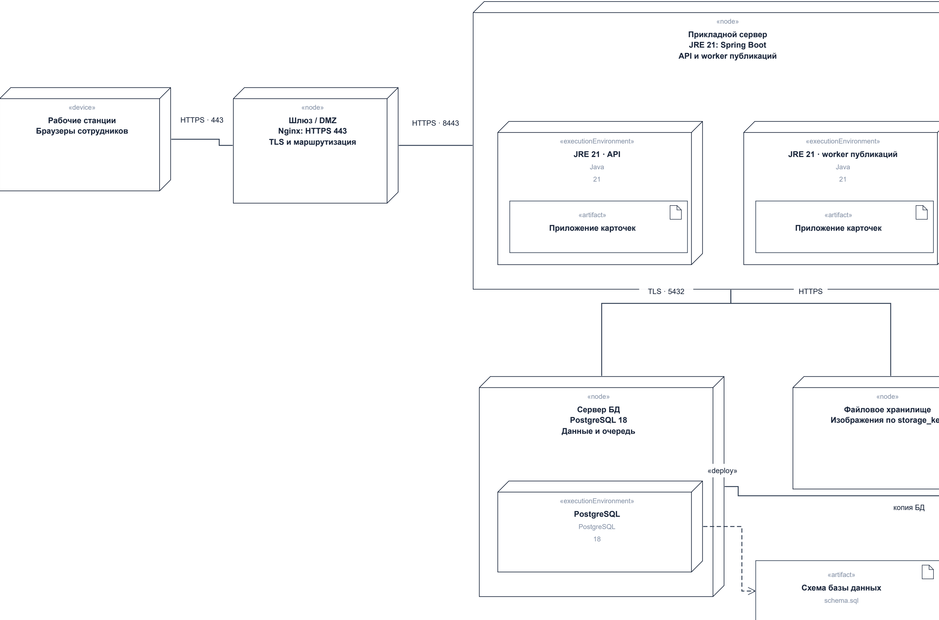
Рисунок 35 — Диаграмма развёртывания · 1/2, 1/2
