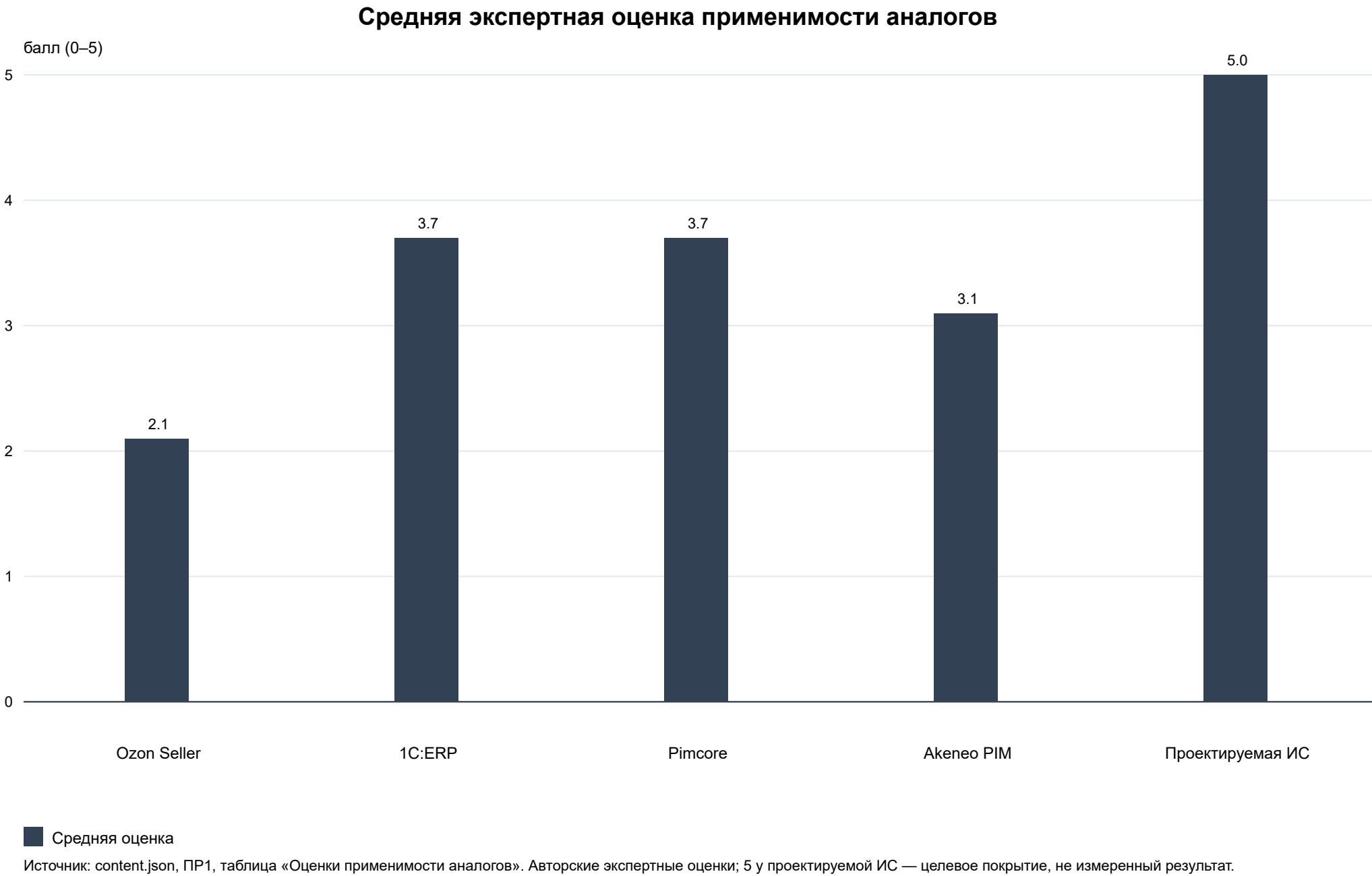
Рисунок 05 — Сравнение аналогов
