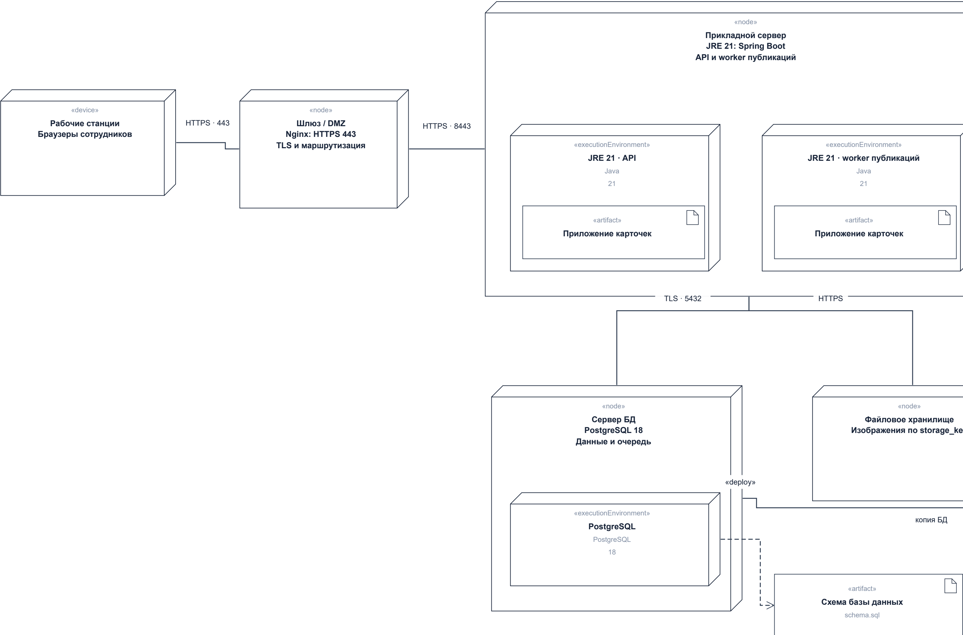
Рисунок 35 — Диаграмма развёртывания · 1/2, 1/2
