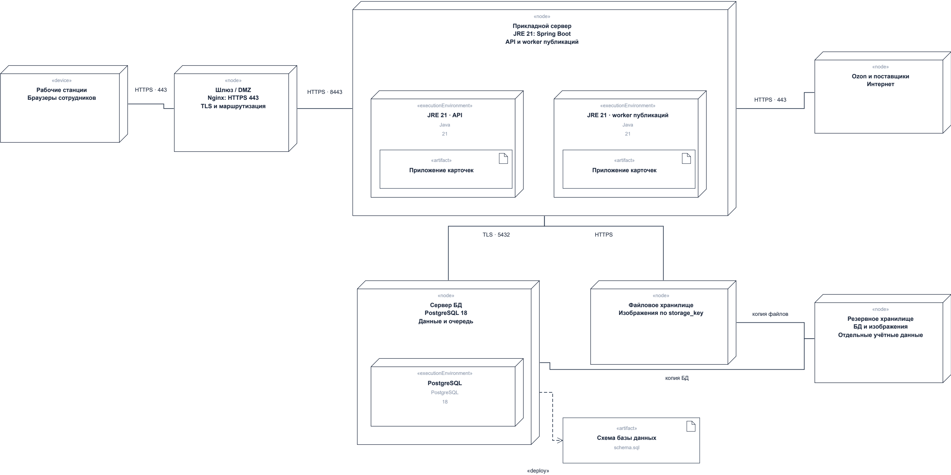
Рисунок 35 — Диаграмма развёртывания
