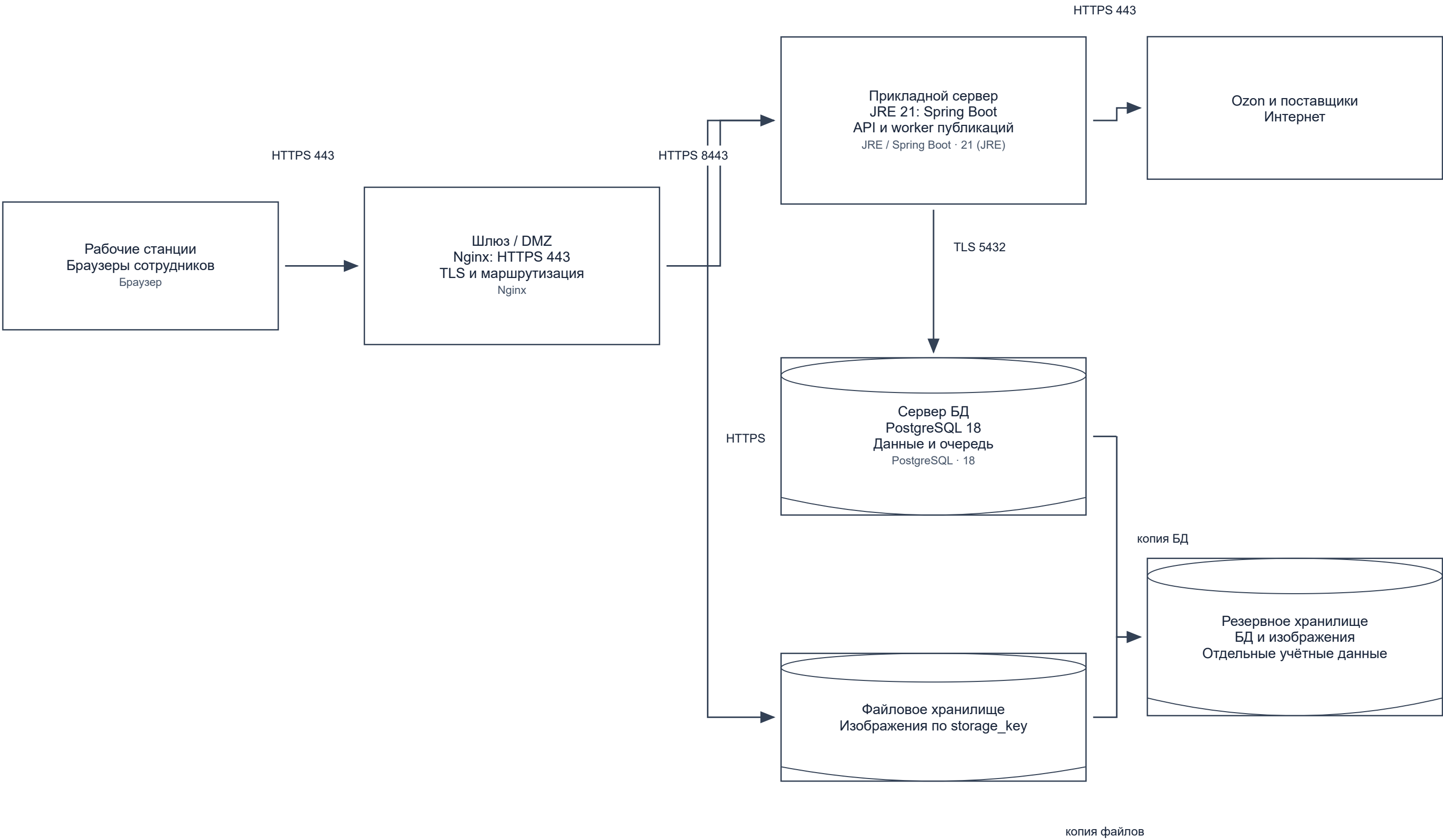
Рисунок 29 — Инфраструктурная схема
