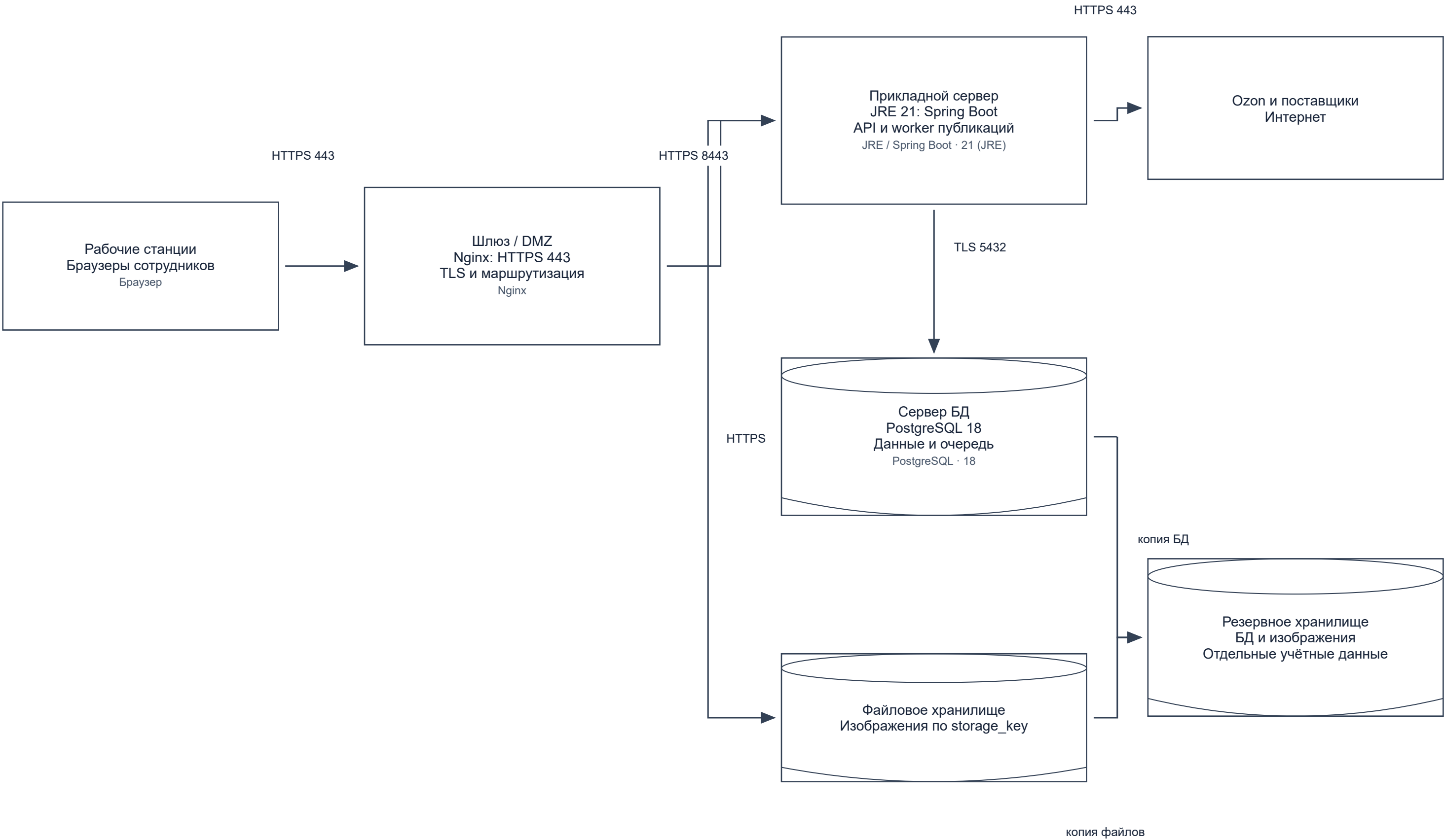
Рисунок 29 — Инфраструктурная схема
