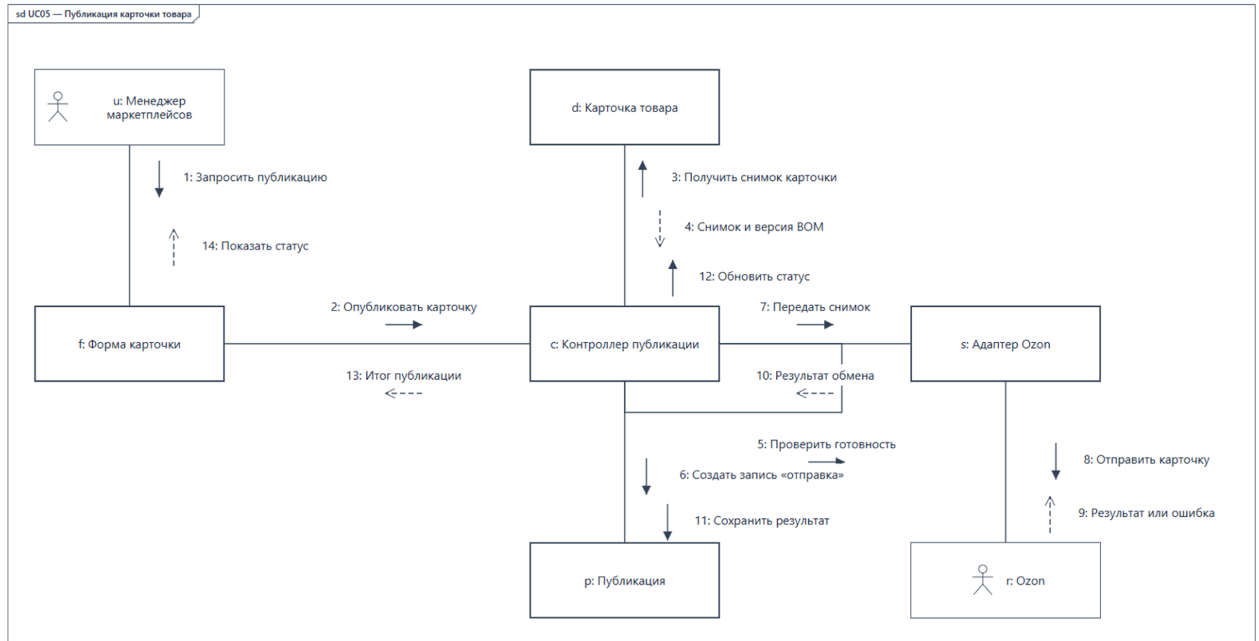
Рисунок 5 – Кооперация объектов при публикации карточки
