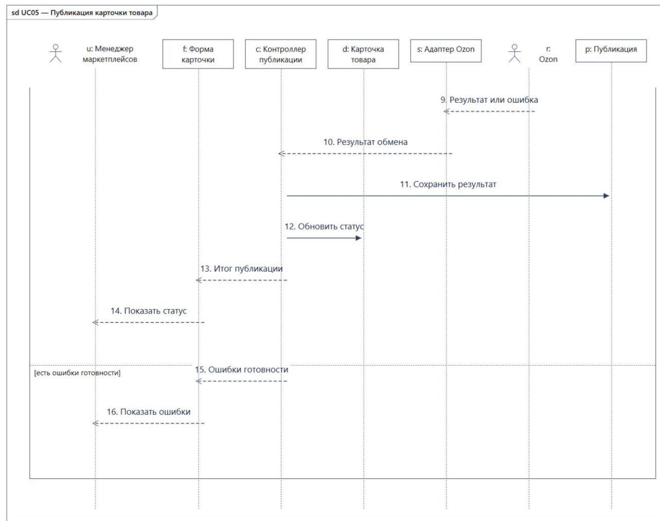
Рисунок 4 – Диаграмма последовательности UC05 (окончание)
