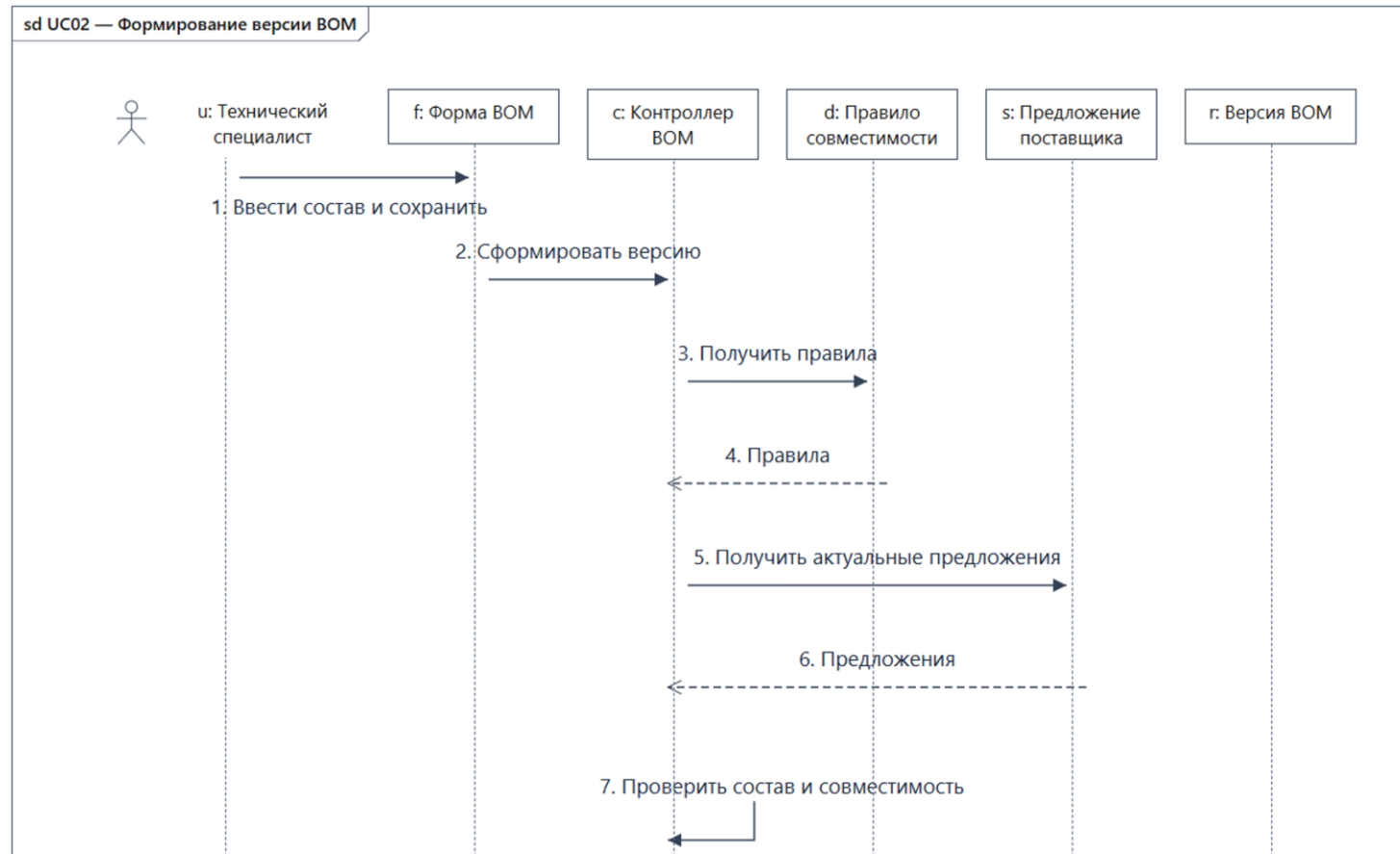
Рисунок 3 – Диаграмма последовательности UC02 (начало)
