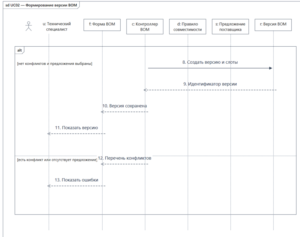
Рисунок 3 – Диаграмма последовательности UC02 (окончание)
