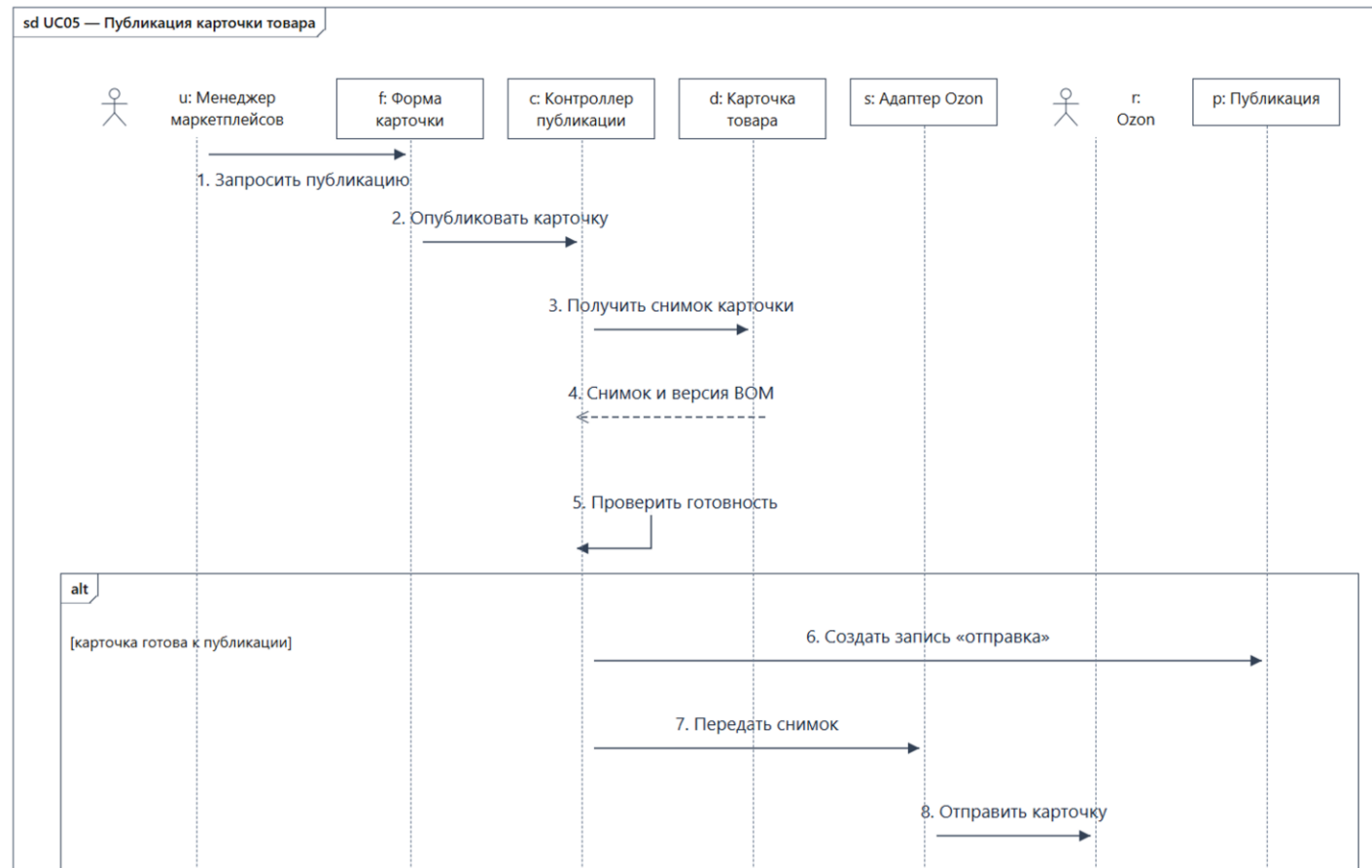
Рисунок 4 – Диаграмма последовательности UC05 (начало)
