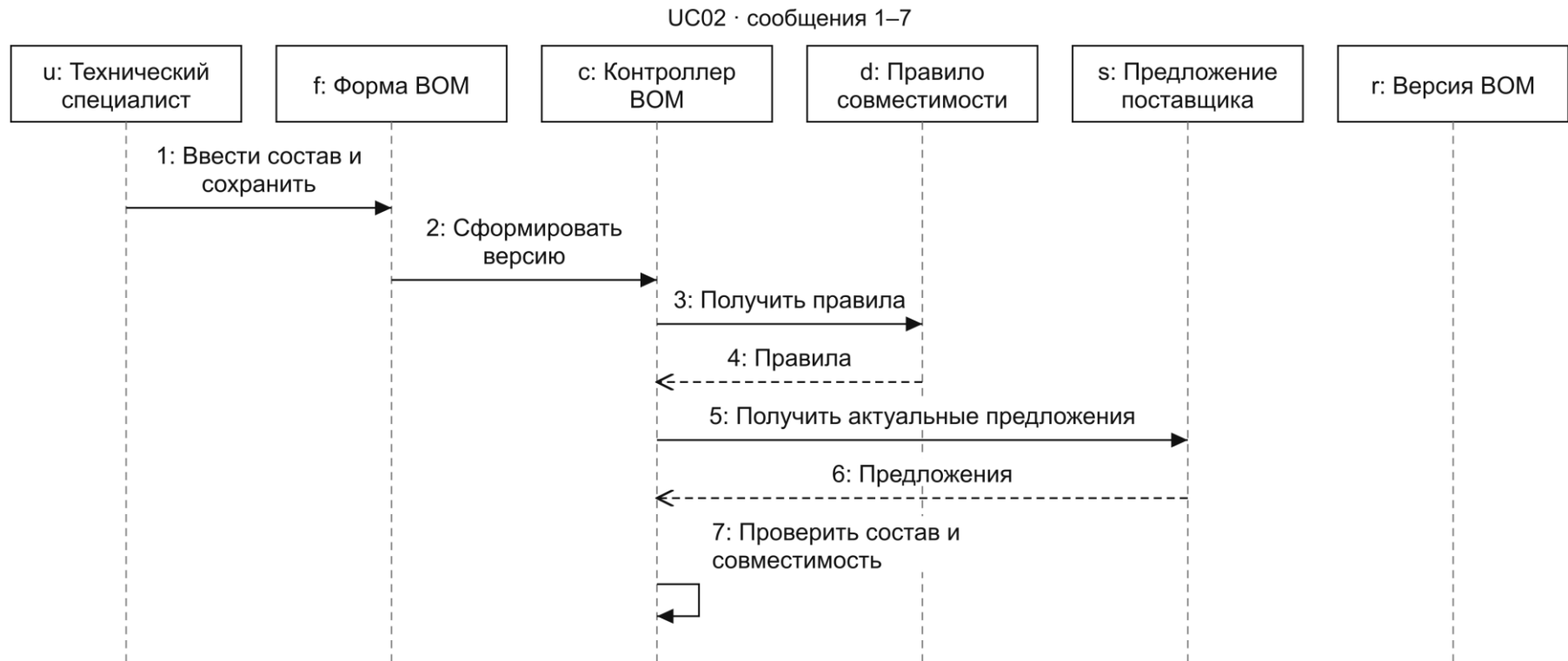
Рисунок 3 – Диаграмма последовательности UC02 (начало)
