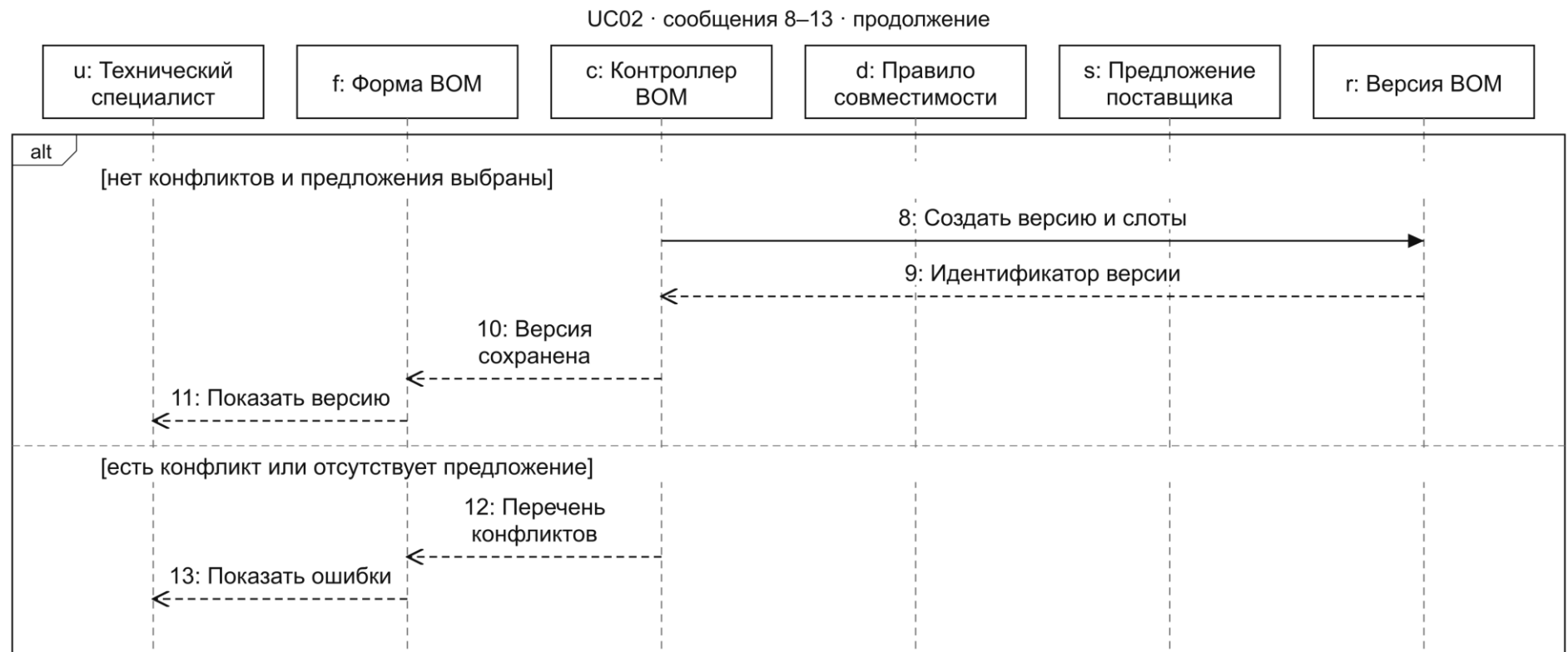
Рисунок 3 – Диаграмма последовательности UC02 (окончание)
