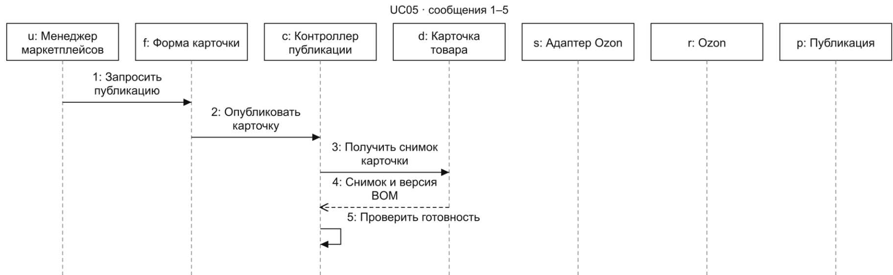
Рисунок 4 – Диаграмма последовательности UC05 (начало)
