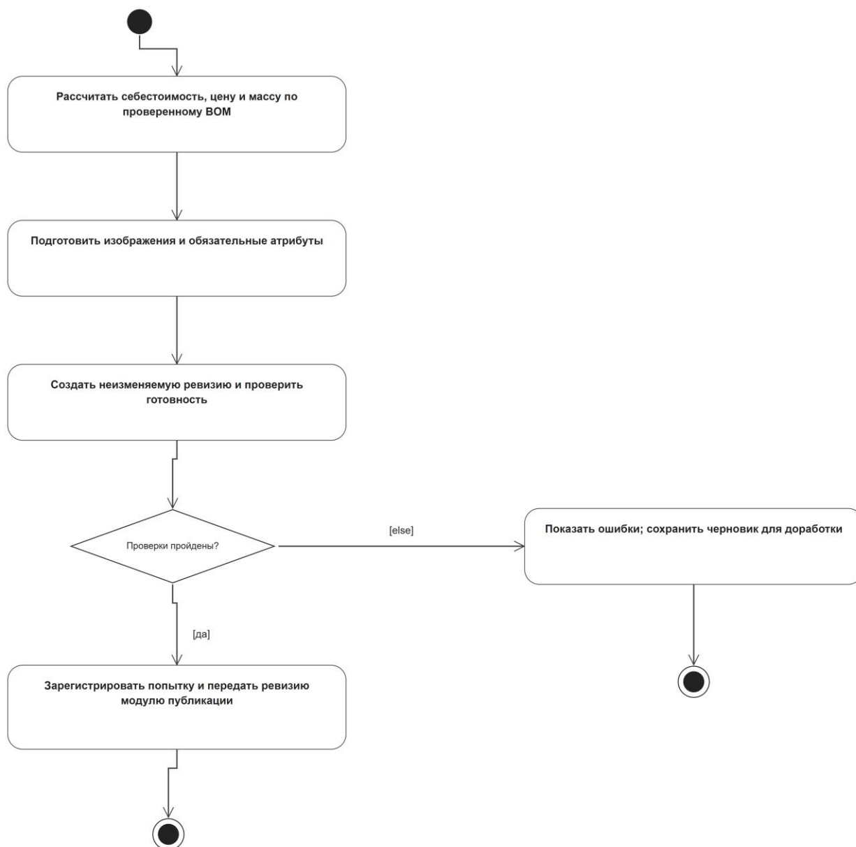
Рисунок 6 – Деятельность: подготовка содержания и передача на публикацию
