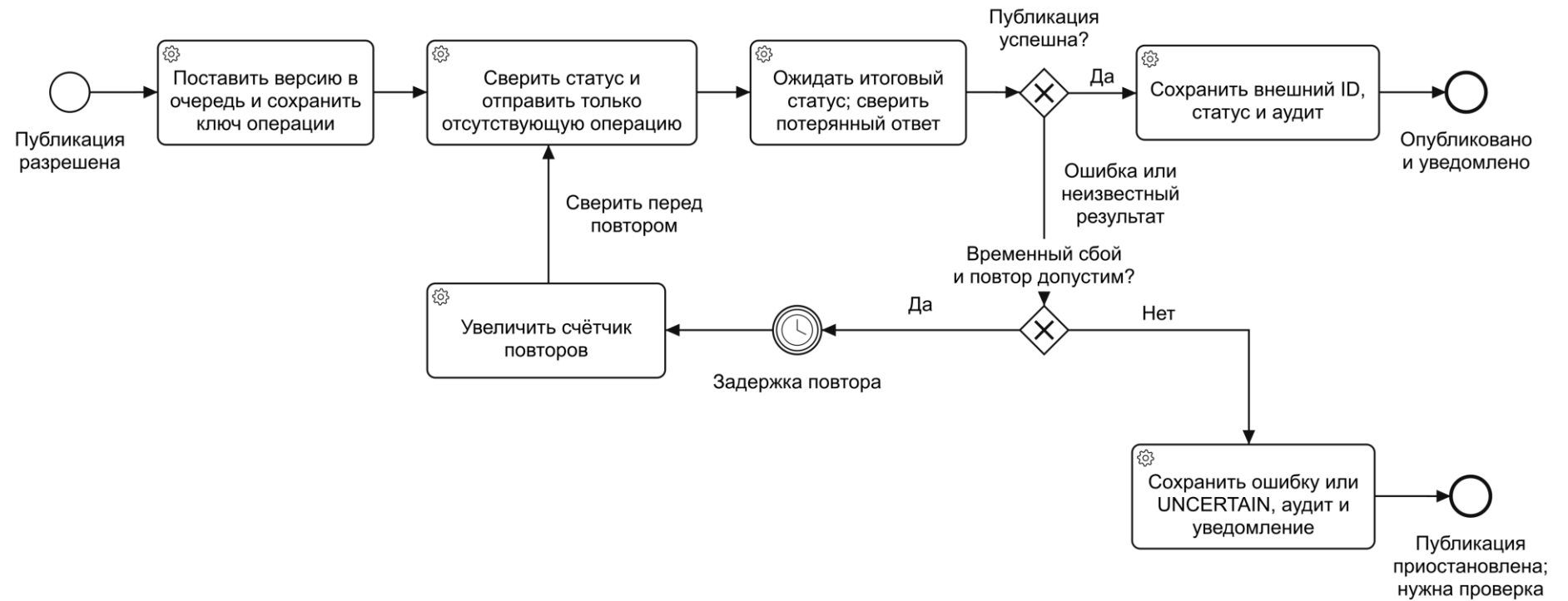
Рисунок 10 – BPMN TO BE: очередь, сверка статуса и обработка результата
