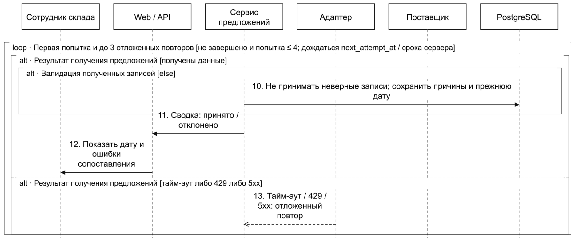
Продолжение рисунка 36 – Последовательность обновления предложений (часть 3 из 4)
