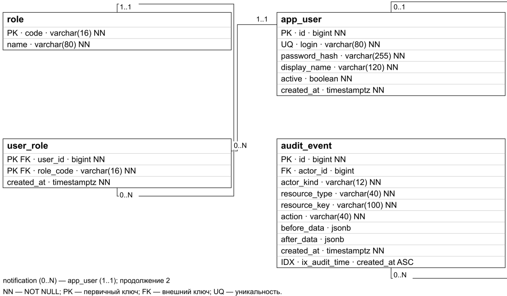
Рисунок 34 – Физическая модель данных, вид 5 (часть 1 из 2)
