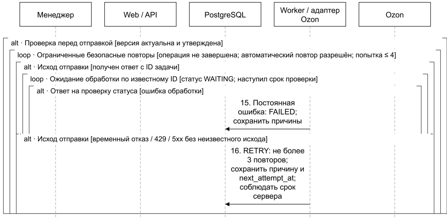
Продолжение рисунка 37 – Последовательность публикации версии карточки (часть 5 из 7)
