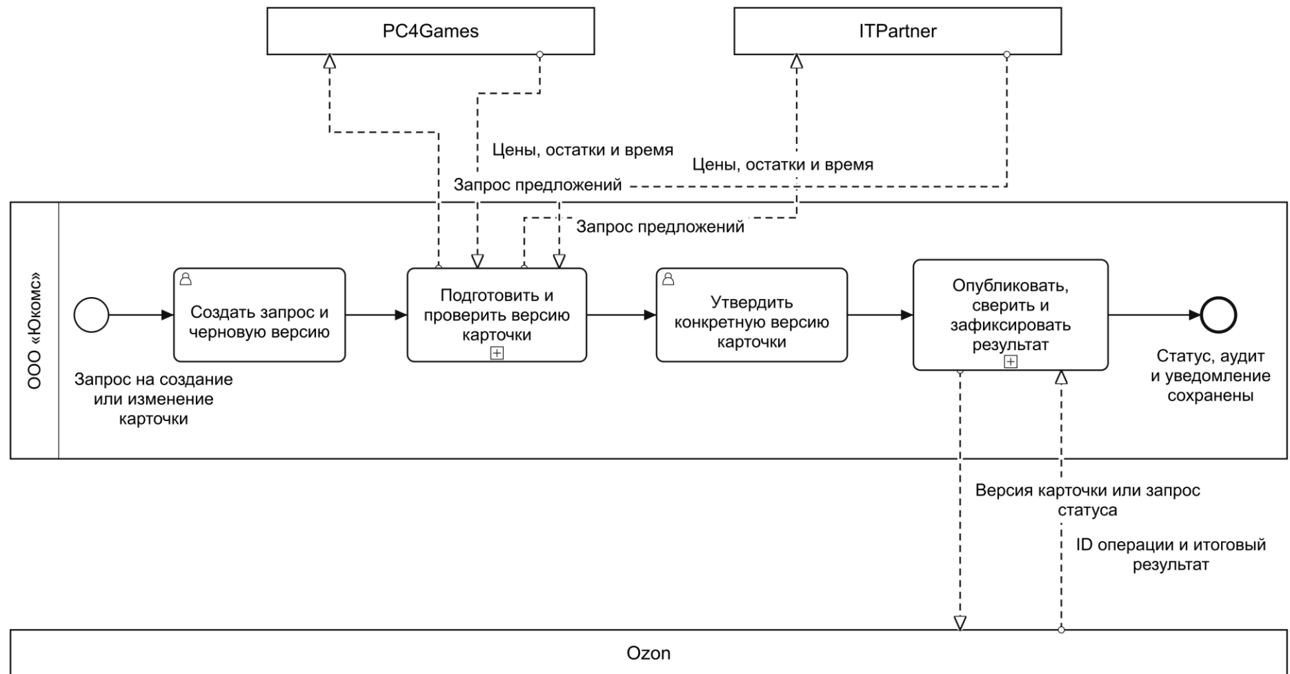
Рисунок 8 – BPMN TO BE: целевой процесс подготовки и публикации
