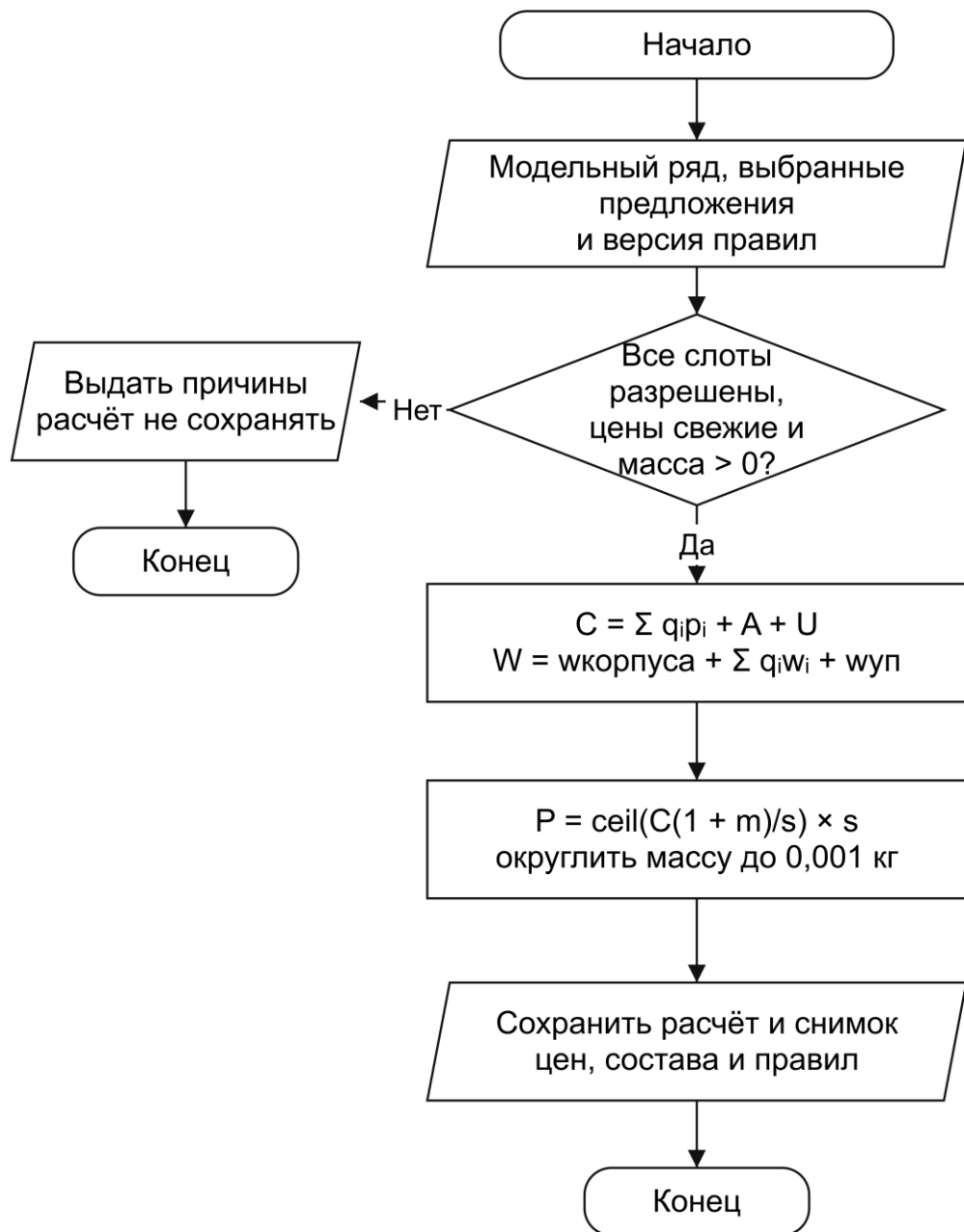
Рисунок 26 – Алгоритм расчёта цены и массы
