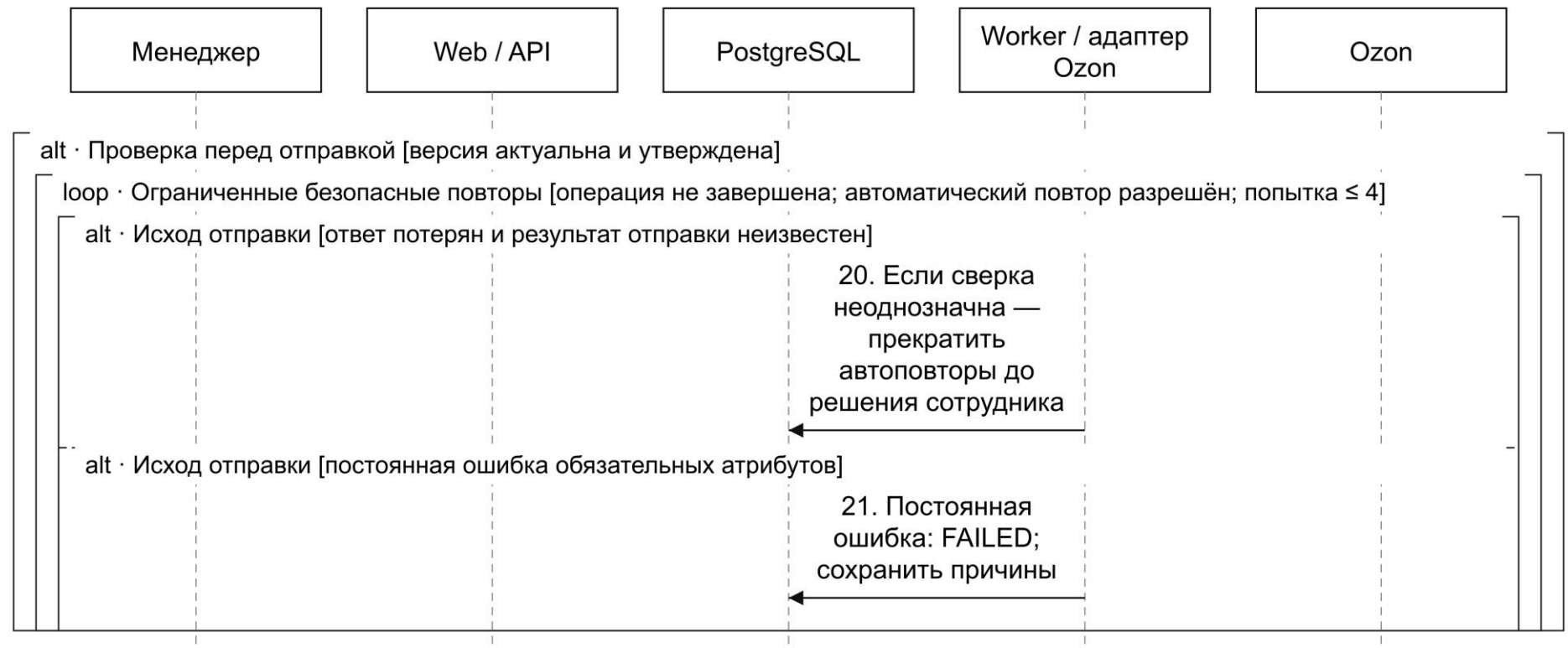
Продолжение рисунка 37 – Последовательность публикации версии карточки (часть 7 из 7)
