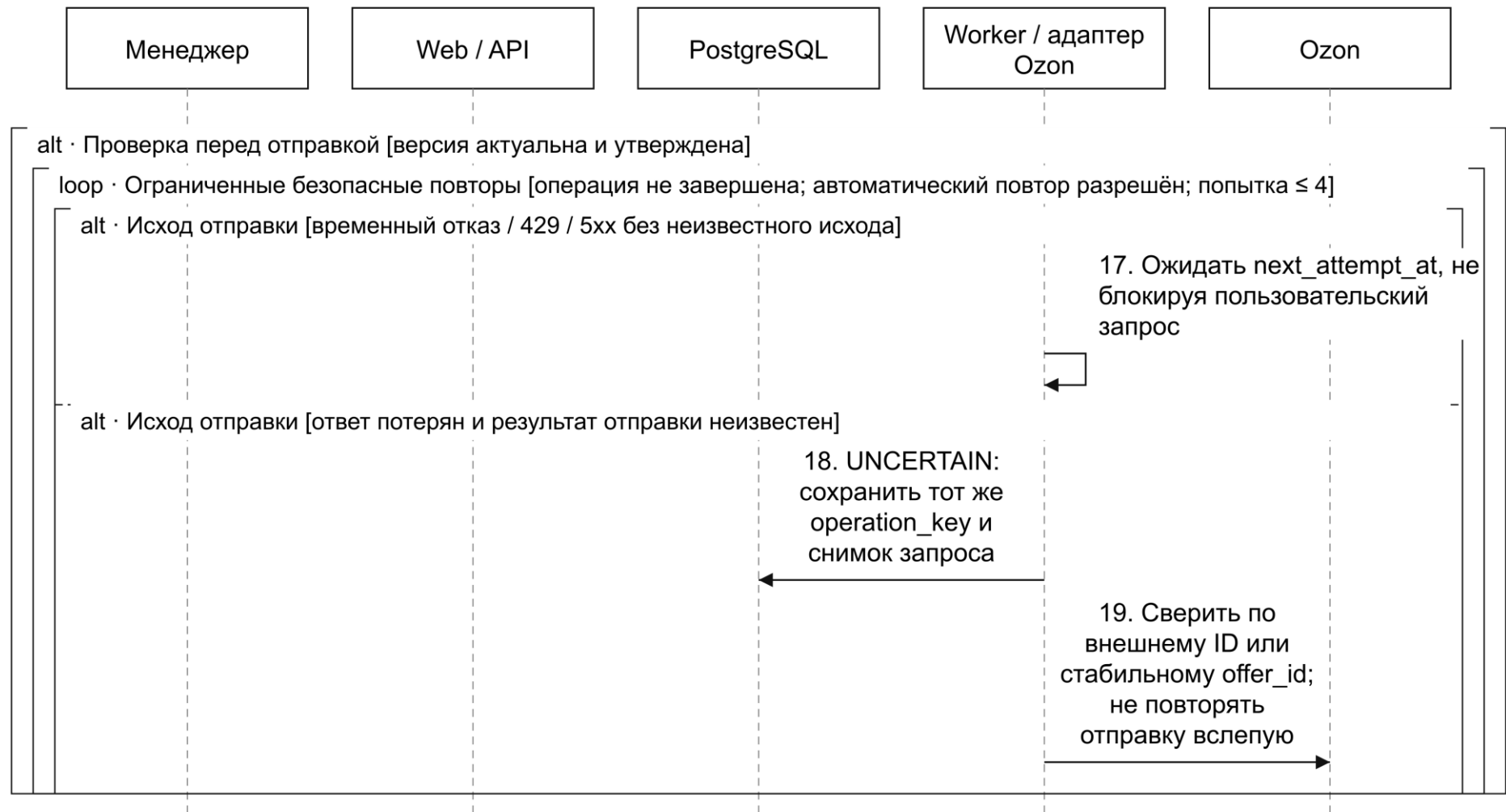
Продолжение рисунка 37 – Последовательность публикации версии карточки (часть 6 из 7)
