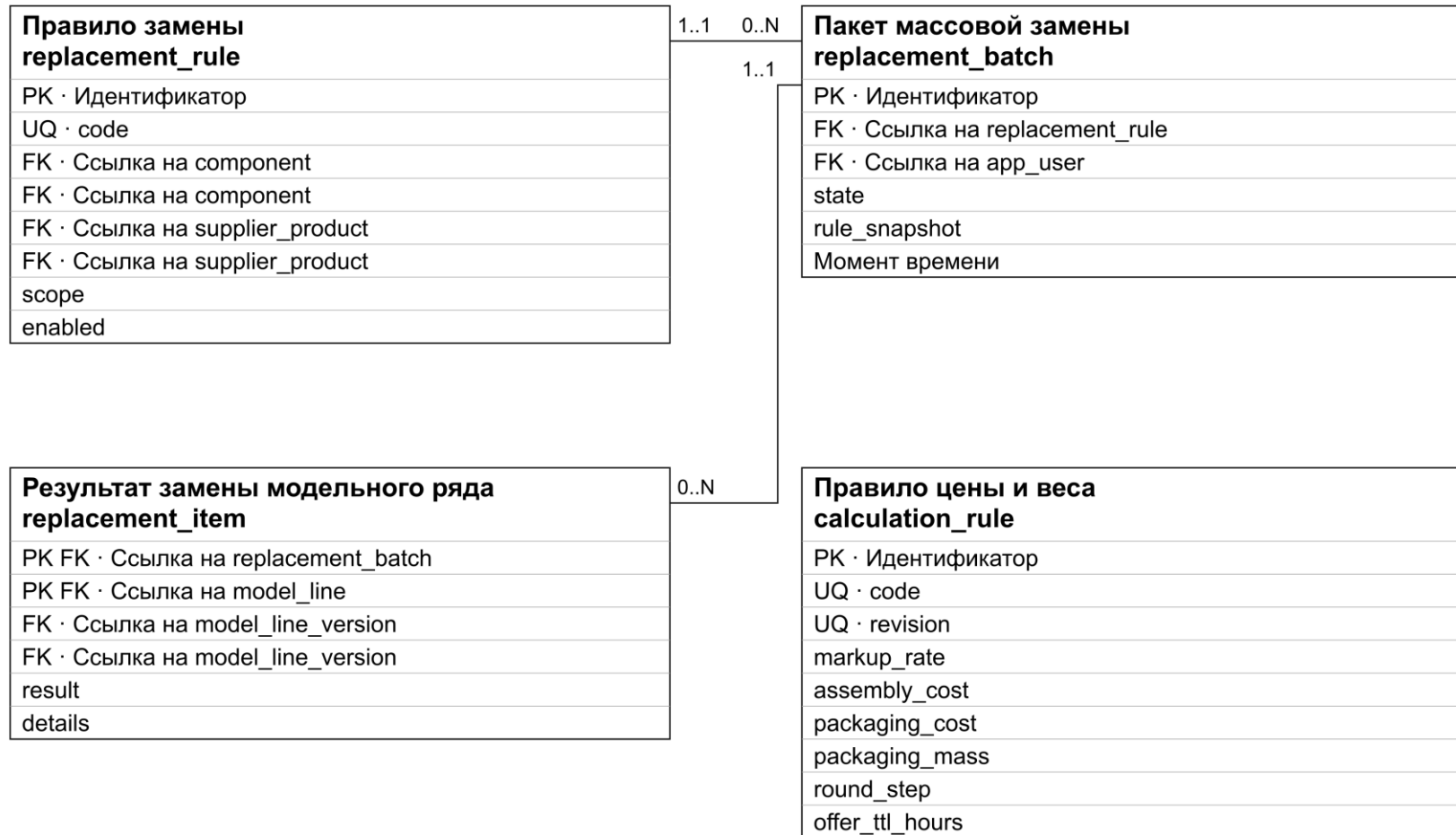
Рисунок 15 – Логическая модель данных, вид 3
