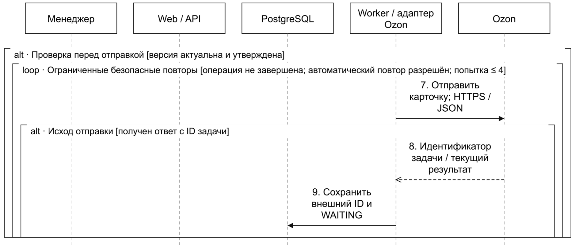
Продолжение рисунка 37 – Последовательность публикации версии карточки (часть 2 из 7)
