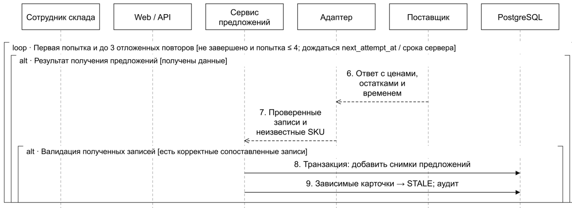
Продолжение рисунка 36 – Последовательность обновления предложений (часть 2 из 4)
