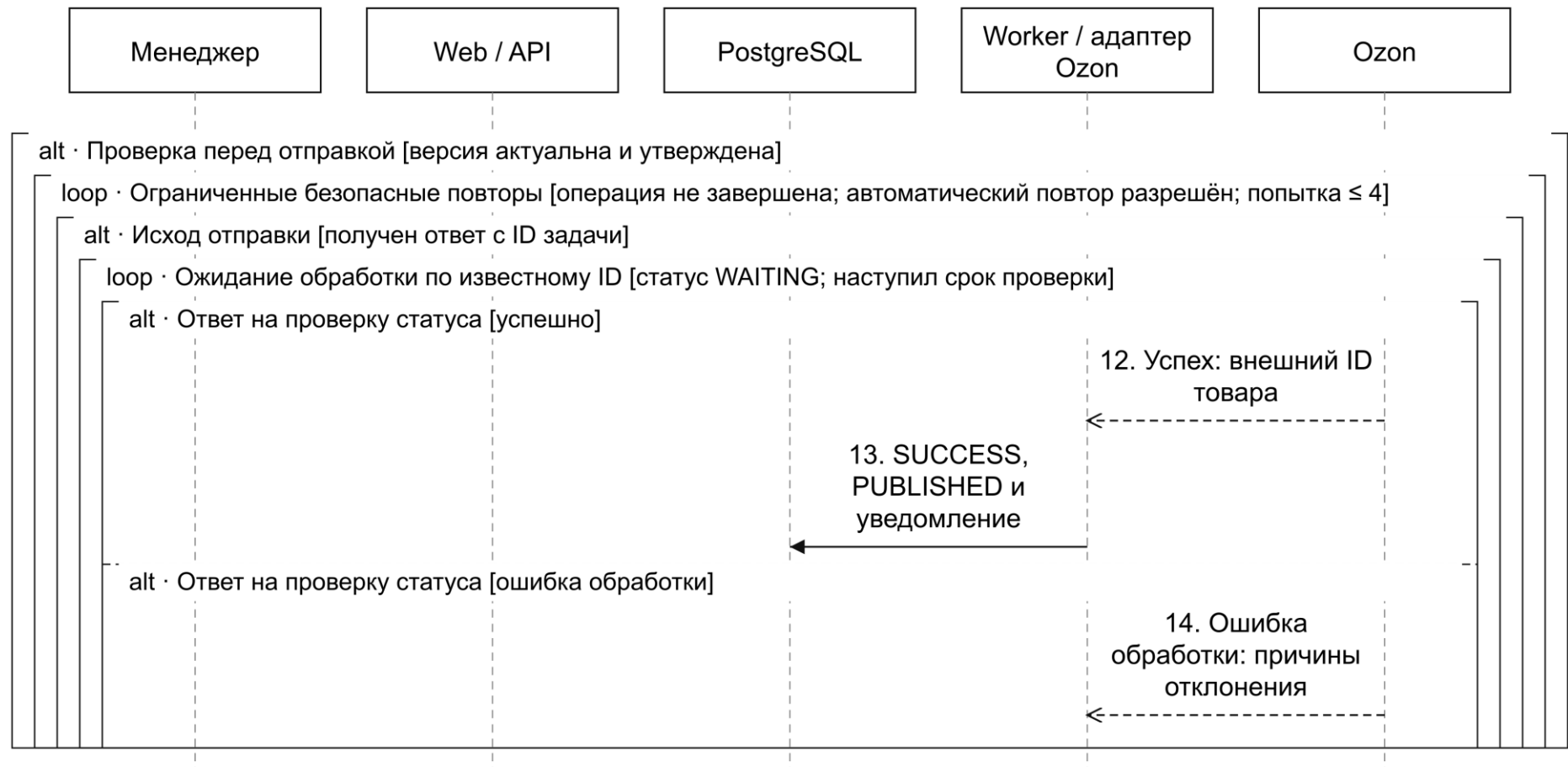
Продолжение рисунка 37 – Последовательность публикации версии карточки (часть 4 из 7)
