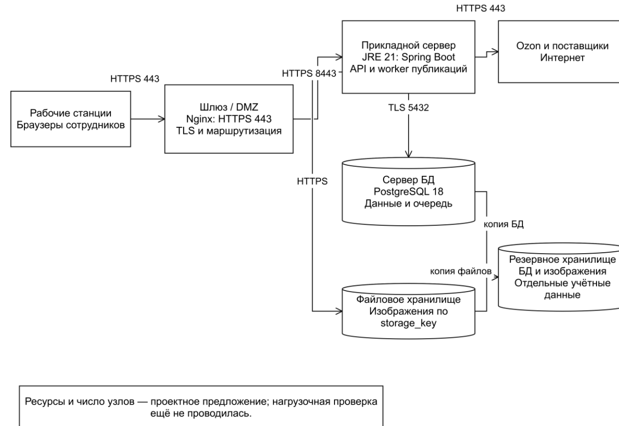
Рисунок 29 – Инфраструктурная схема
