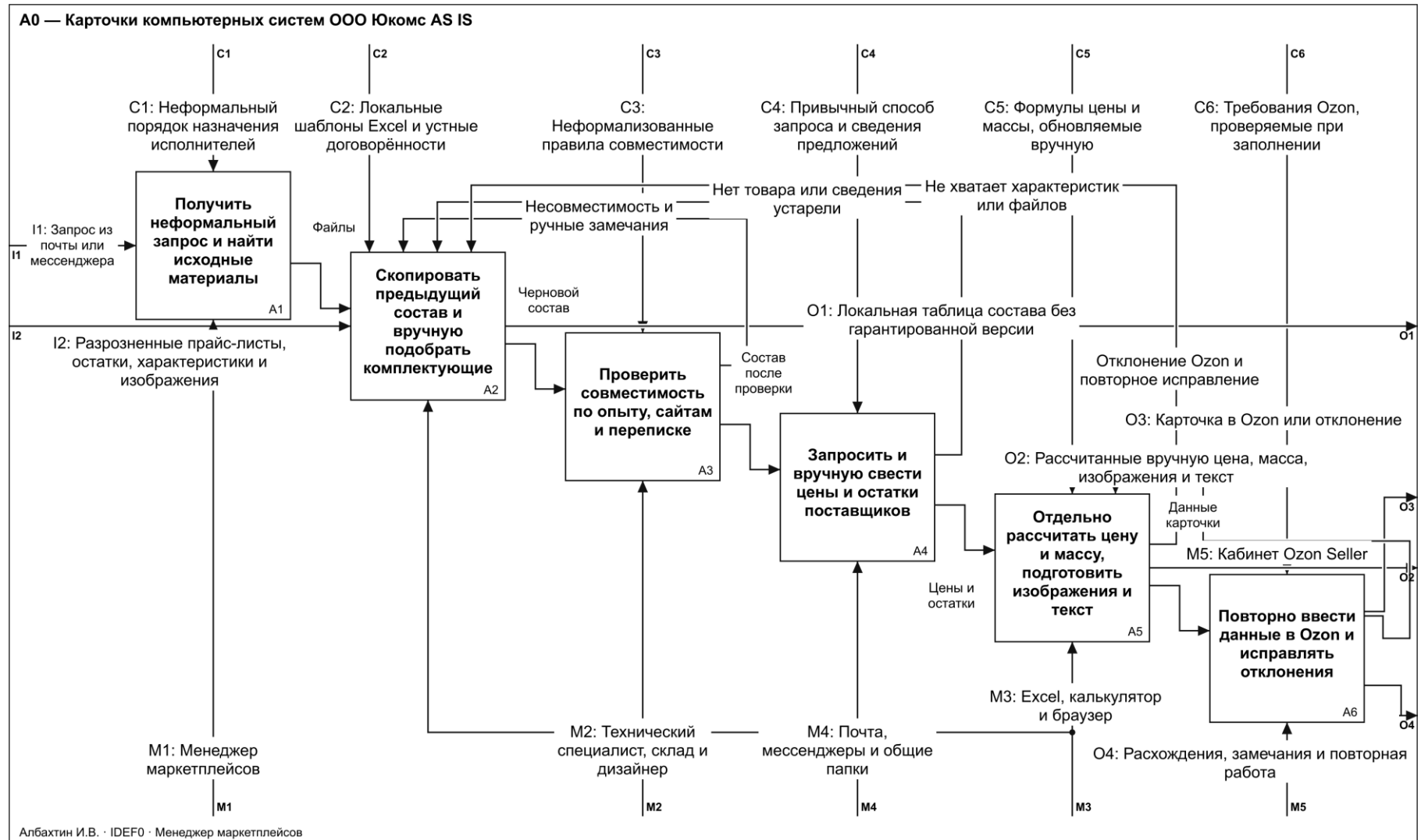
Рисунок 2 – IDEF0 AS IS: ручная подготовка и повторный ввод
