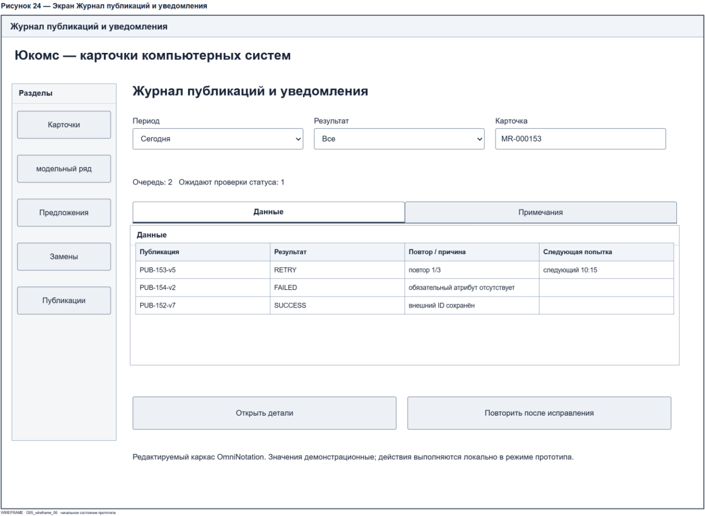
Рисунок 24 – Экран Журнал публикаций и уведомления
