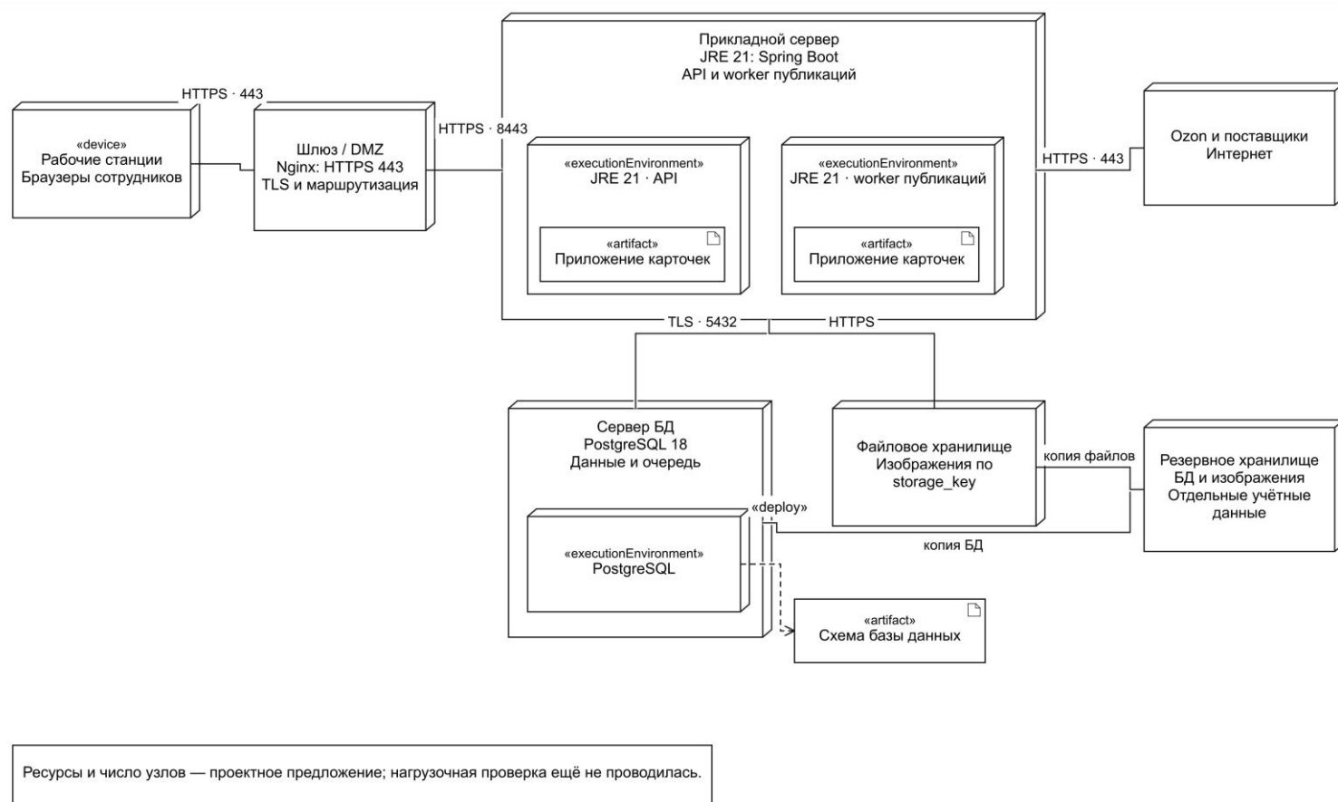
Рисунок 35 – Диаграмма развёртывания
