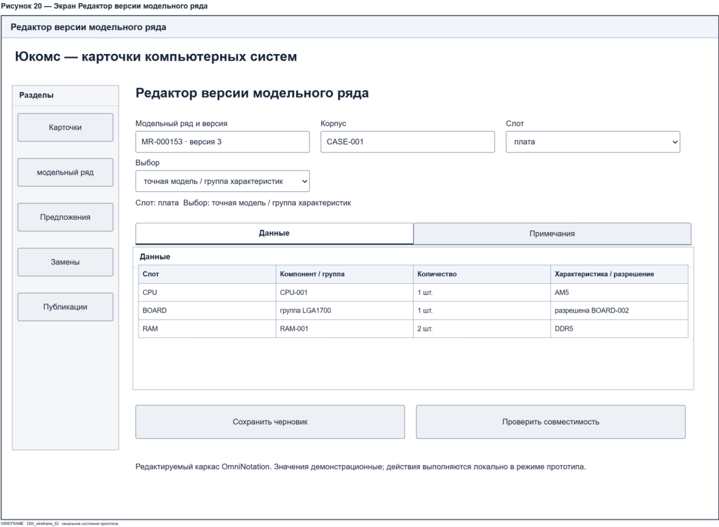
Рисунок 20 – Экран Редактор версии модельного ряда
