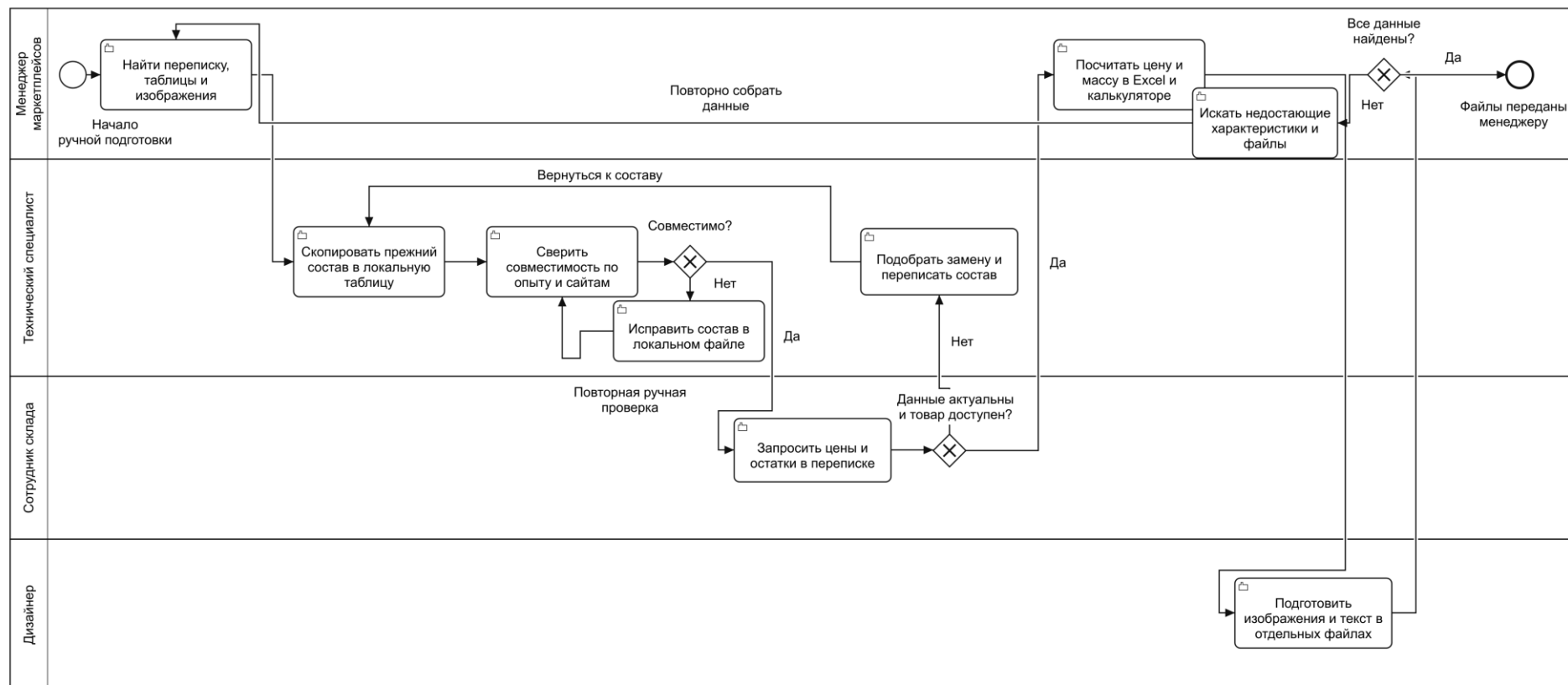
Рисунок 4 – BPMN AS IS: подготовка данных в разрозненных инструментах
