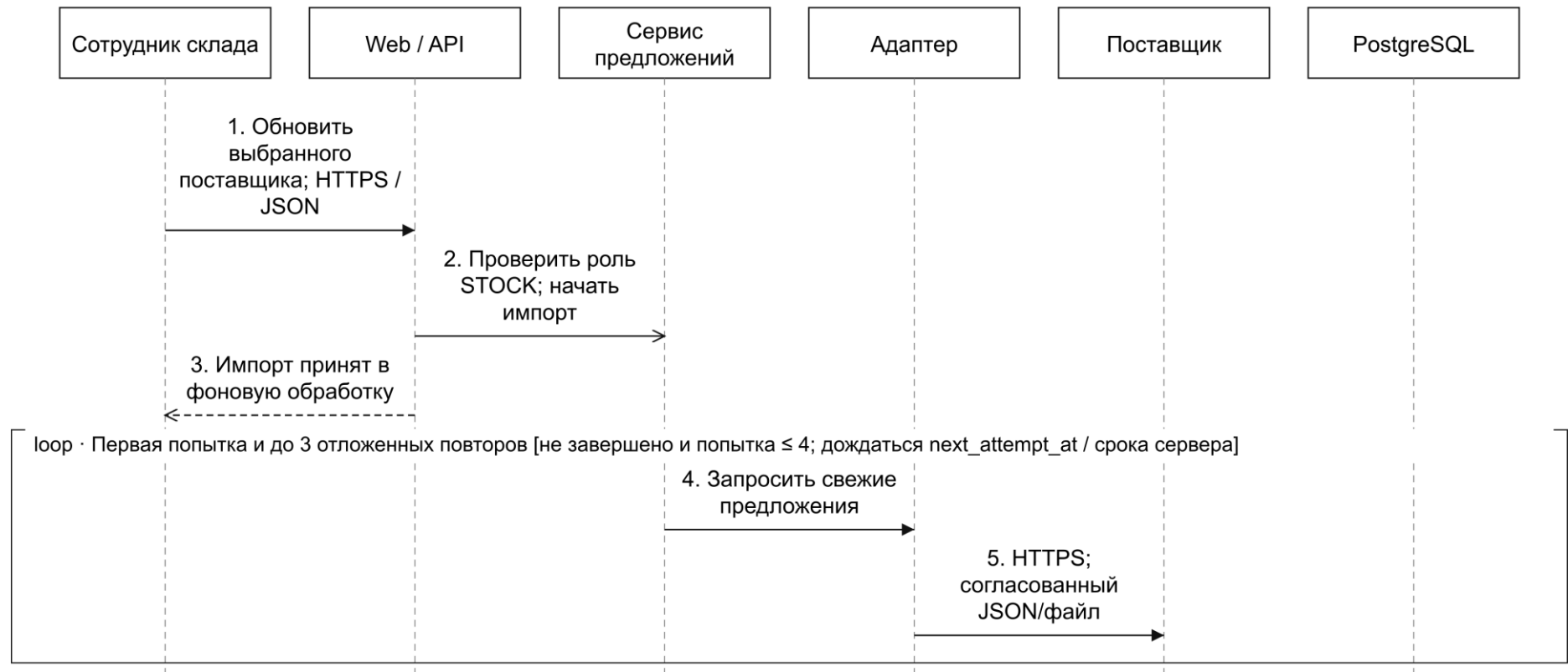
Рисунок 36 – Последовательность обновления предложений (часть 1 из 4)
