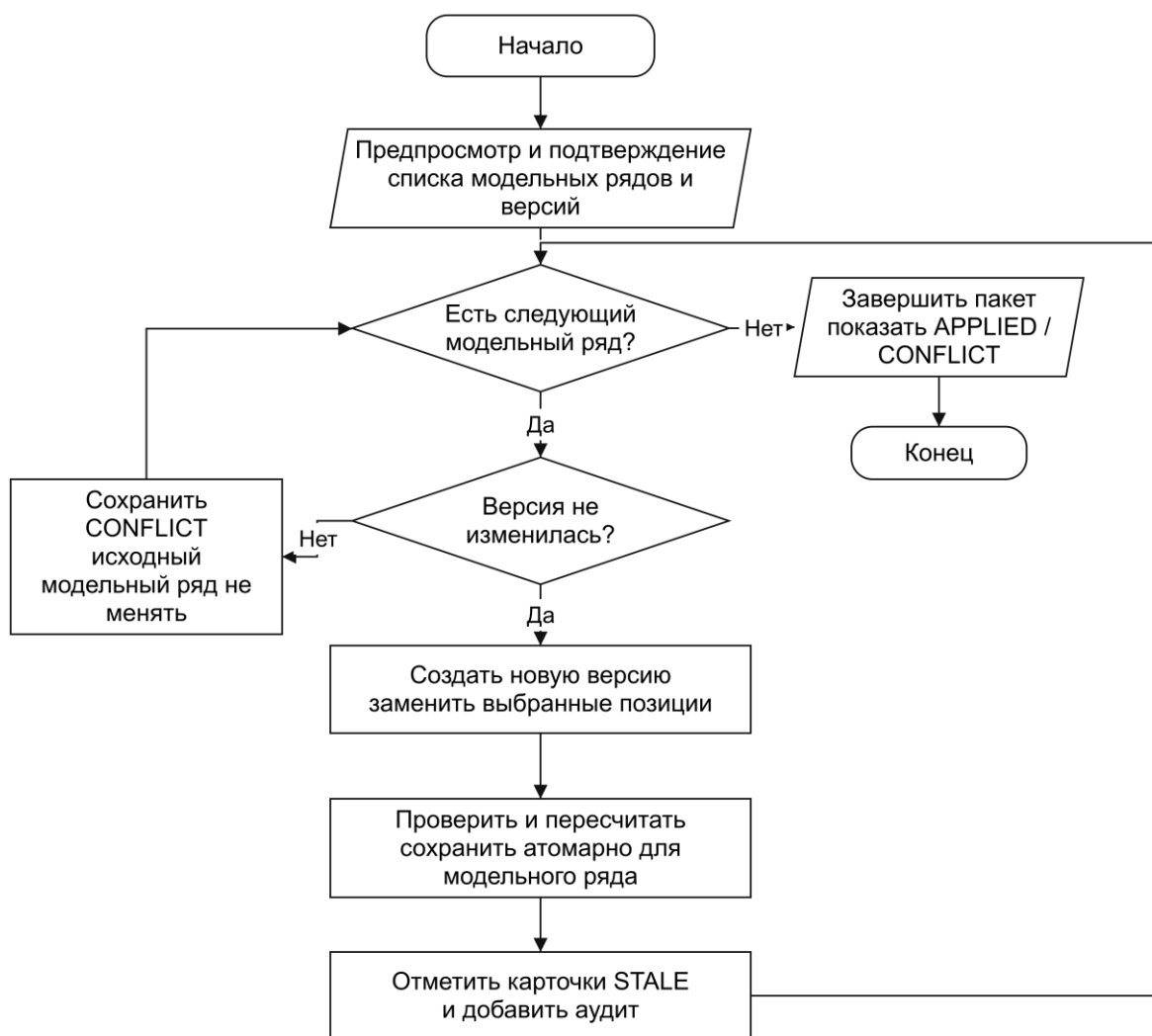
Рисунок 28 – Алгоритм массовой замены
