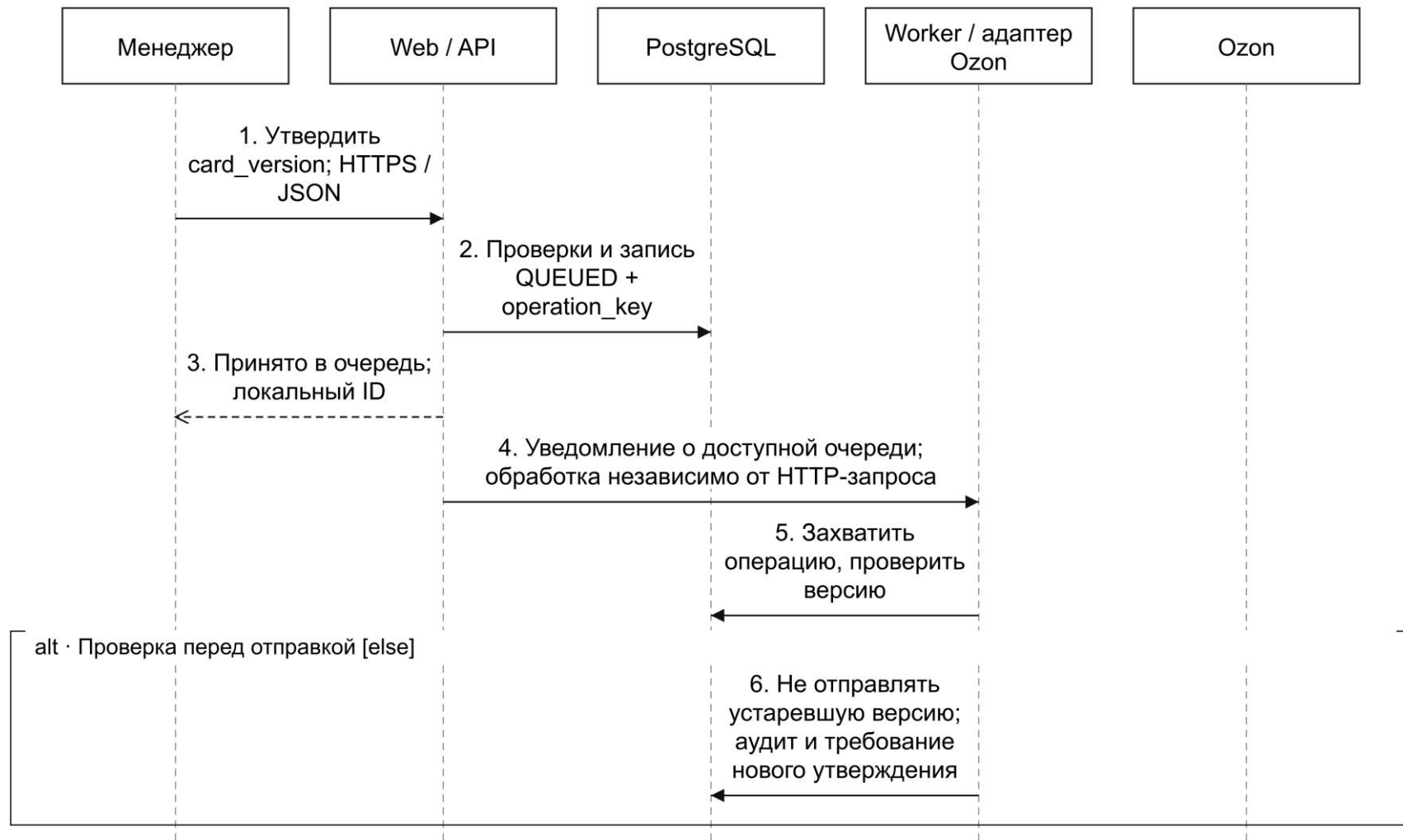
Рисунок 37 – Последовательность публикации версии карточки (часть 1 из 7)
