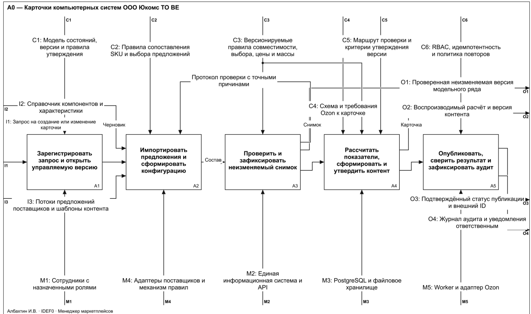
Рисунок 7 – IDEF0 TO BE: версионированная подготовка и публикация
