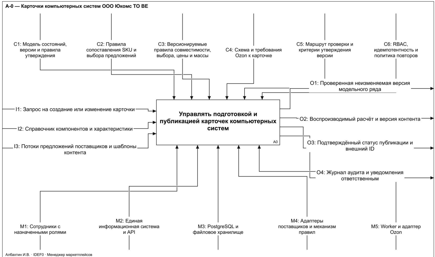
Рисунок 6 – IDEF0 TO BE: контекст управляемого процесса
