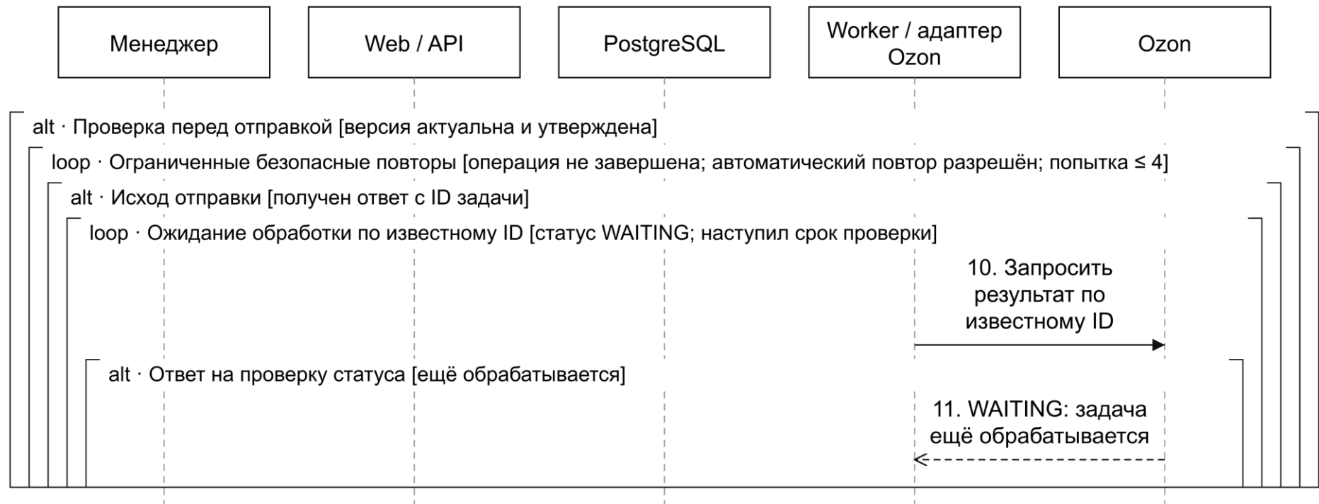
Продолжение рисунка 37 – Последовательность публикации версии карточки (часть 3 из 7)
