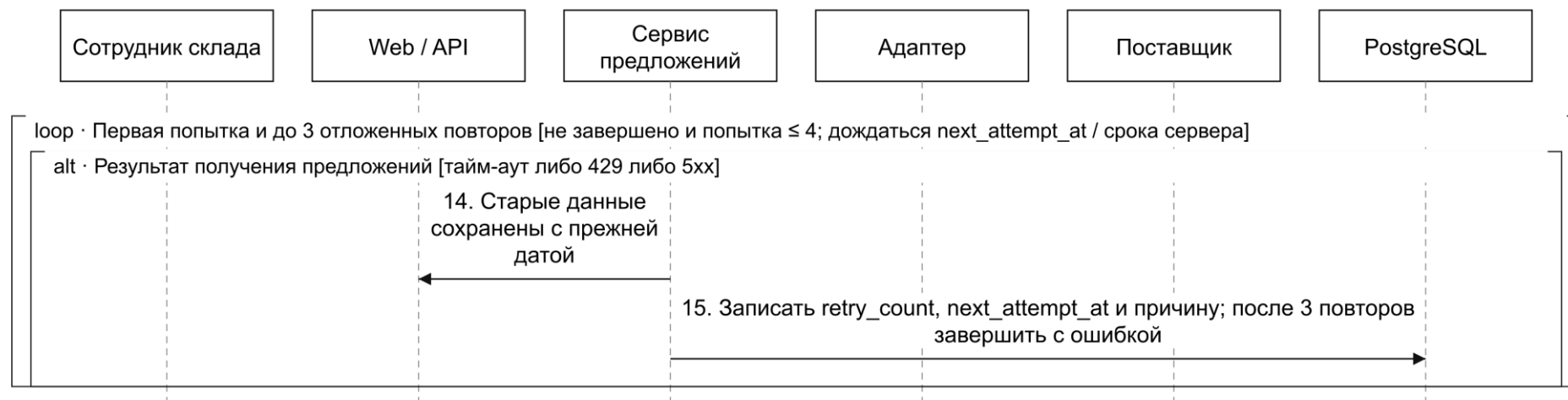
Продолжение рисунка 36 – Последовательность обновления предложений (часть 4 из 4)
