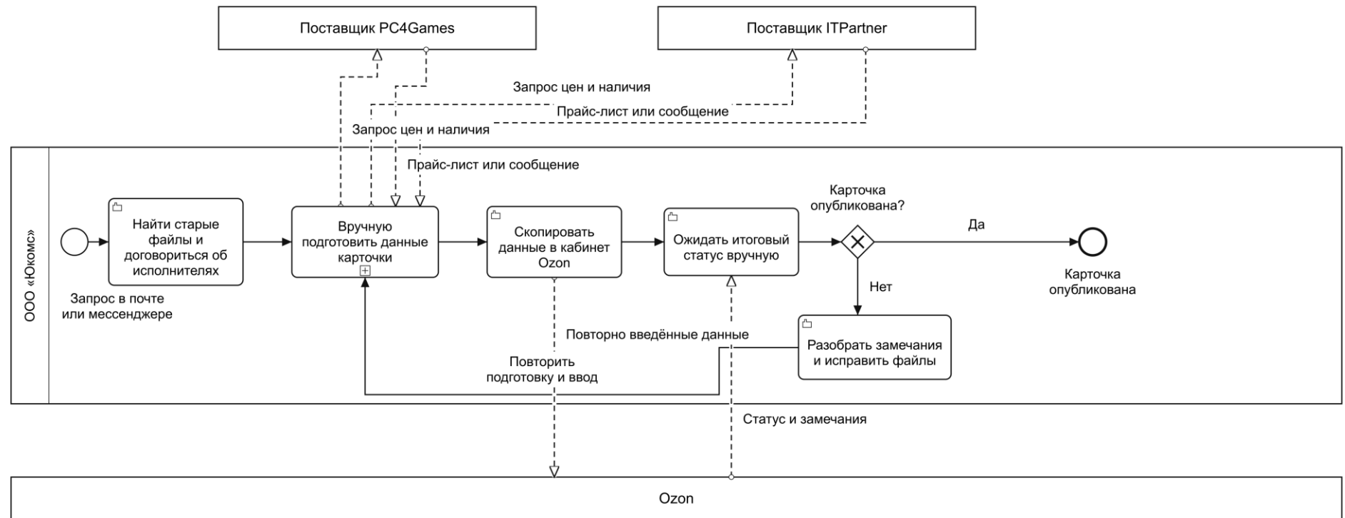
Рисунок 3 – BPMN AS IS: ручная публикация и возврат отклонённой карточки
