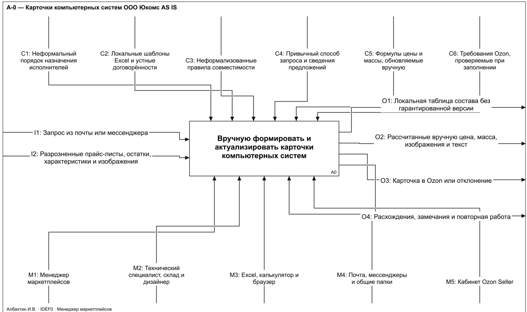
Рисунок 1 – IDEF0 AS IS: контекст ручной подготовки карточки
