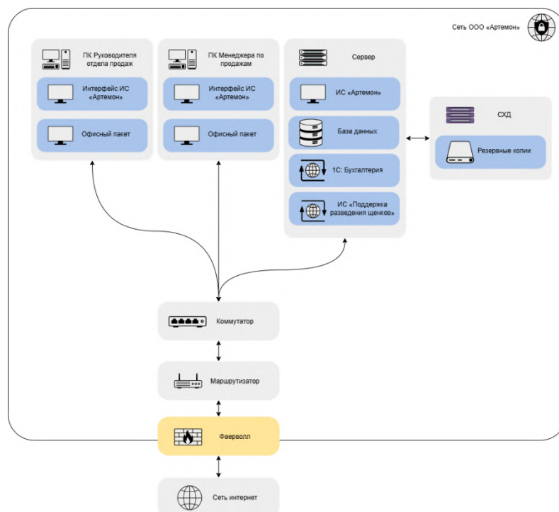
Рисунок 2.29 — ИТ-инфраструктура
