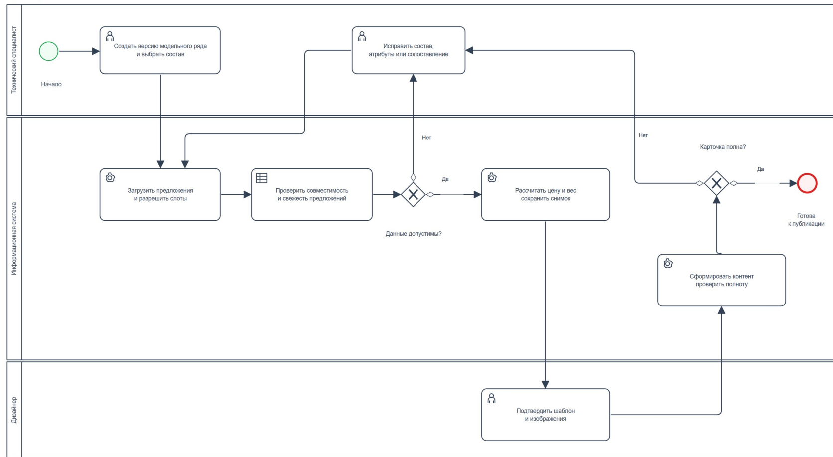
Рисунок 09 — Подготовить версию карточки
