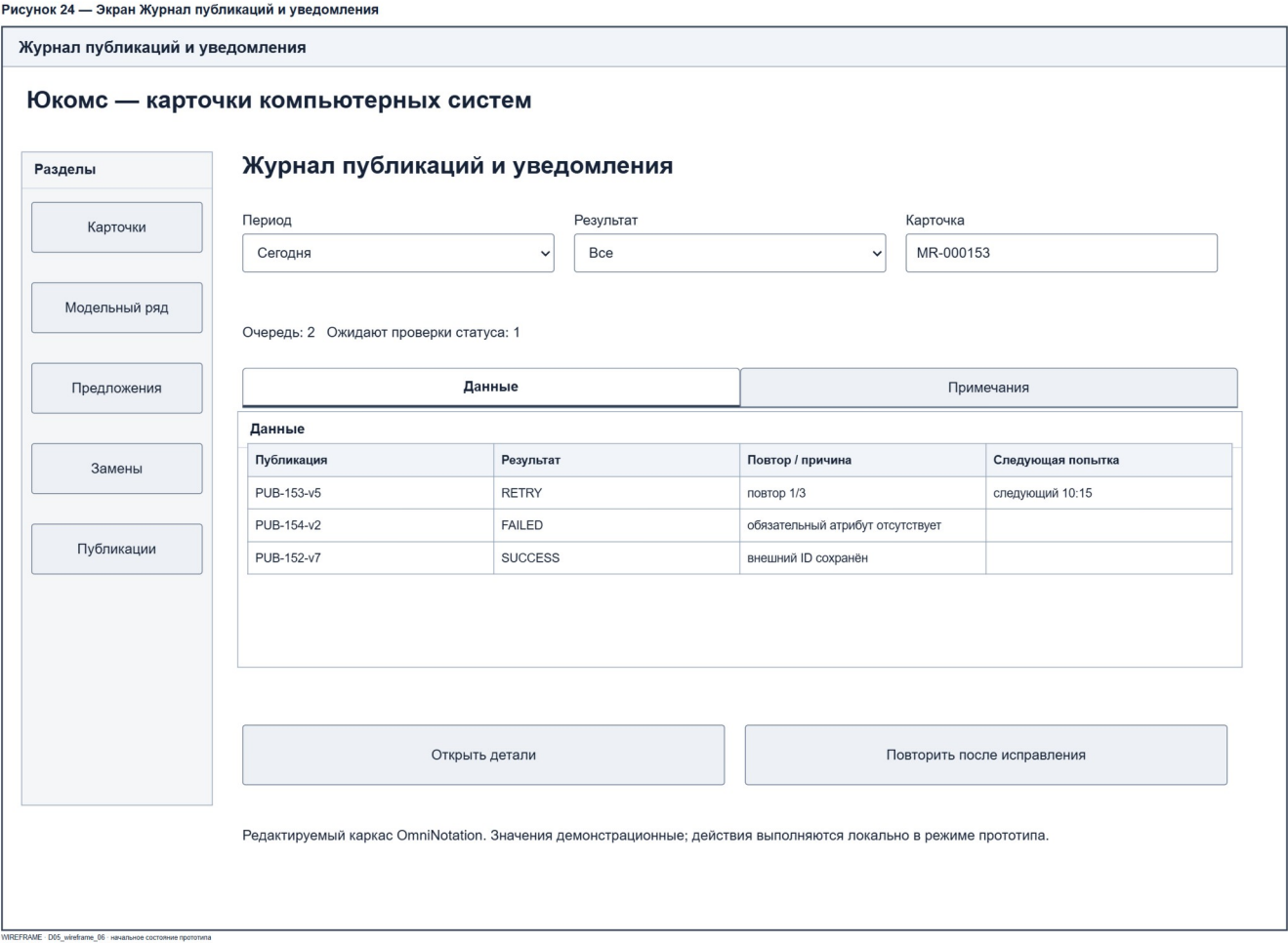
Рисунок 24 – Экран Журнал публикаций и уведомления
