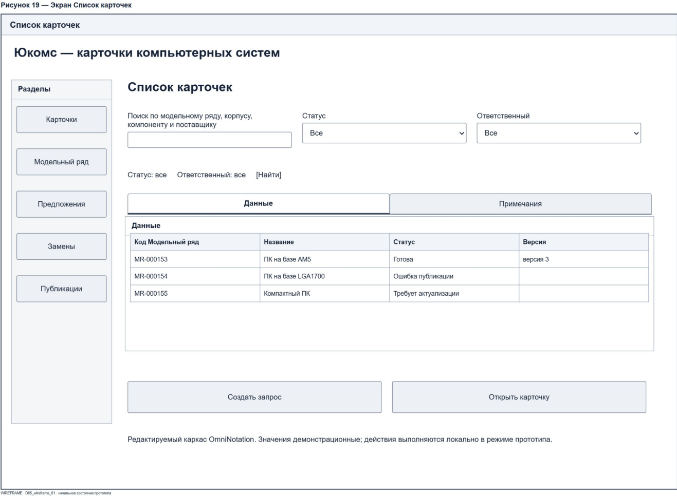
Рисунок 19 – Экран Список карточек
