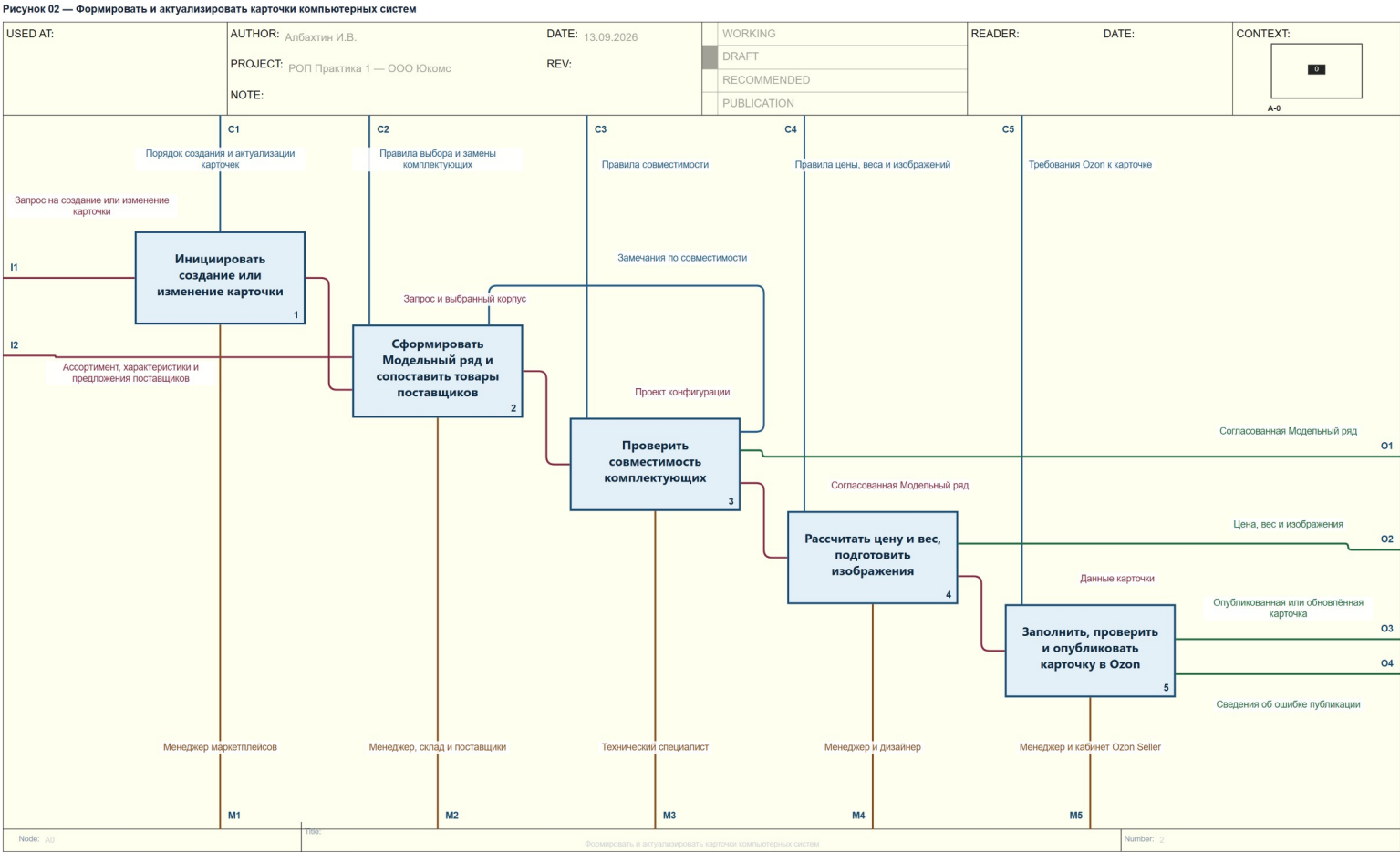
Рисунок 2 – Формировать и актуализировать карточки компьютерных систем
