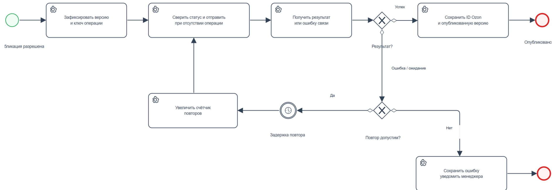
Рисунок 10 — Опубликовать и обработать результат
