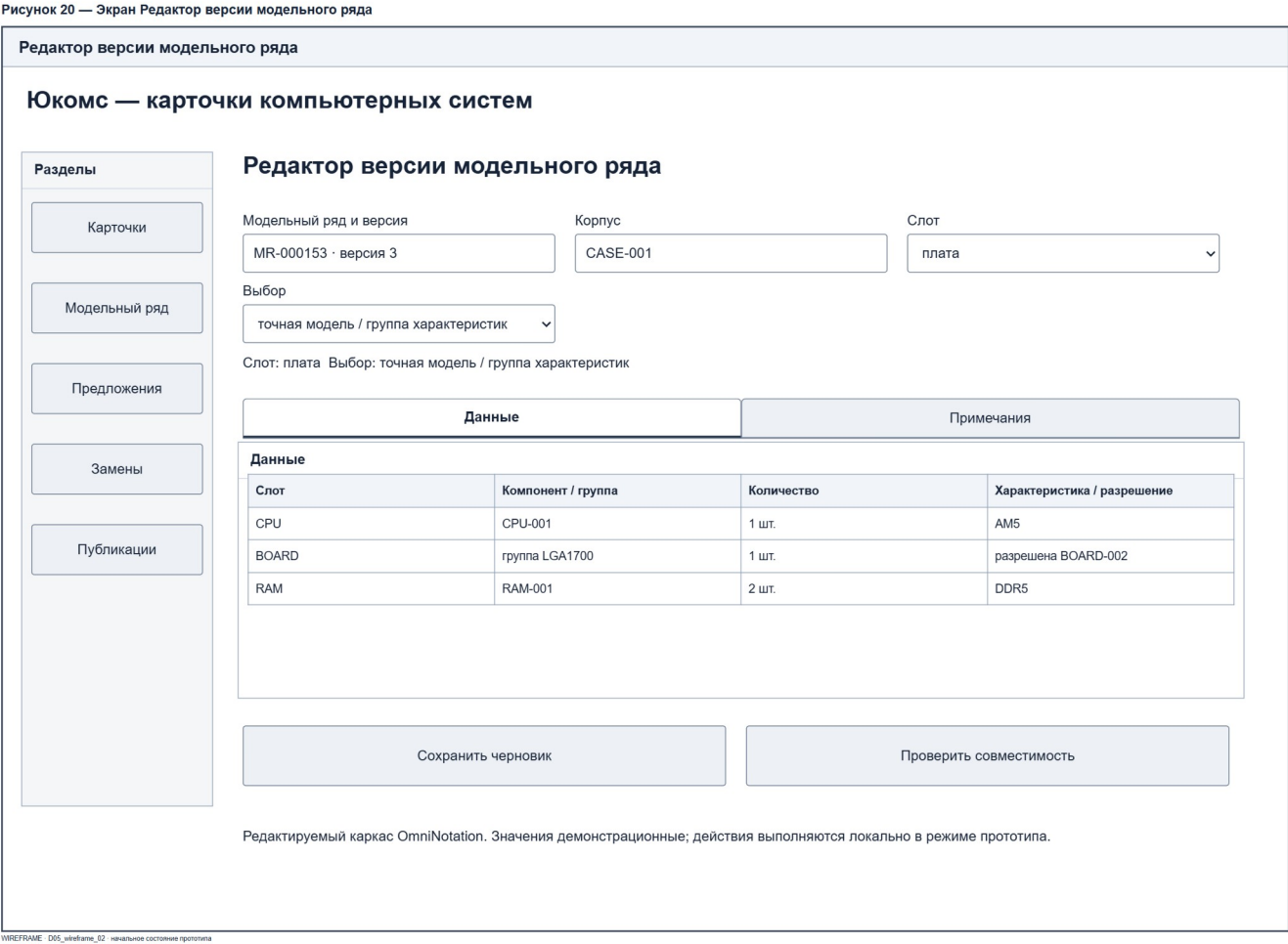
Рисунок 20 – Экран Редактор версии модельного ряда
