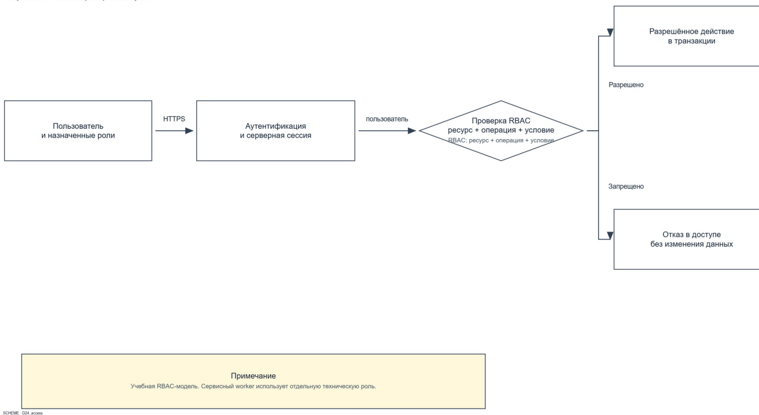
Рисунок 38 — Схема проверки доступа
