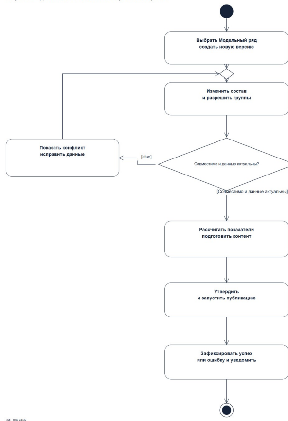
Рисунок 25 – Деятельность по подготовке и публикации карточки
