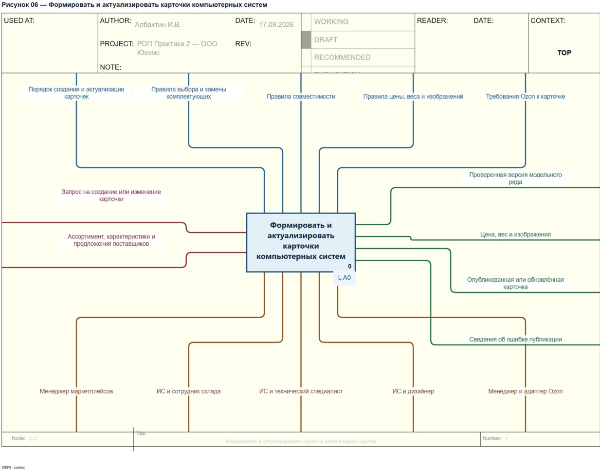
Рисунок 6 – Формировать и актуализировать карточки компьютерных систем
