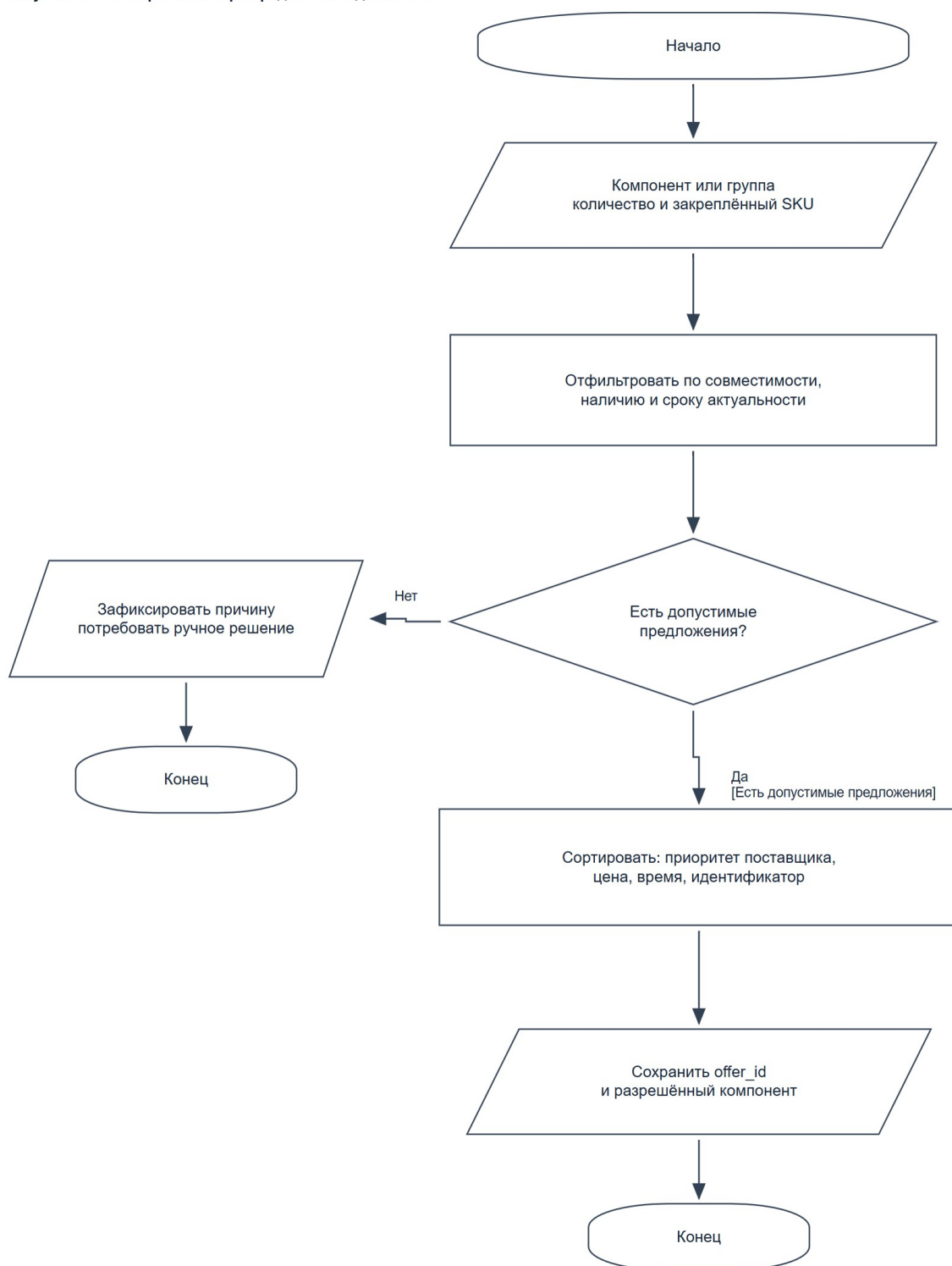
Рисунок 27 — Алгоритм выбора предложения для слота
