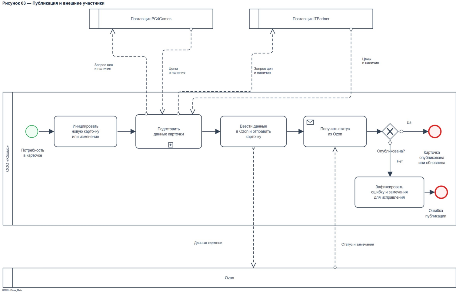
Рисунок 3 – Публикация и внешние участники
