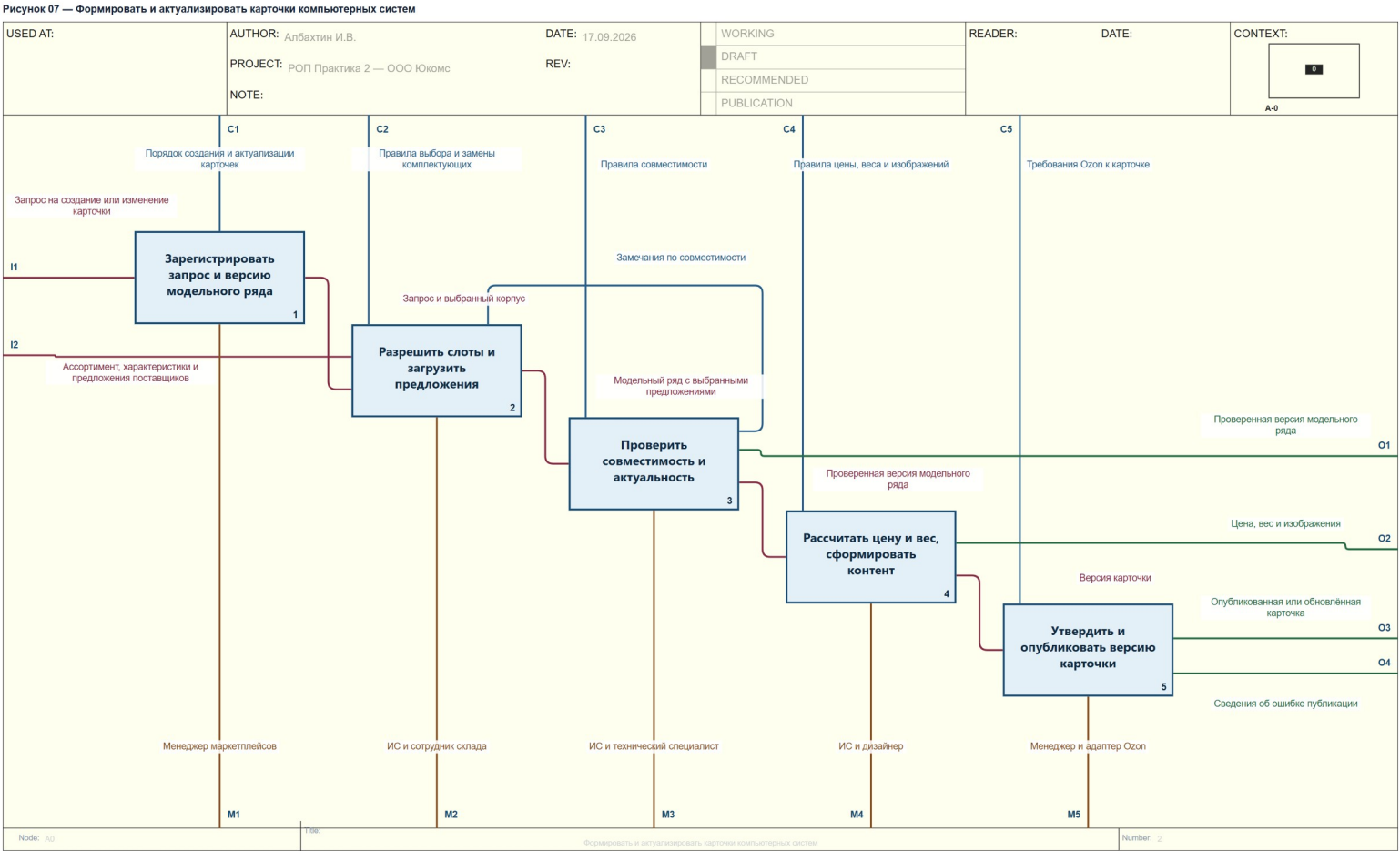
Рисунок 7 – Формировать и актуализировать карточки компьютерных систем
