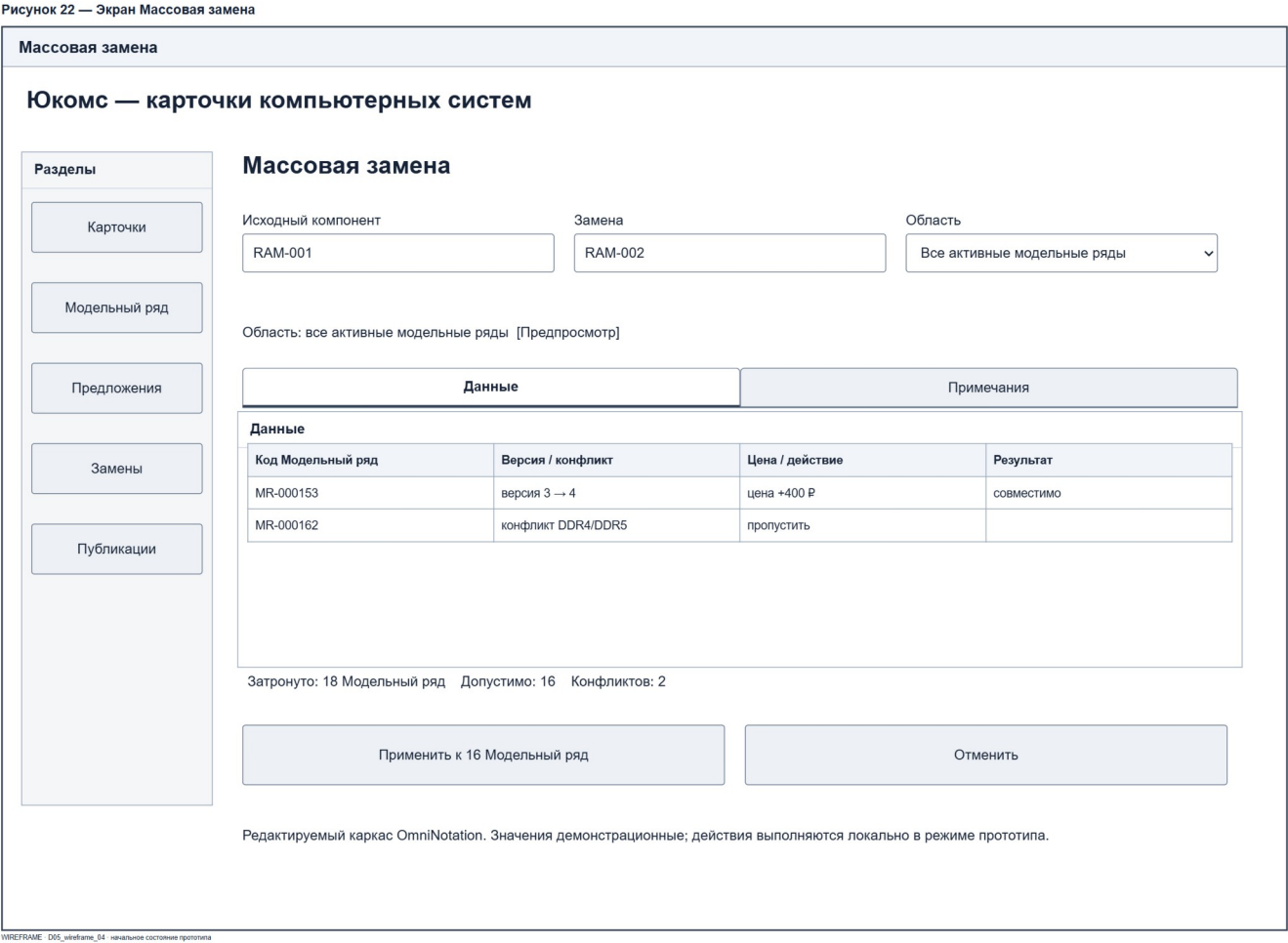
Рисунок 22 – Экран Массовая замена
