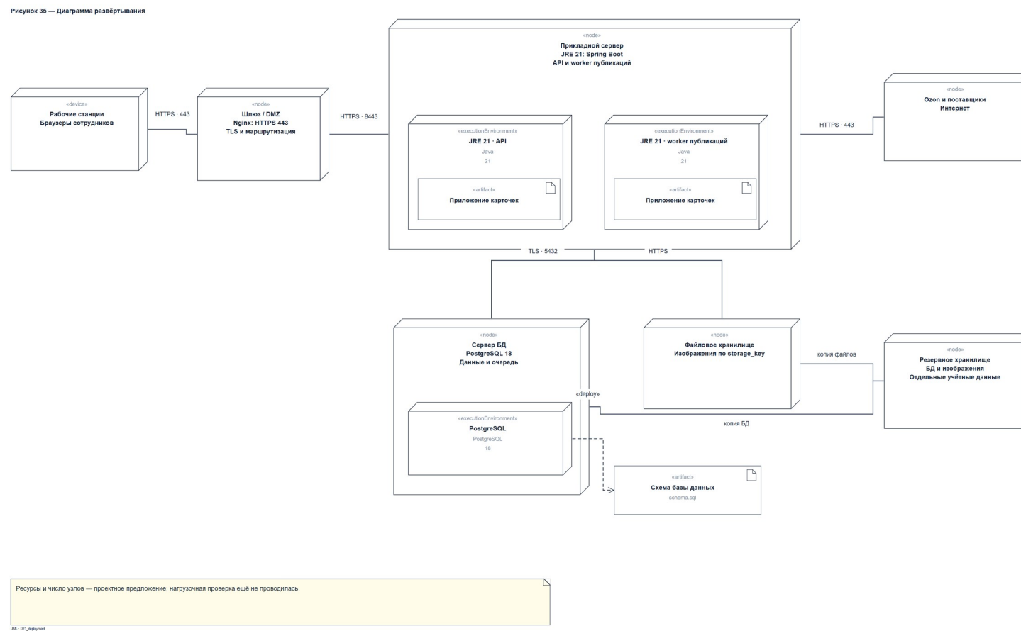
Рисунок 35 – Диаграмма развёртывания
