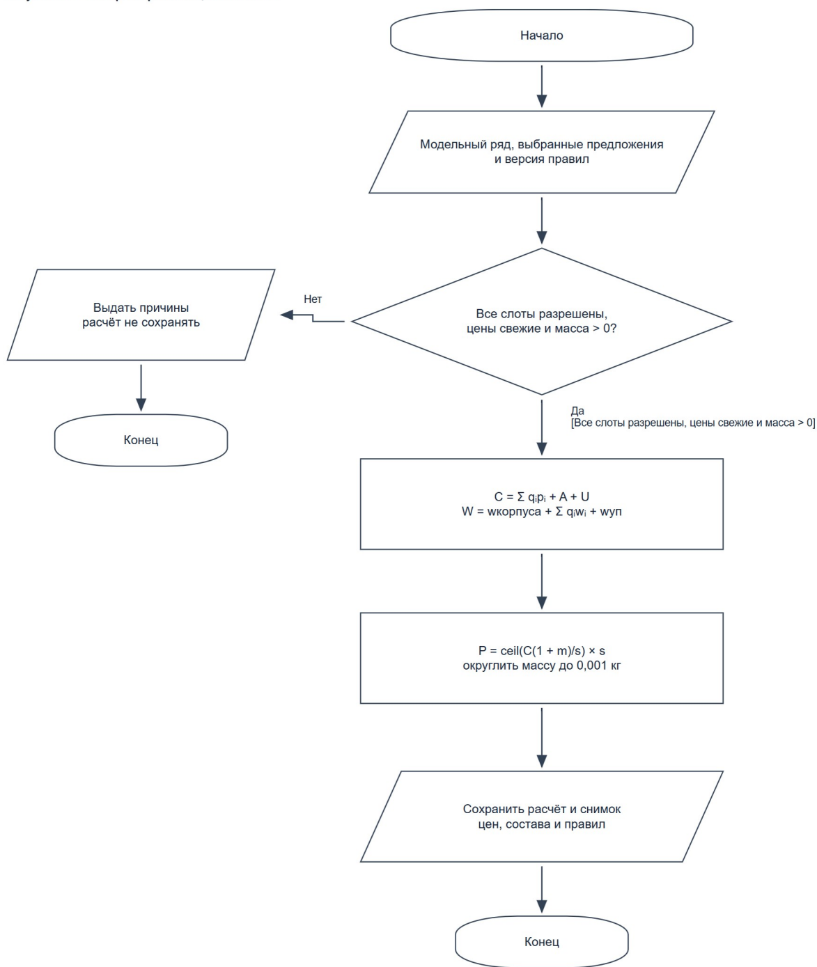
Рисунок 26 — Алгоритм расчёта цены и массы
