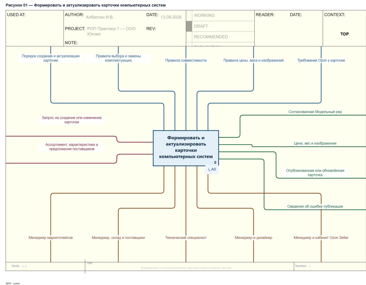
Рисунок 1 – Формировать и актуализировать карточки компьютерных систем
