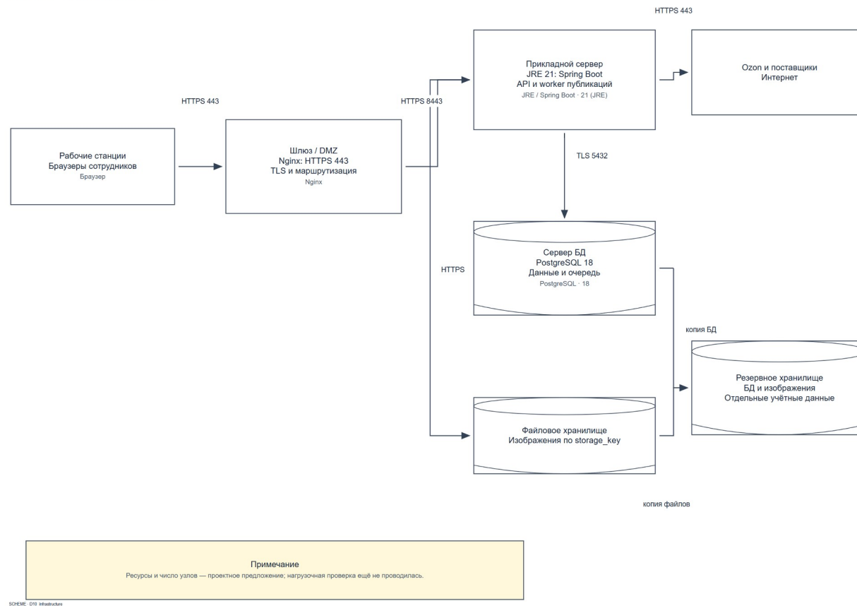
Рисунок 29 – Инфраструктурная схема
