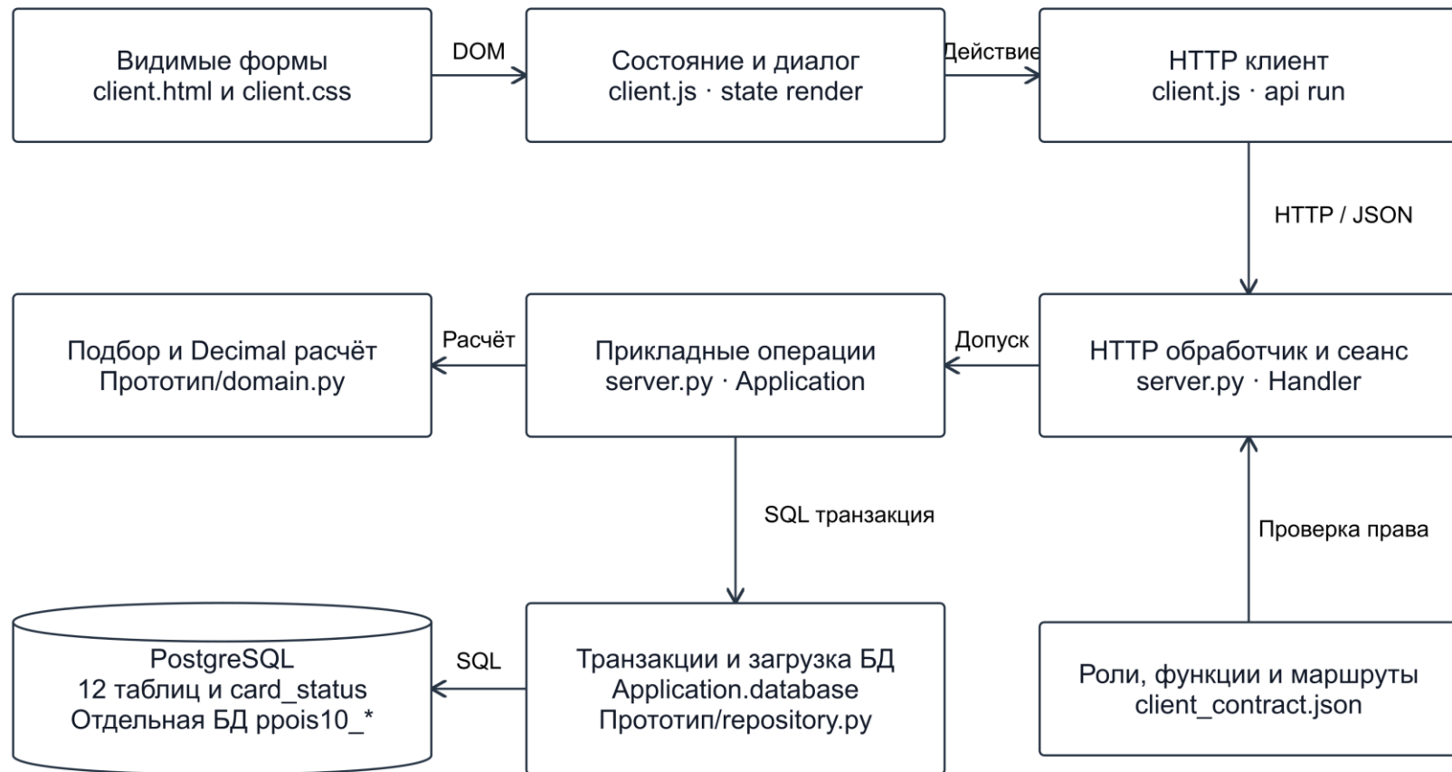
Рисунок 12 – Структурная схема версии 0.2
