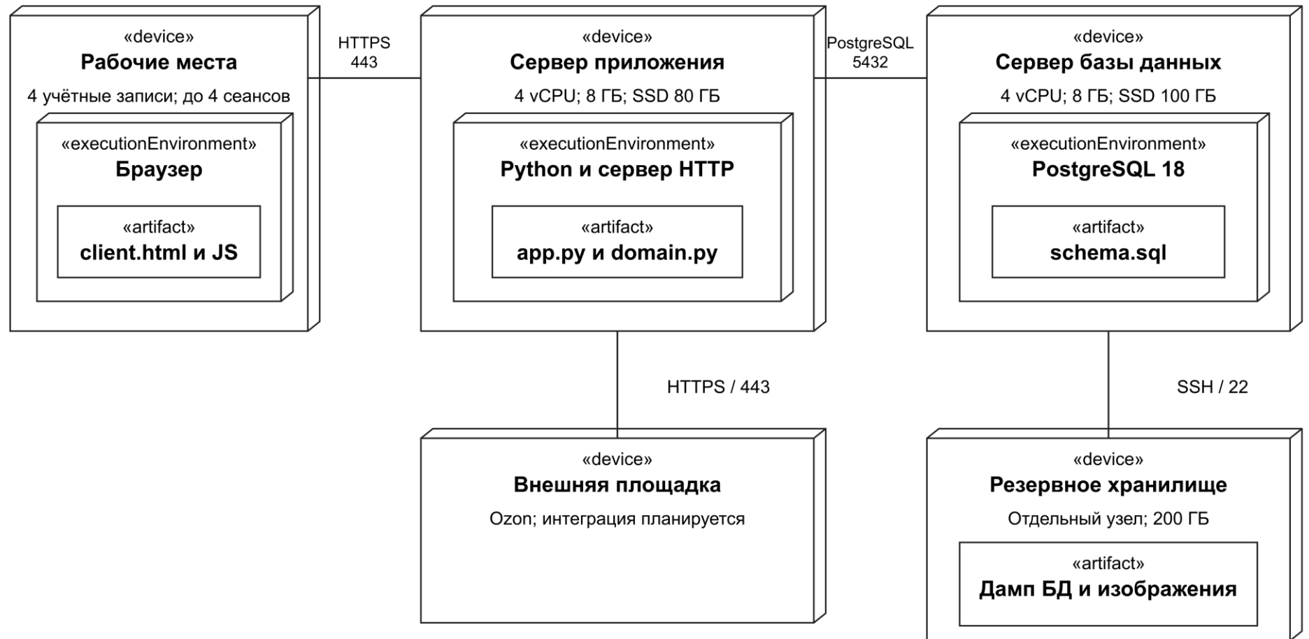
Рисунок 2 – Целевое размещение узлов и артефактов
