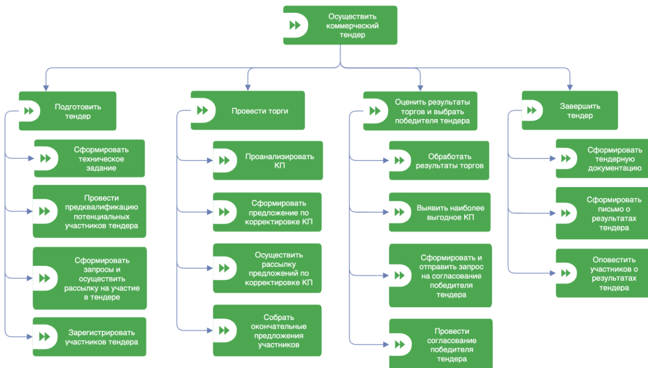
Рисунок 2.1 — Дерево функций
