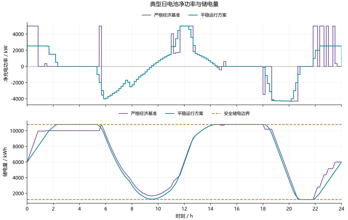
图1 典型日电池净充电功率与储电轨迹
