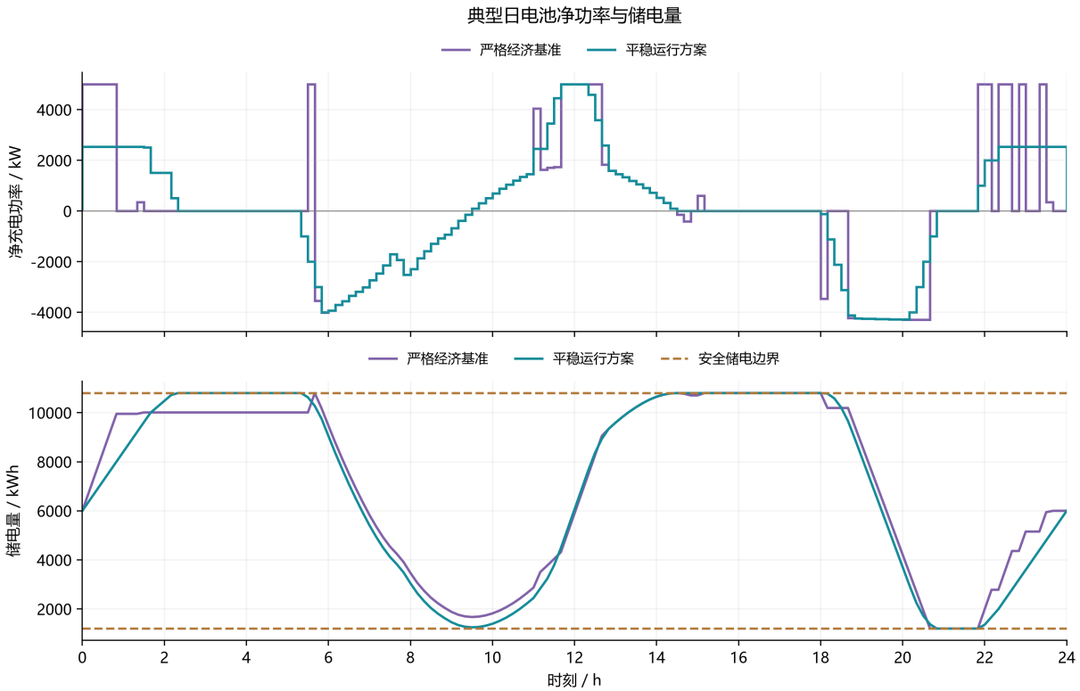
图 2 典型日电池净充电功率与储电轨迹
