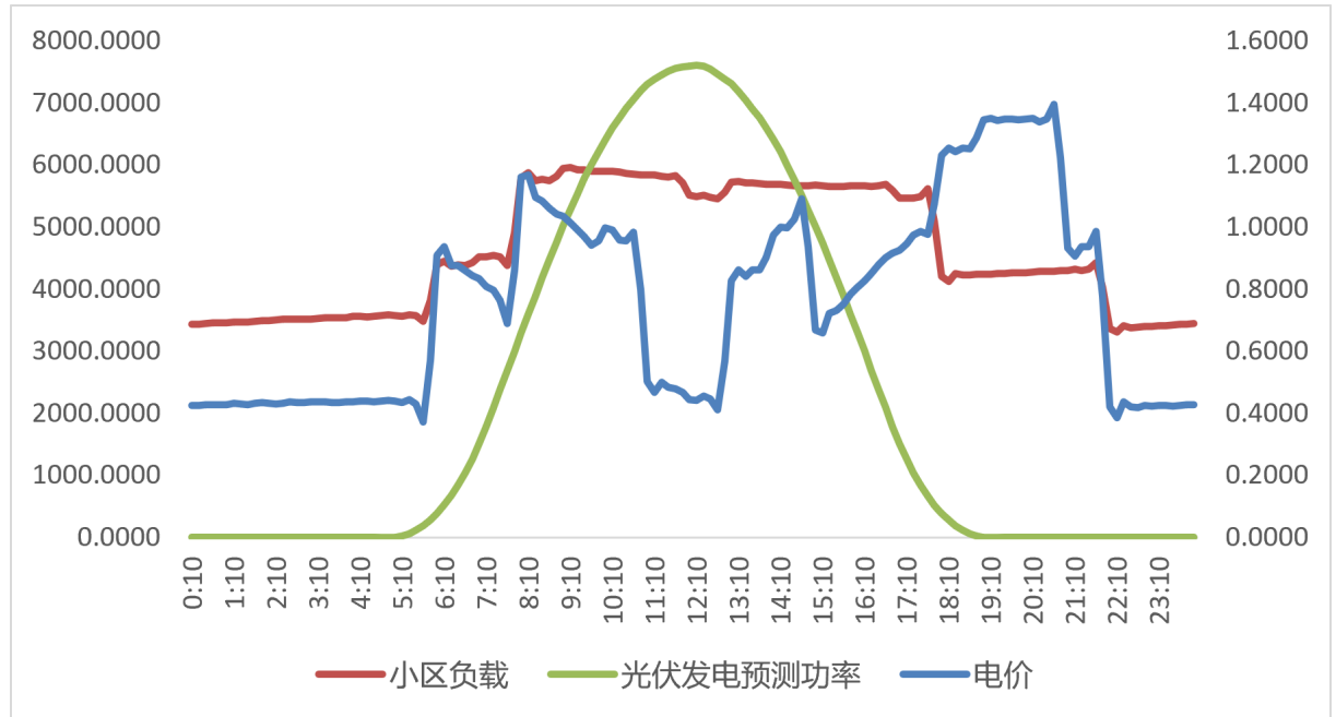
图 1 典型日负载、发电与电价
