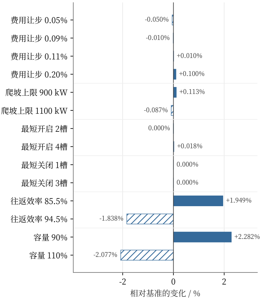
(a) 购电费用变化
