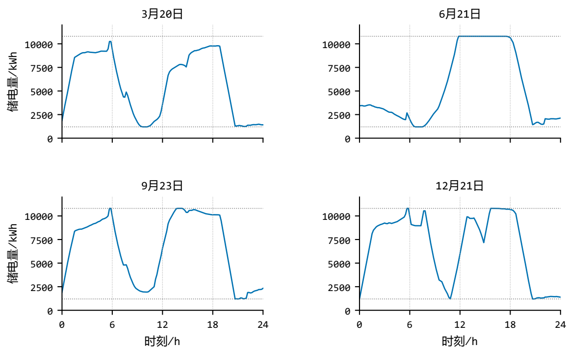
图 6 四个指定日的储电量轨迹。左上、右上、左下、右下依次为 3 月 20 日、6 月 21 日、9 月 23 日、12 月 21 日；水平虚线为 1200 与 10800 kWh 安全边界。
