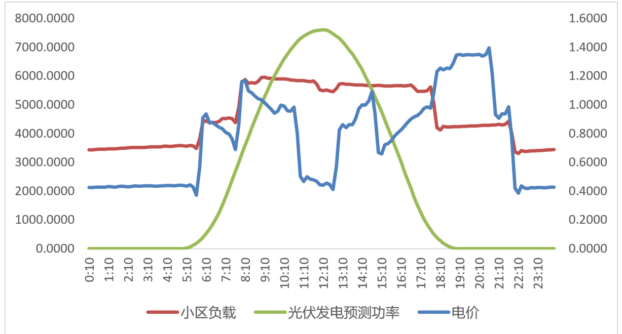
图2 典型日负载、光伏与电价
