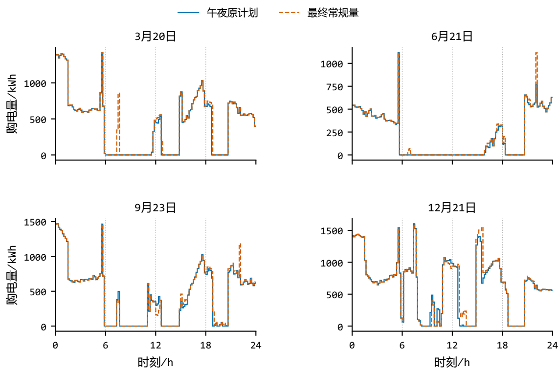
图 5 四个指定日的午夜原计划与最终常规购电量。竖线为 6、12、18 时的预报发布时间。
