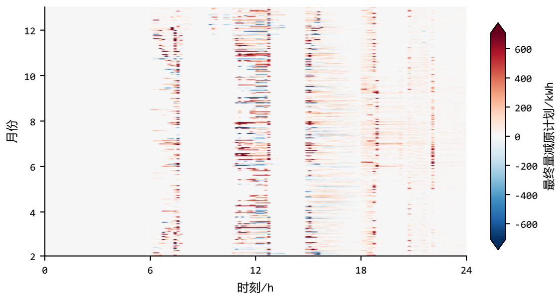
图 7 2 月至 12 月逐槽最终调整量。颜色表示最终常规量减午夜原计划；色轴在绝对调整量 99.5% 分位处截断以显示主要分布，原始值均保留参与费用计算。
