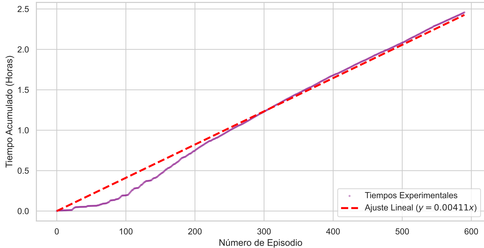
Coste Computacional: Tiempo vs Número de Episodios
