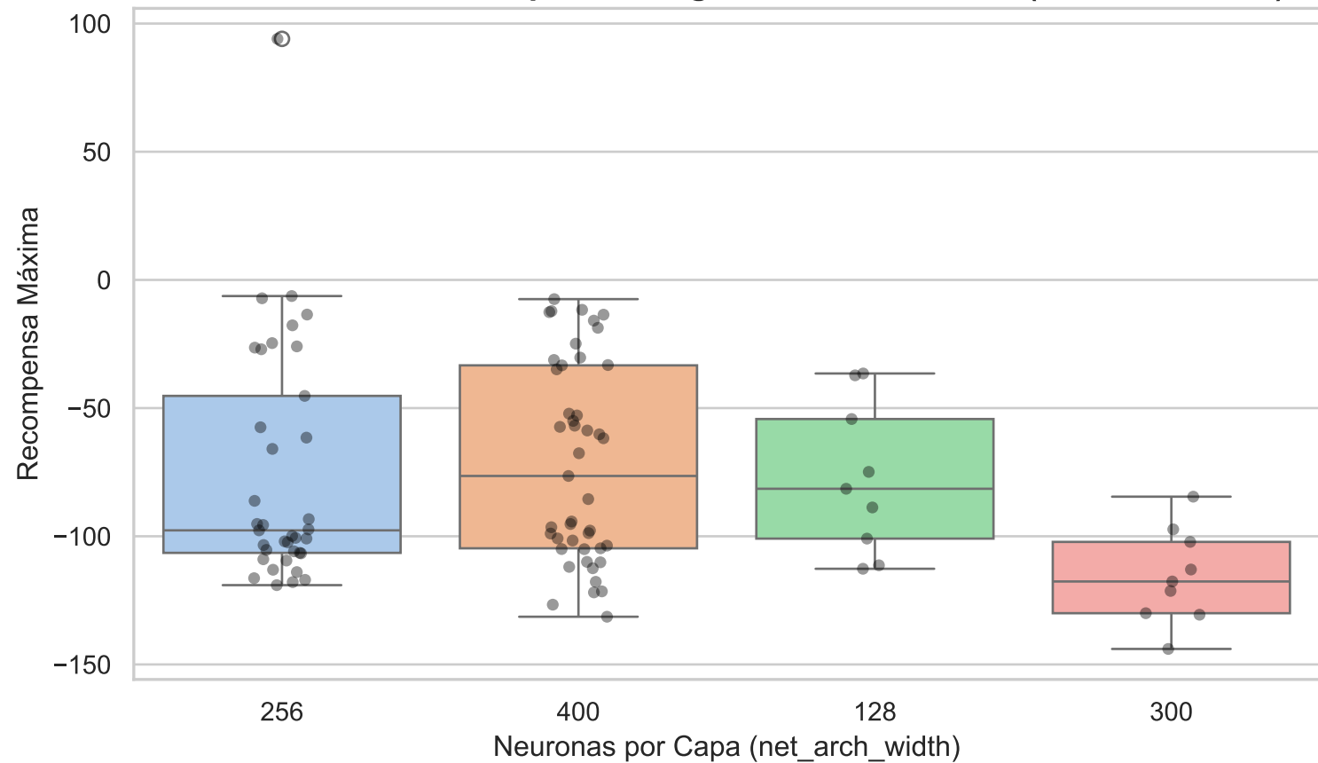
Distribución de Recompensas según Ancho de la Red (Net Arch Width)
