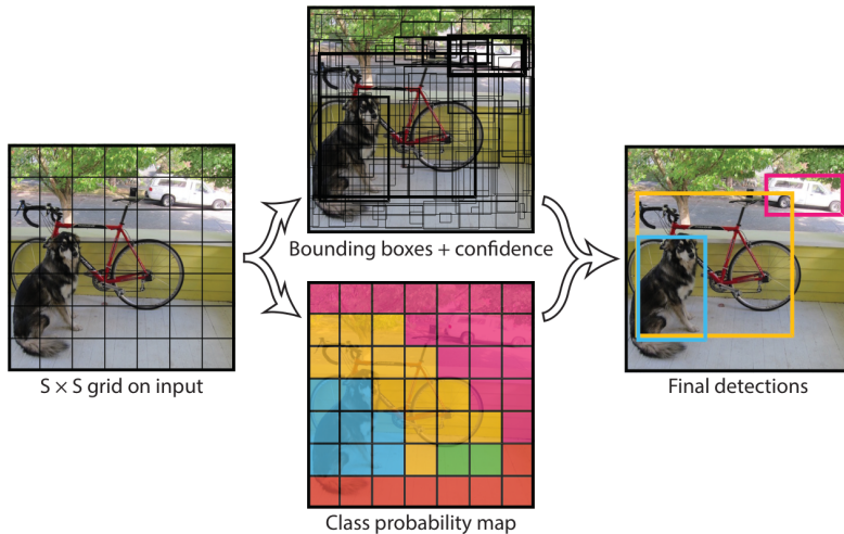
Figura: Esquema de predicción unificada: de la rejilla a la detección final.
