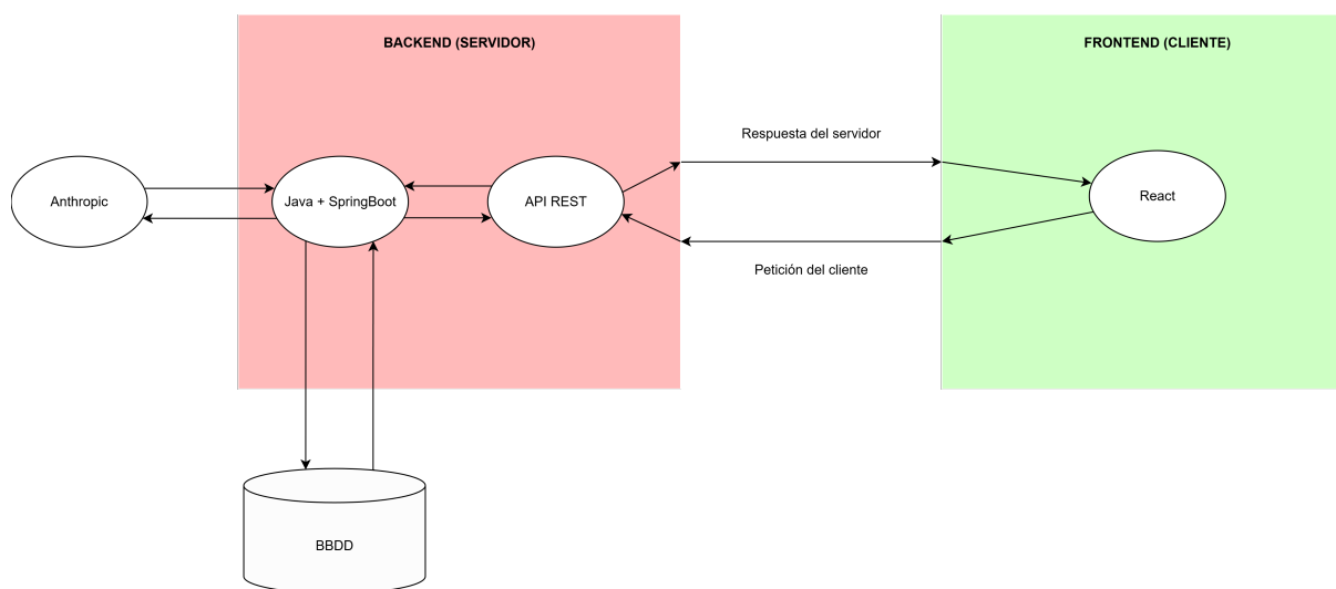
Figura 7.1.: Arquitectura de la solución
