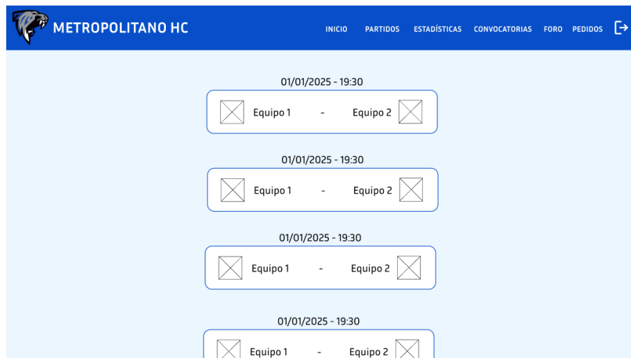
Figura 7.4.: Prototipo de pantalla de partidos
