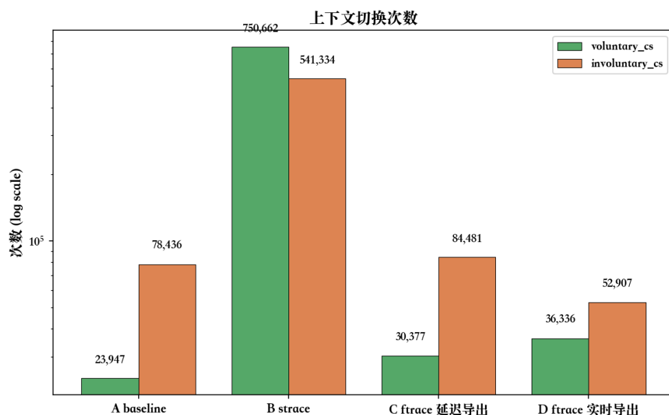
图 3-2 四组的自愿与非自愿上下文切换次数（对数坐标）
