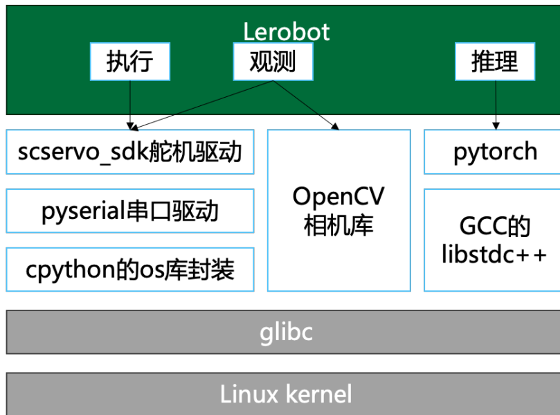
图 2-3 Lerobot 软件栈架构
