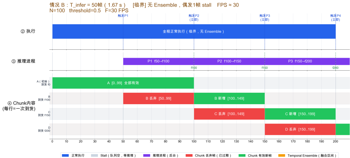
图 4-3 情况 B: T_{\text{infer}} = 50 帧, 恰好处于临界点
