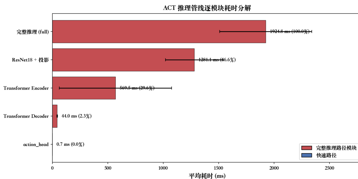
图 3-10 ACT 推理管线逐模块耗时分解
