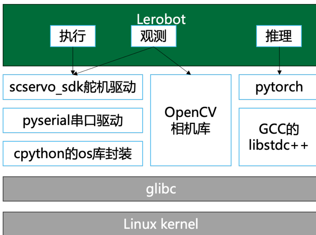
图 2-3 Lerobot 软件栈架构
