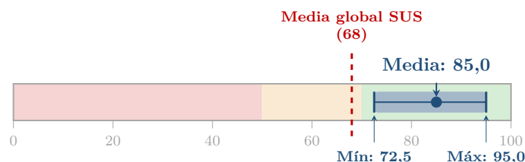
Figura 3: Distribución del intervalo muestral (mínimo, media y máximo) respecto al umbral SUS (68).
