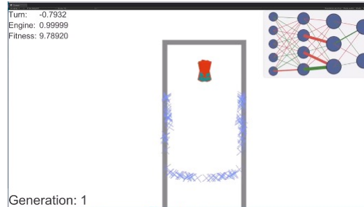
apprentissage automatique
