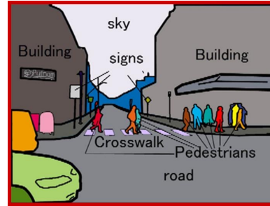
reconnaissance d'objets
