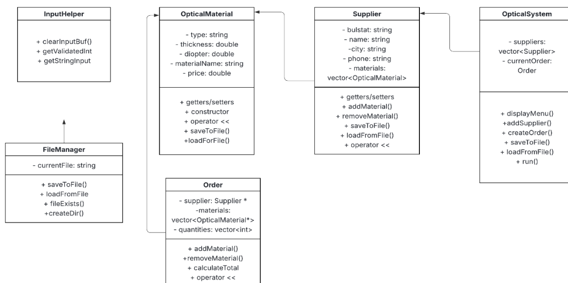
Фиг. 1: UML диаграма
