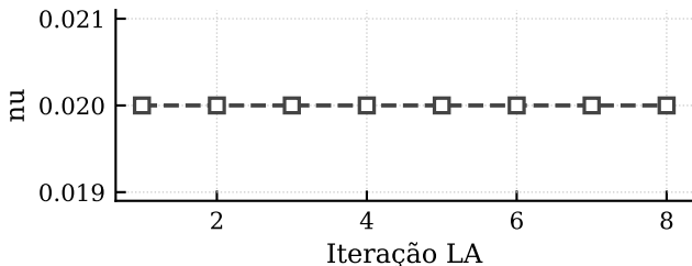
Parâmetro: \nu
