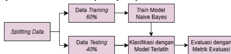
Gambar 3. Alur Pemodelan Naïve Bayes
