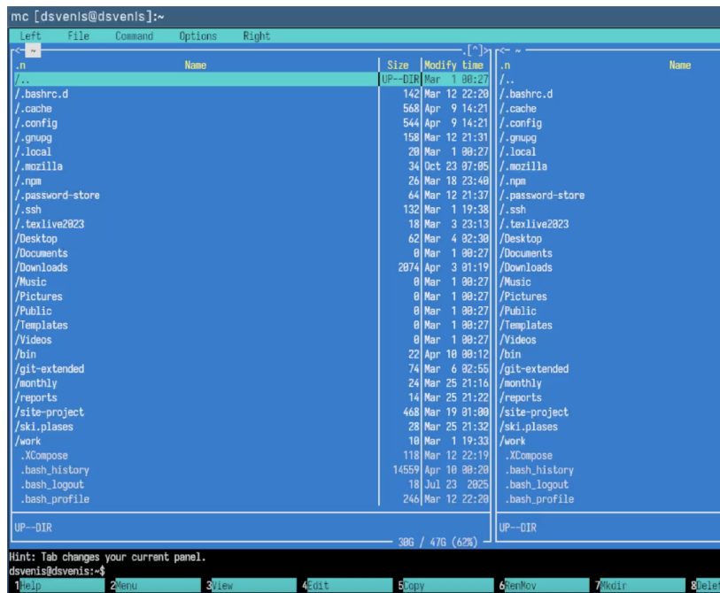
Рисунок 4.2: Интерфейс mc
