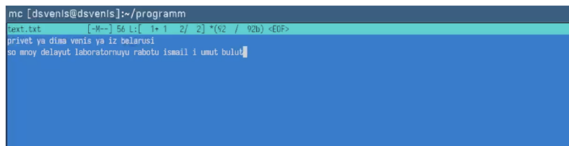
Рисунок 4.3: Редактор mc
