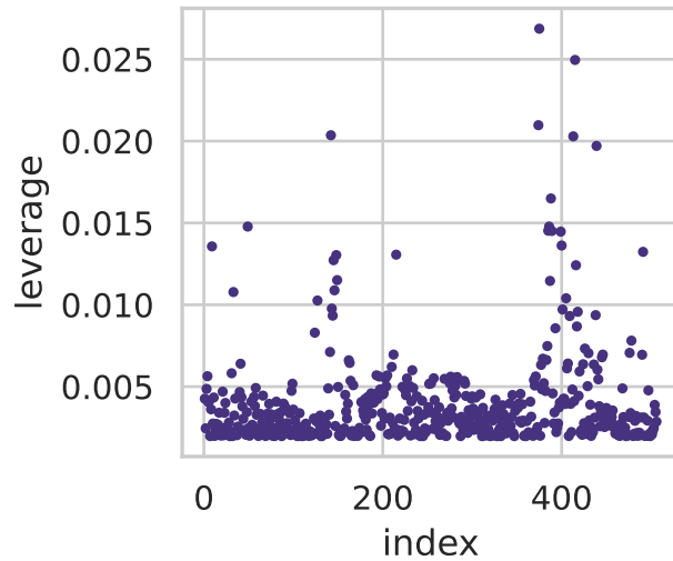
Hat values
