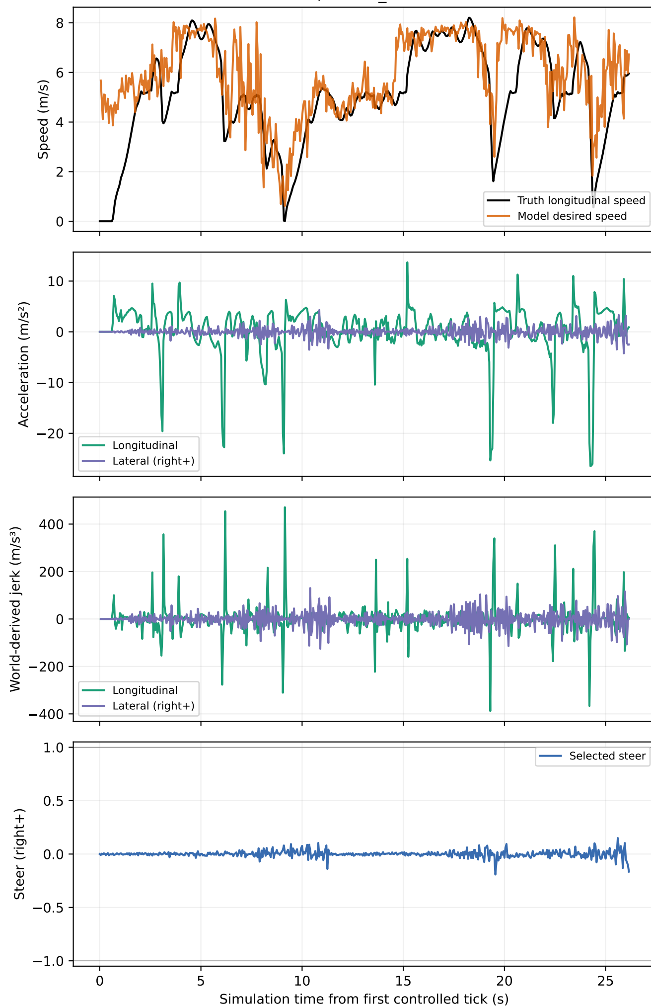
1711 / native_common
